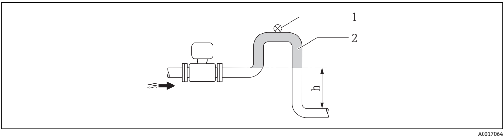
4 在竖直向下管道中安装
