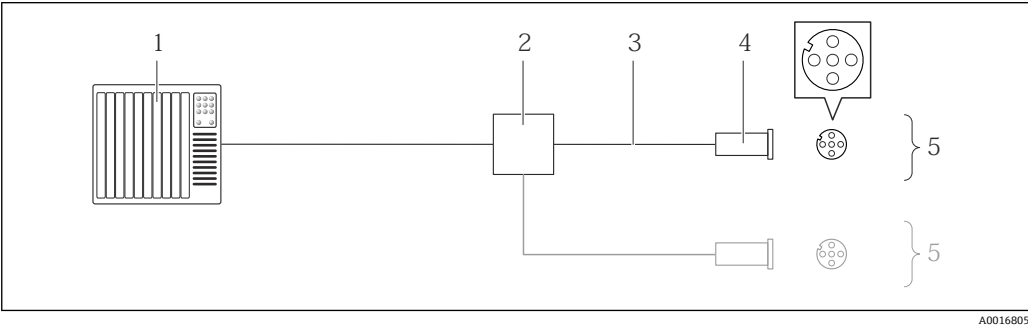
图 7 工业以太网(EtherNet/IP)的连接示例
