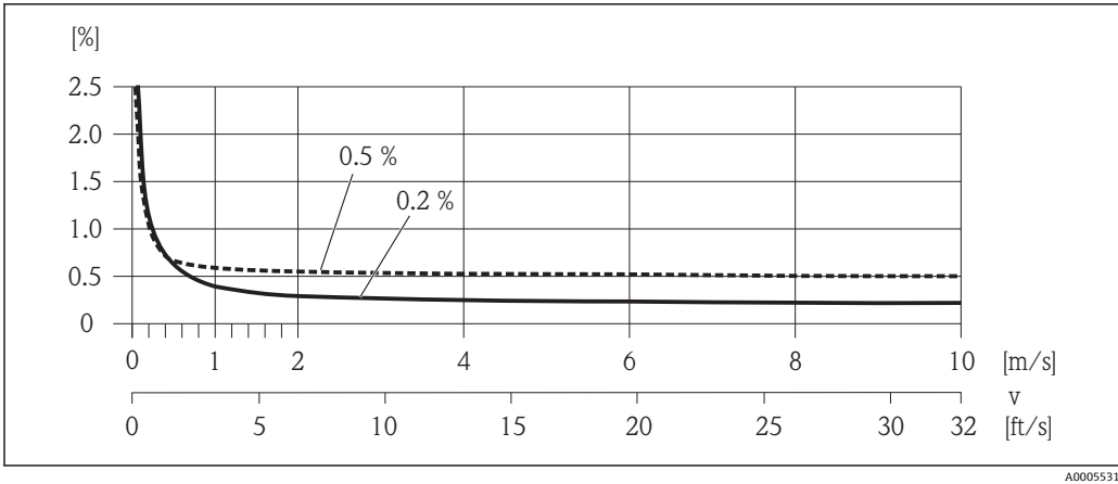
图 11 最大测量误差(% o.r.)示意图
