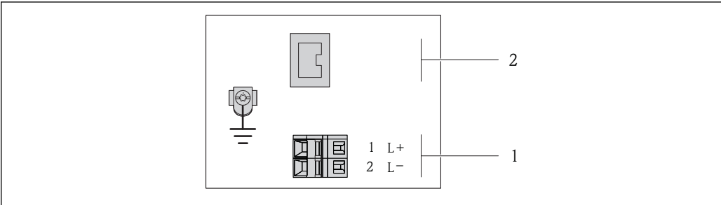
图 6 工业以太网(EtherNet/IP)的接线端子分配示意图
