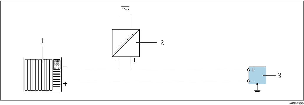
11 接线实例：脉冲输出/频率输出/开关量输出（无源）
