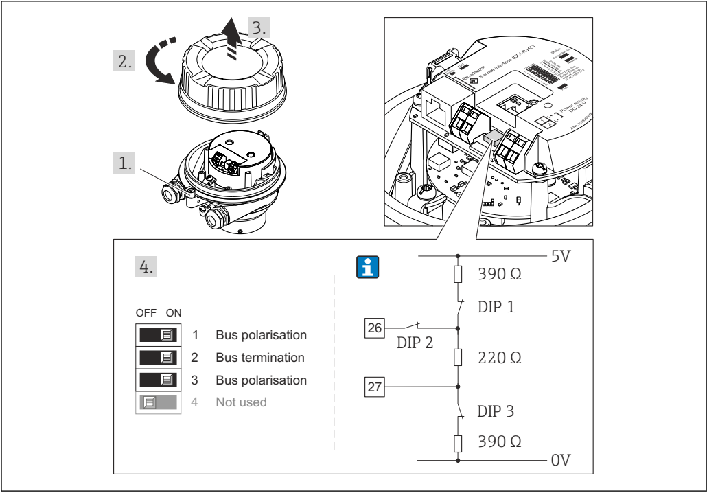
13 使用 I/O 电子模块上的 DIP 开关端接(波特率小于 1.5 MBaud)
