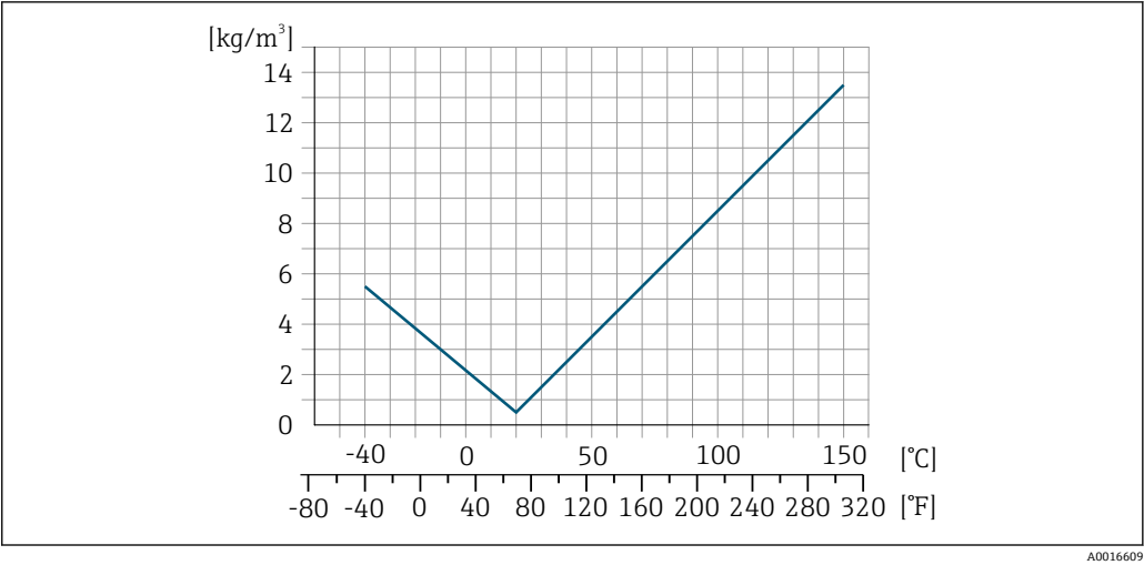
18 现场密度校正，例如在+20 °C (+68 °F)时
