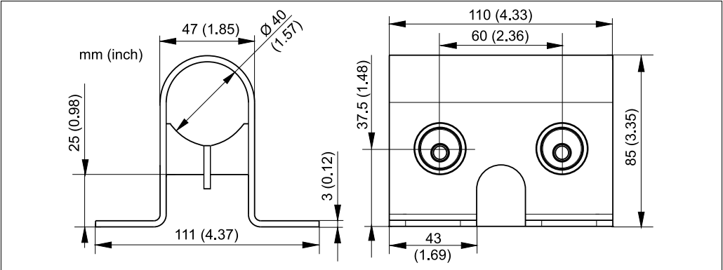
壁式安装件和平面安装基座的外形尺寸示意图
