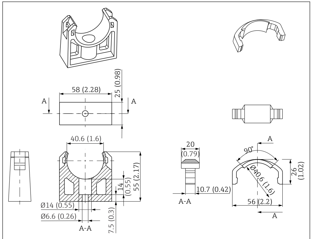
图 21 管箍; 单位: mm (in)
