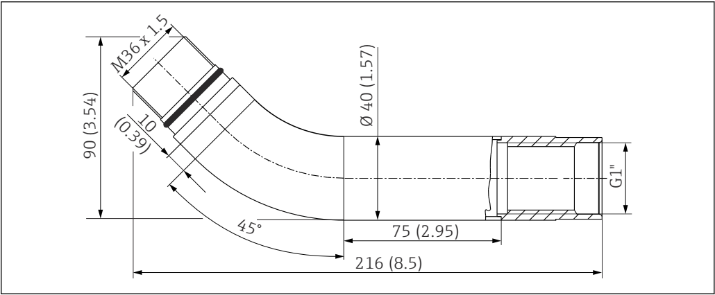
图 30 45°弯连接管; 单位: mm (in)
