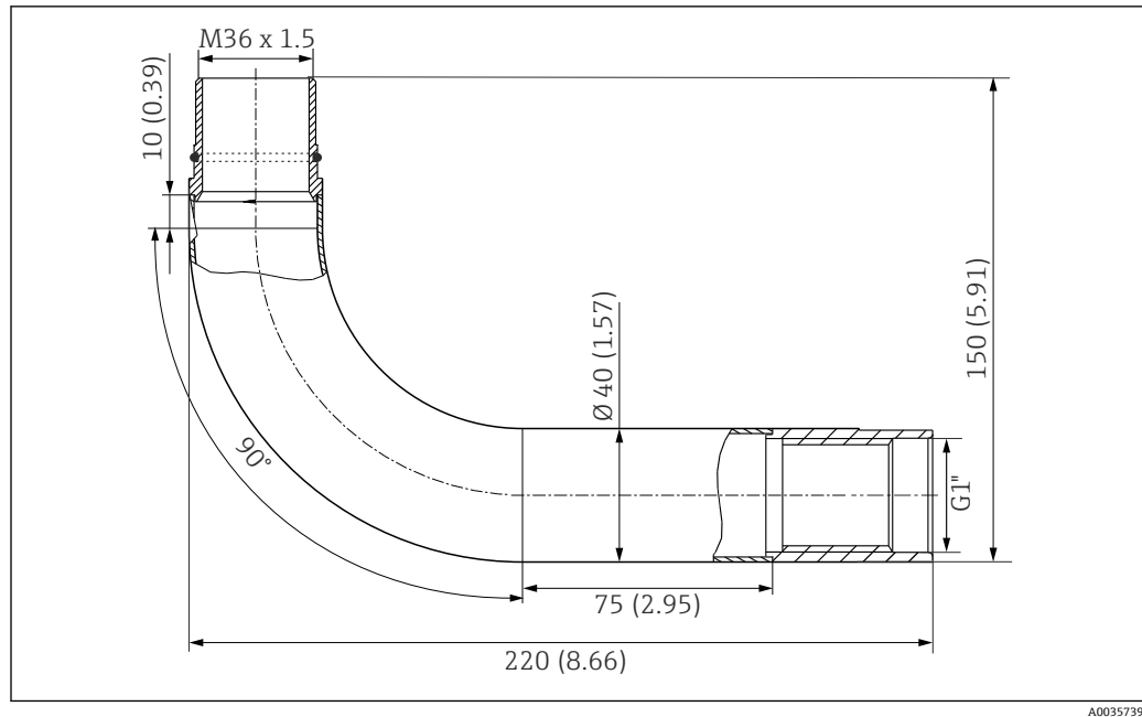
图 31 90°直角连接管；单位：mm (in)
