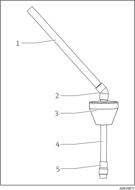
图 6 浮球型安装支架
