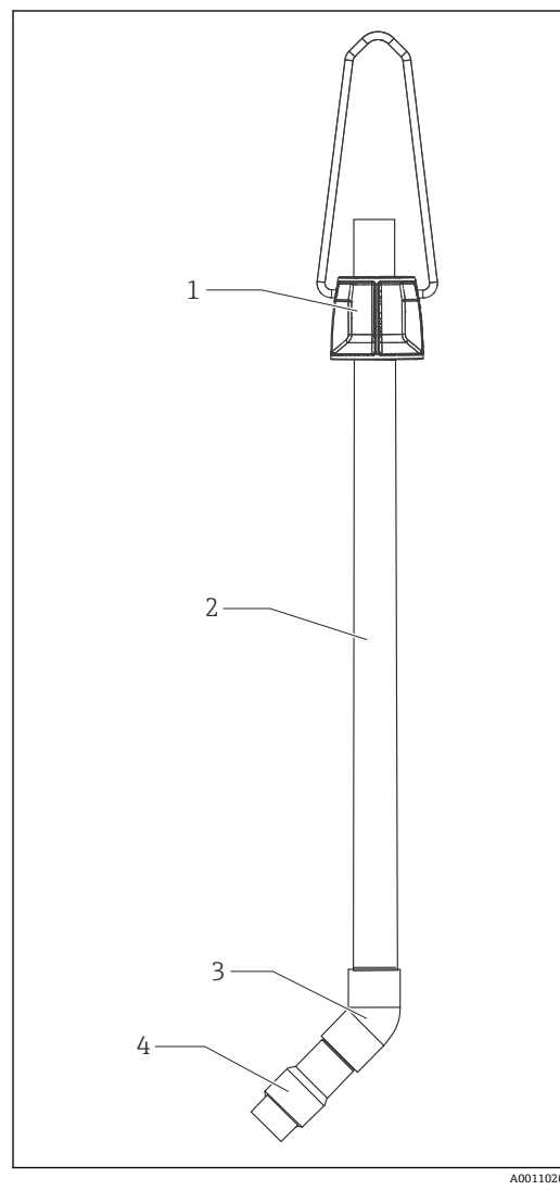
图 13 OKCYA112 安装支架，带弯连接管和链条卡扣
