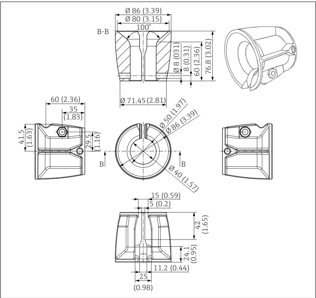
图 19 多功能卡扣; 单位: mm (in)
