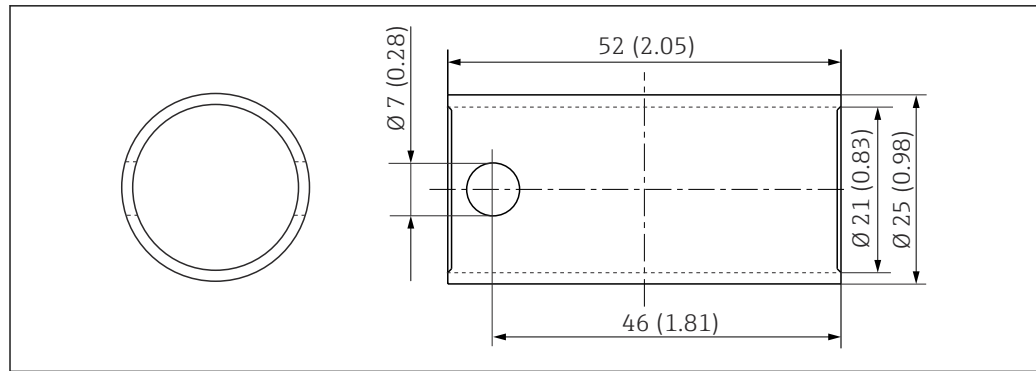
■ 23 安装工具；单位：mm (in)
