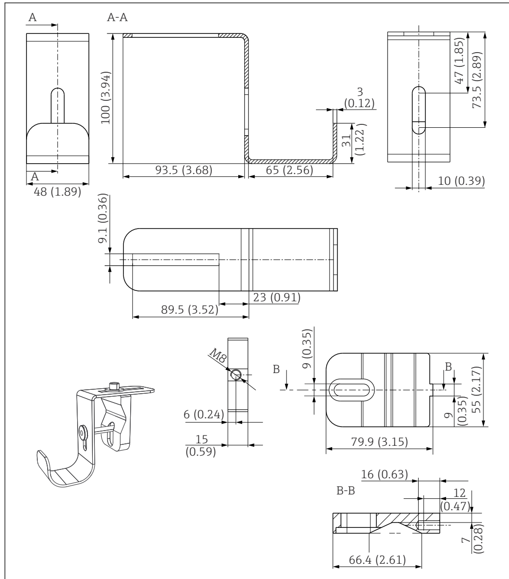
图 20 浸入管托架; 单位: mm (in)
