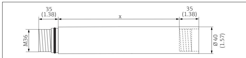
图 28 浸入管; 单位: mm (in)
