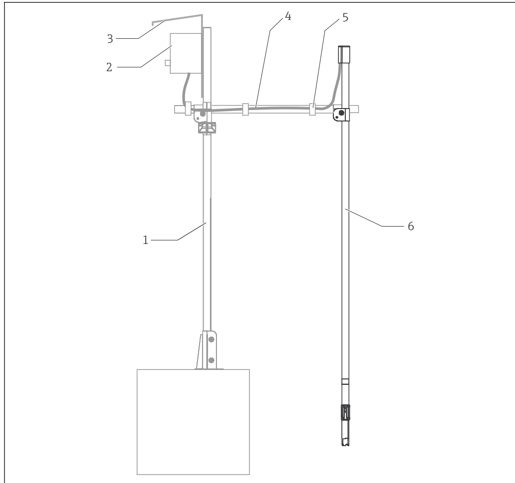
图 1 使用 CYA112 安装支架的测量系统
