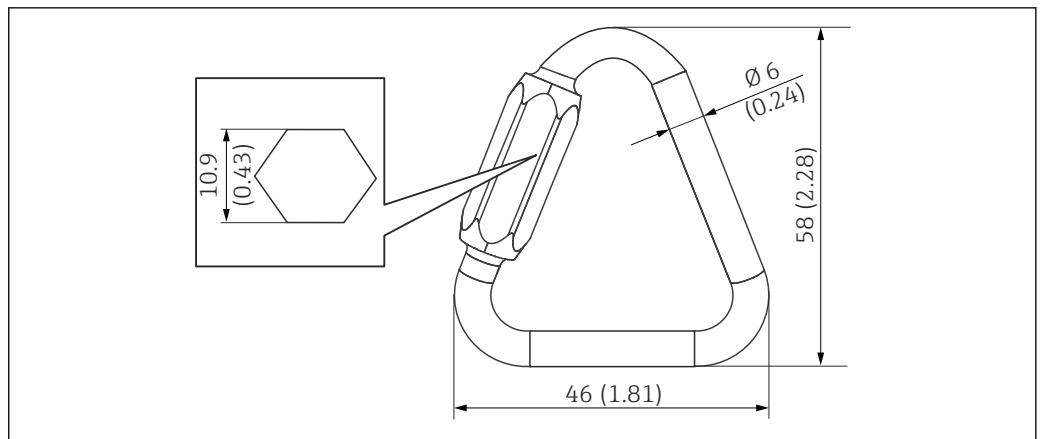
图 22 三角锁扣; 单位: mm (in)
