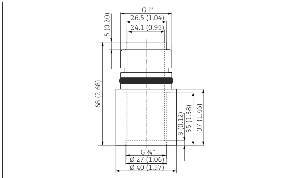
26 G 1" - G 3/4"传感器转接头; 单位: mm (in)
