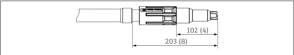
18 安装就位的快速紧固件和 Pg 13.5 传感器接头的外形尺寸；单位：mm (in)
