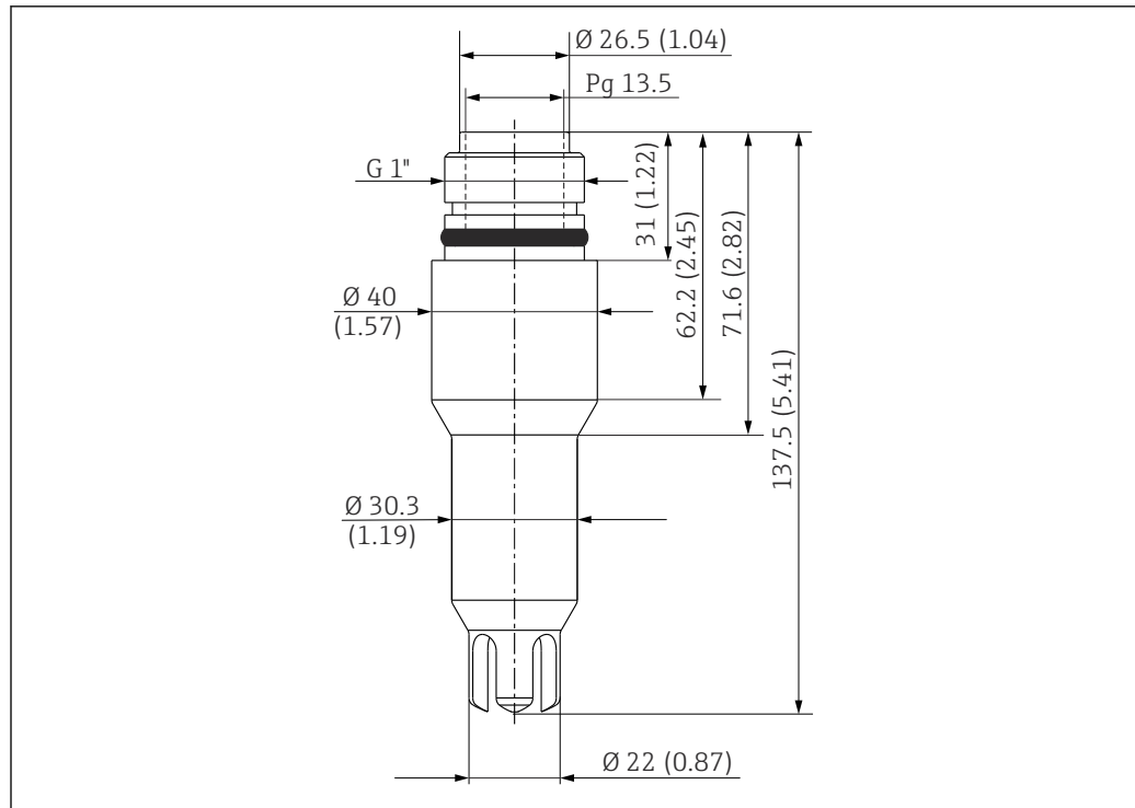
图 27 G 1" - Pg 13.5"传感器转接头; 单位: mm (in)
