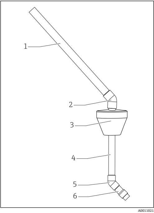
11 CYA112 安装支架，带浮球
