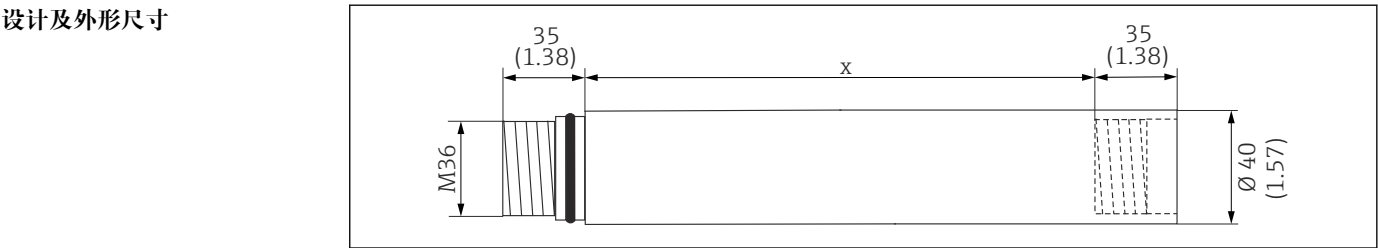
17 不锈钢浸入管 x 自由调节长度
