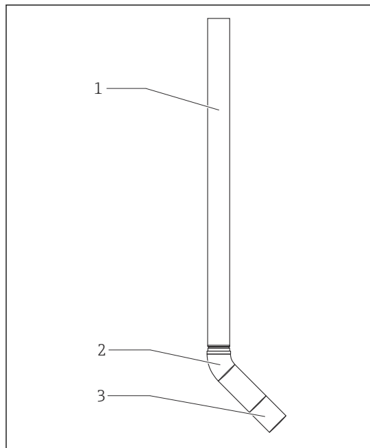
图 9 CYA112 安装支架，带弯连接管，G 1"传感器接头
