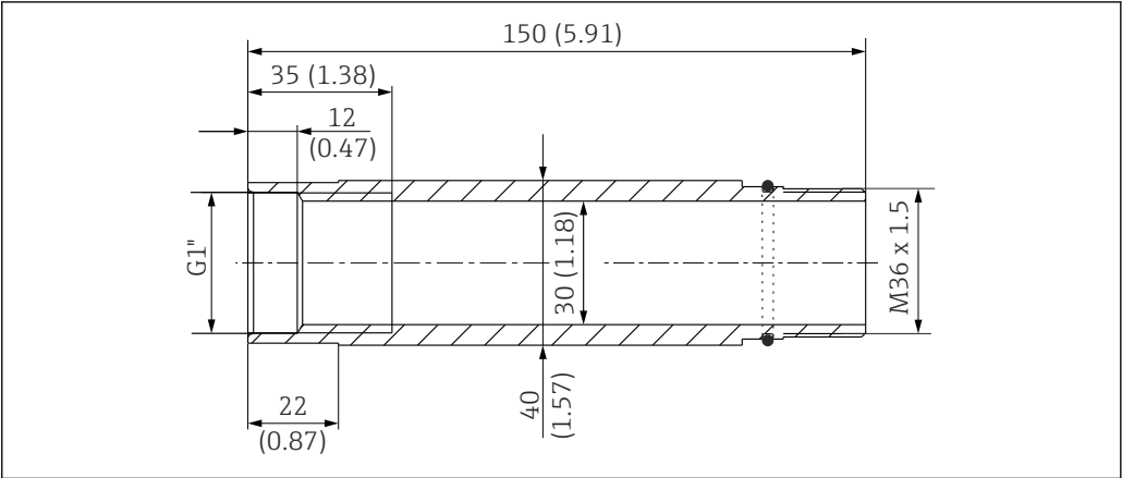
图 29 直连接管; 单位: mm (in)
