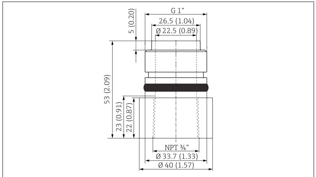
25 G 1" - NPT 3/4"传感器转接头; 单位: mm (in)
