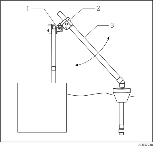
图 7 浮球型安装支架，安装在悬摆底座上
