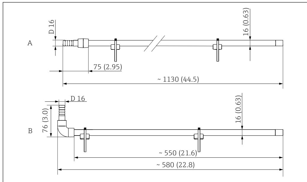
图 32 CYA112 专用喷洒清洗单元；单位：mm (in)
