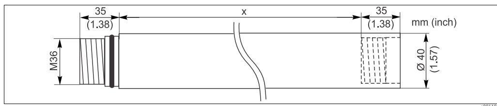
浸入管示意图
