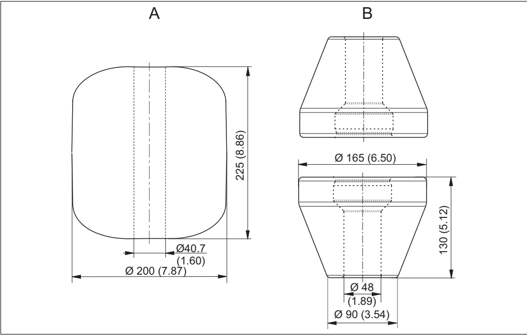
浮球示意图
