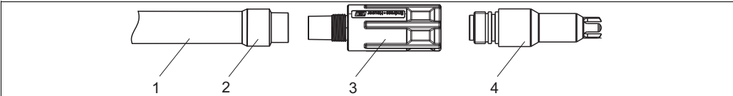
快速紧固件示意图
