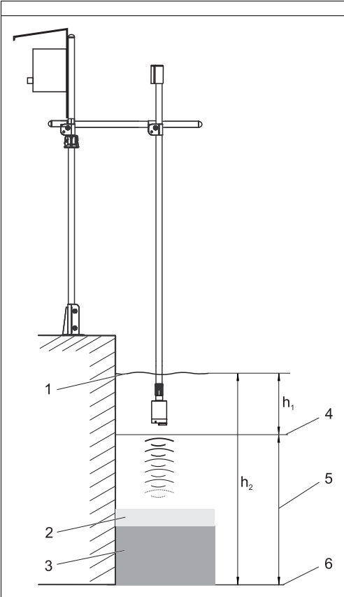
图 10: 罐底盲区
