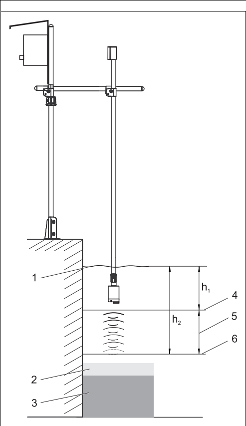
图 11: 罐体上方的盲区
