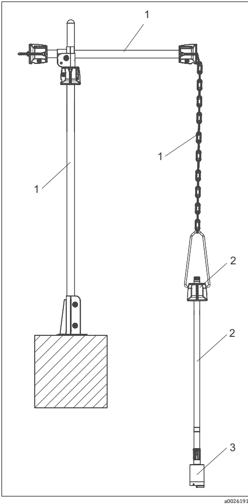
图 5: 测量系统示意图，带链条式安装支座
