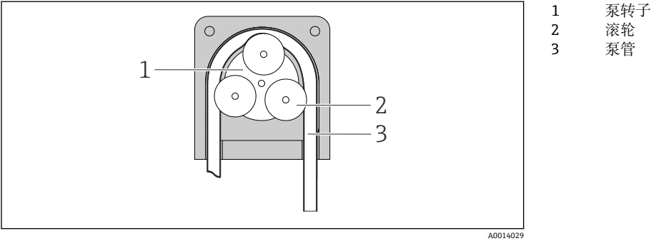
图 28 蠕动泵内视图
