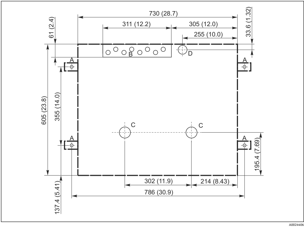
5 底座平面图。测量单位 mm (in)
