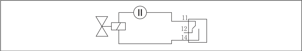
图 15 带继电器的数字量输出的连接实例
