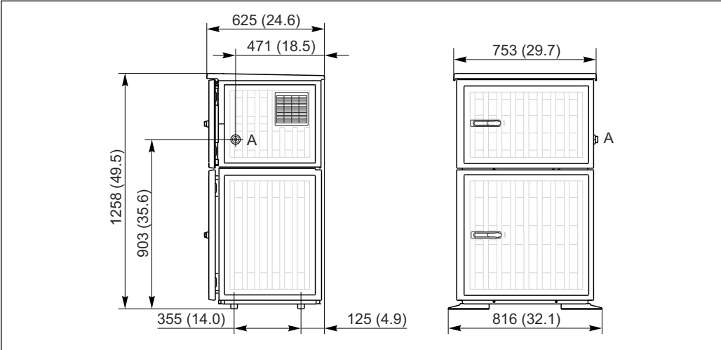
3 Liquistation 的外形尺寸示意图；塑料外壳。测量单位 mm (in) A 吸液管道接口
