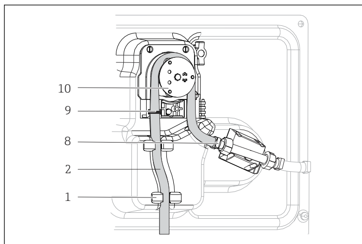
图 25 更换泵管
