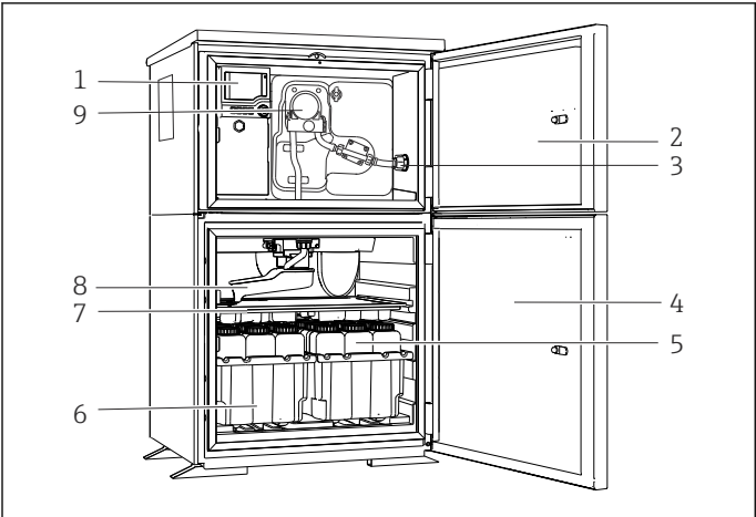
图 2 Liquistation 采样仪（带蠕动泵的仪表型号）的结构示意图
