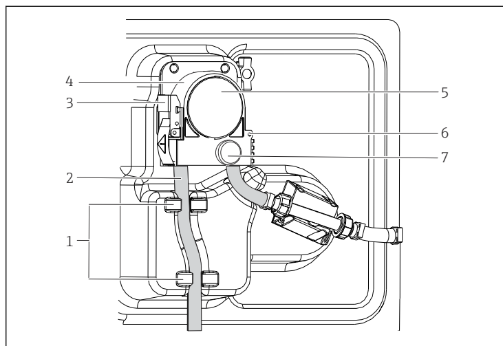
图 24 打开蠕动泵
