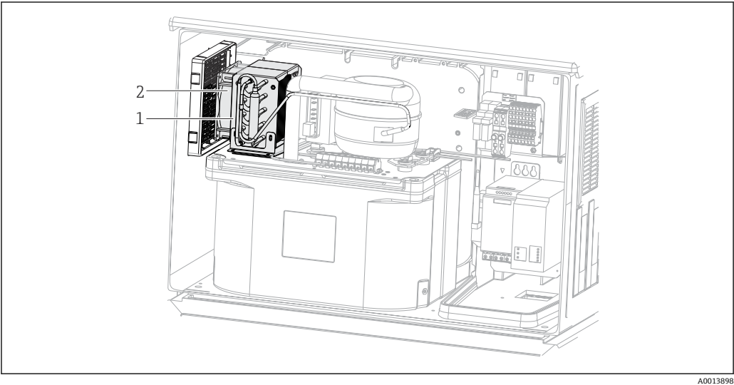
图 29 清洗温度控制模块
