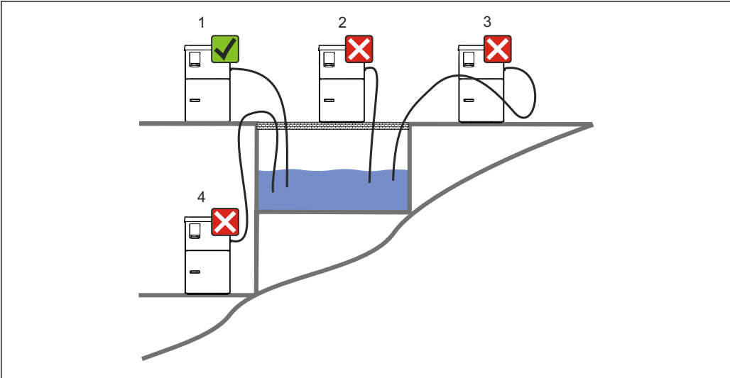
4 Liquistation 的安装位置
