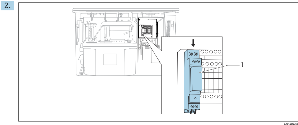
16 数字量输出接线
