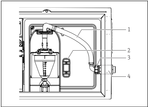
图 7 侧面连接吸液管道（出厂状态）
