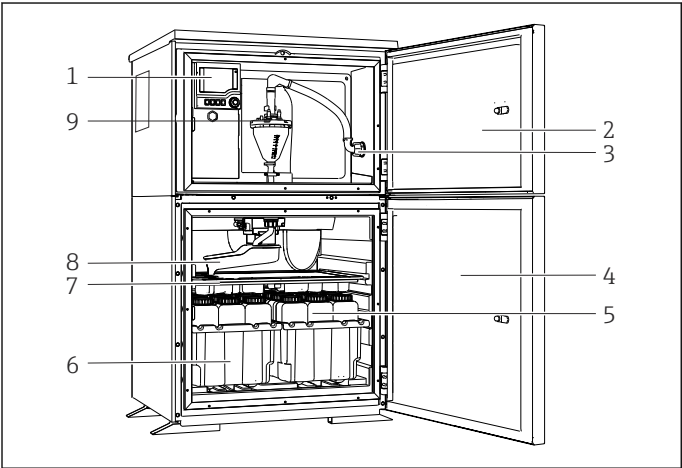
图 1 Liquistation 采样仪（带真空泵的仪表型号）的结构示意图
