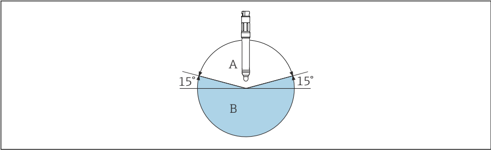
图 1 水平方向上的倾斜安装角范围，不得小于 15^\circ
