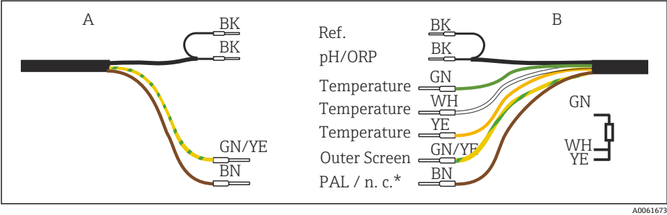
5 整体电缆
