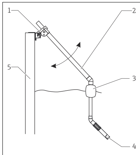
图 8 池边安装
