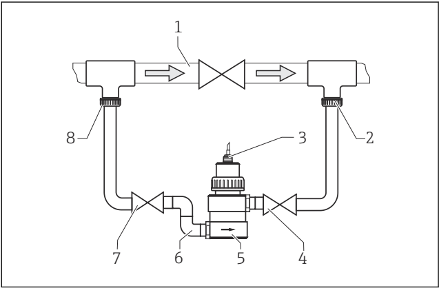
11 手动动作阀或电磁阀的旁路安装
