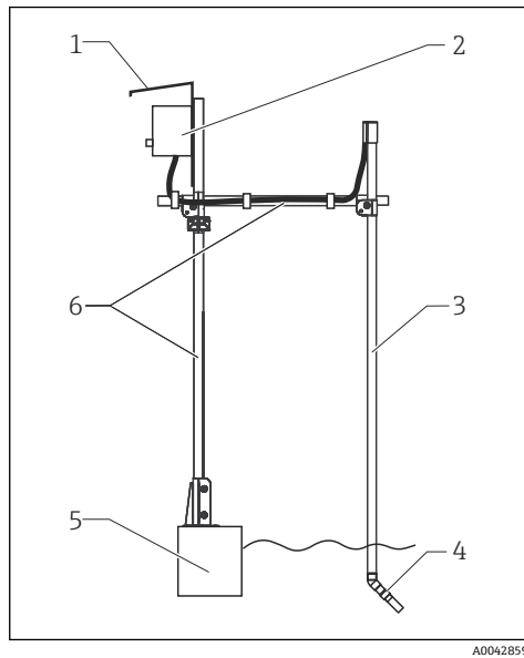
图 7 带浸入管的浸入式支座
