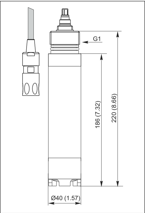
图 15 带 TOP68 插头的型号
