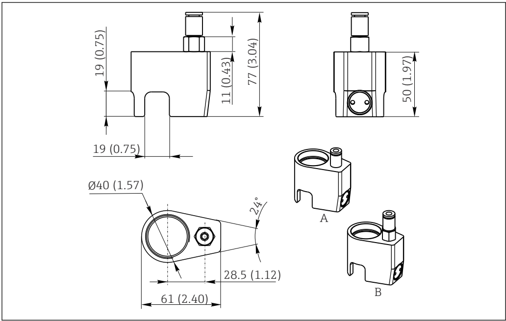
图 16 单位: mm (inch) A 压缩空气清洗单元 (适用 COS61/61D) , 接口直径 6/8 mm (详细信息参见→ 图 14) B 压缩空气清洗单元 (适用 COS61/61D) , 接口直径 6.35 mm (¼") (详细信息参见→ 图 14)
