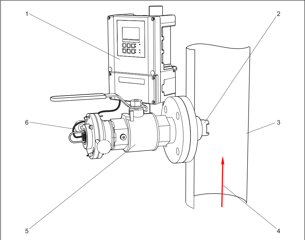
2 安装有 COS61 传感器的测量系统示意图
