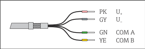
图 3 传感器整体电缆，电缆线芯完成预端接
