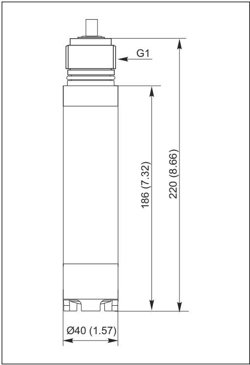
图 14 带整体电缆的型号 单位: mm (inch)
