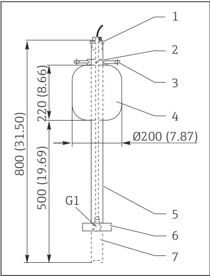
9 单位: mm (inch)
