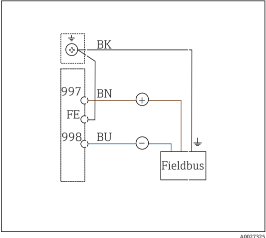
图 21 接线图
