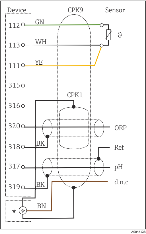
图 40 接线图
