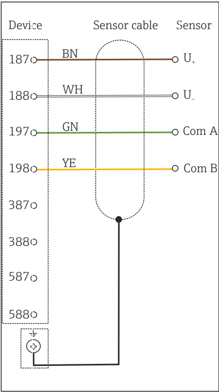
23 接线图
