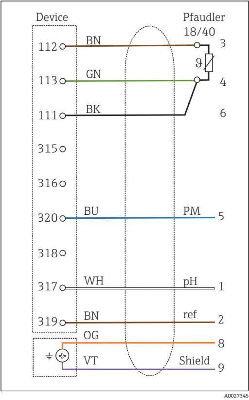
35 接线图
