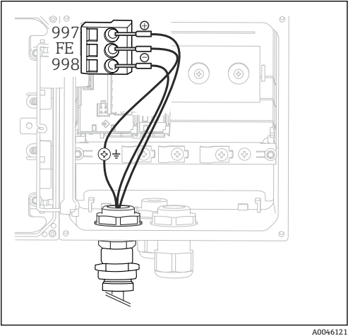
图 20 变送器的内部结构示意图 (CPU 模块)
