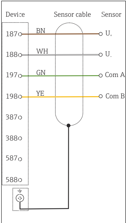
图 25 接线图
