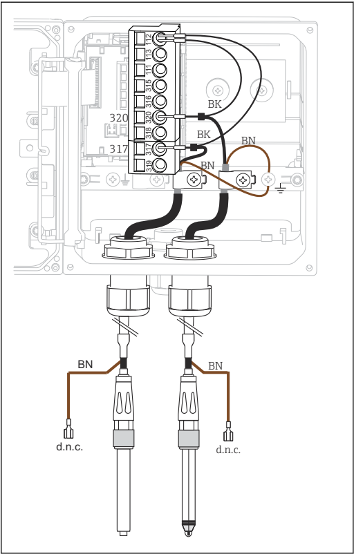
38 变送器的内部结构示意图 (传感器模块)
