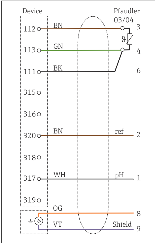
37 接线图
