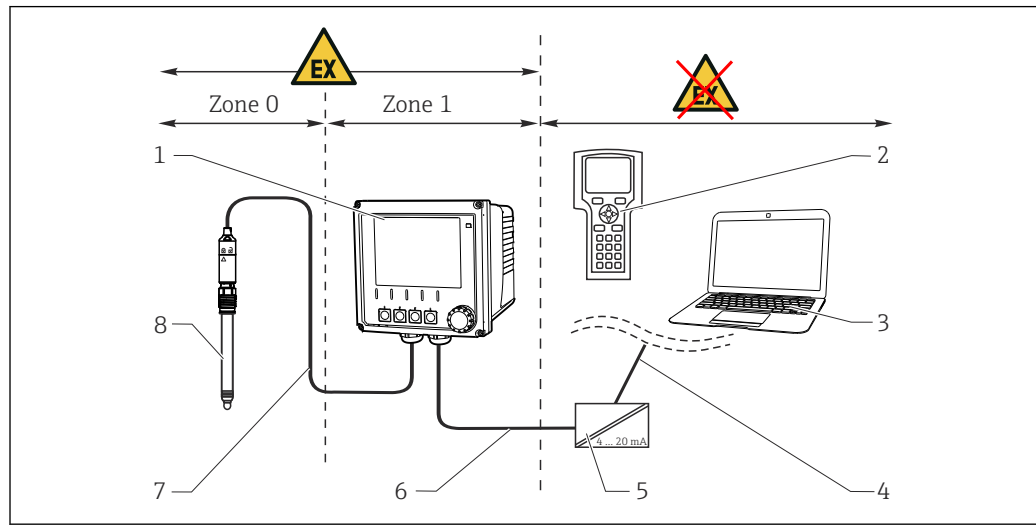
51 在 Ex ib (ia Ga) 防爆区中安装
