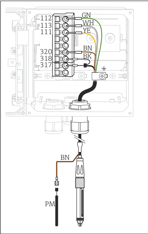
图 26 变送器的内部结构示意图 (传感器模块)
