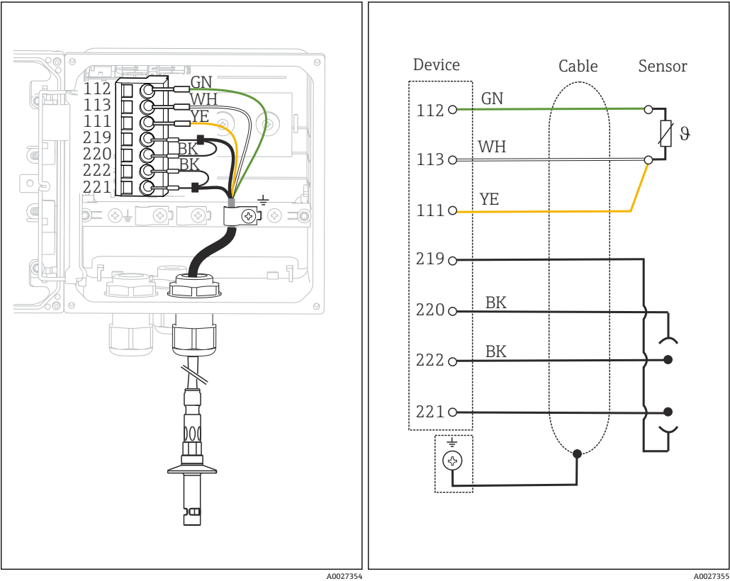
43 变送器的内部结构示意图（传感器模块）
