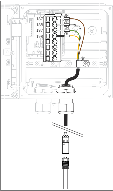
22 变送器的内部结构示意图 (传感器模块)
