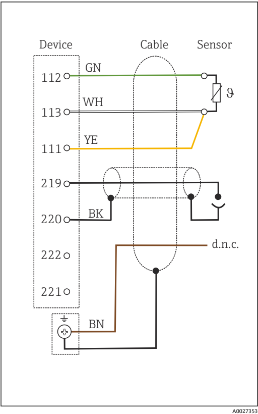
图 42 接线图
