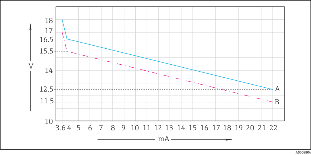
图 9 变送器的最小供电电压，取决于输出电流
