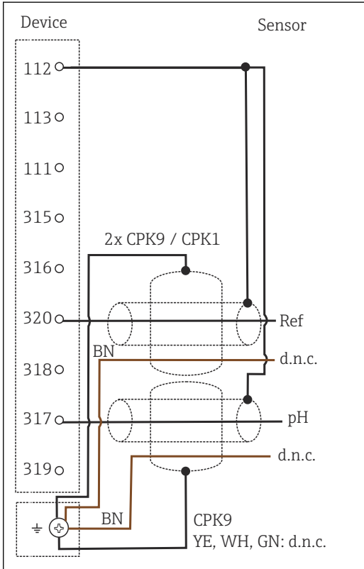
39 接线图
