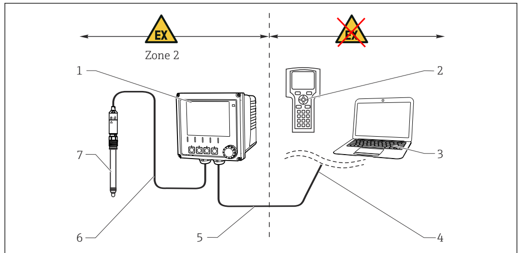
53 在 Ex nA (ic) 防爆区中安装
