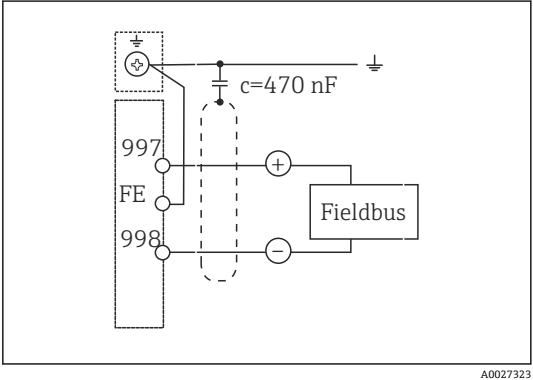
图 19 接线图
