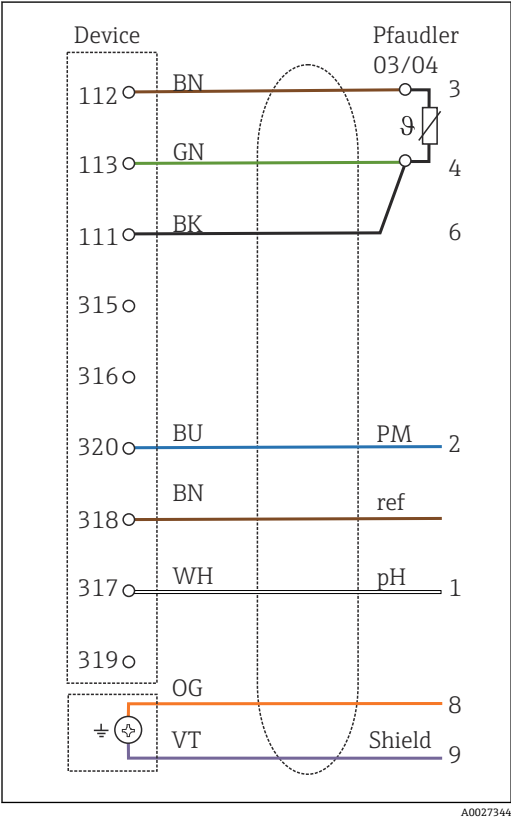
34 接线图
