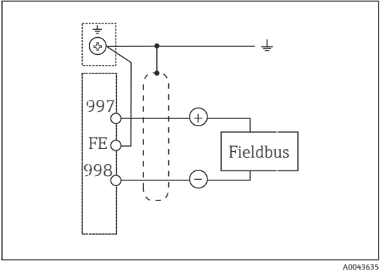
图 17 接线图
