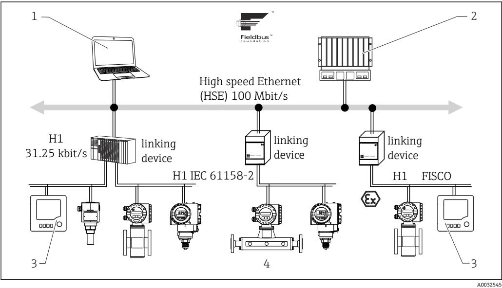
图 66 系统架构及组件
