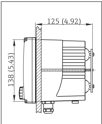
58 盘装
