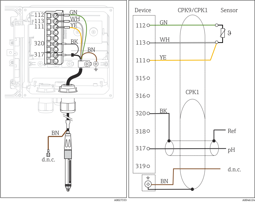
图 28 变送器的内部结构示意图（传感器模块）
