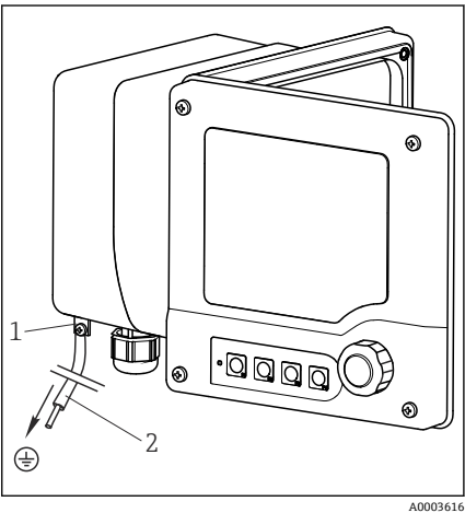
图 11 外壳接地
