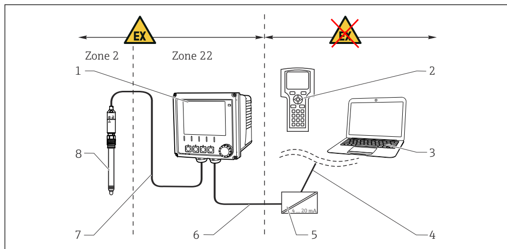
52 在 Ex tc (ic) 防爆区中安装
