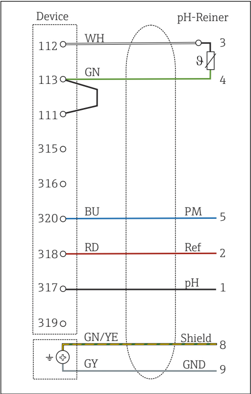
36 接线图
