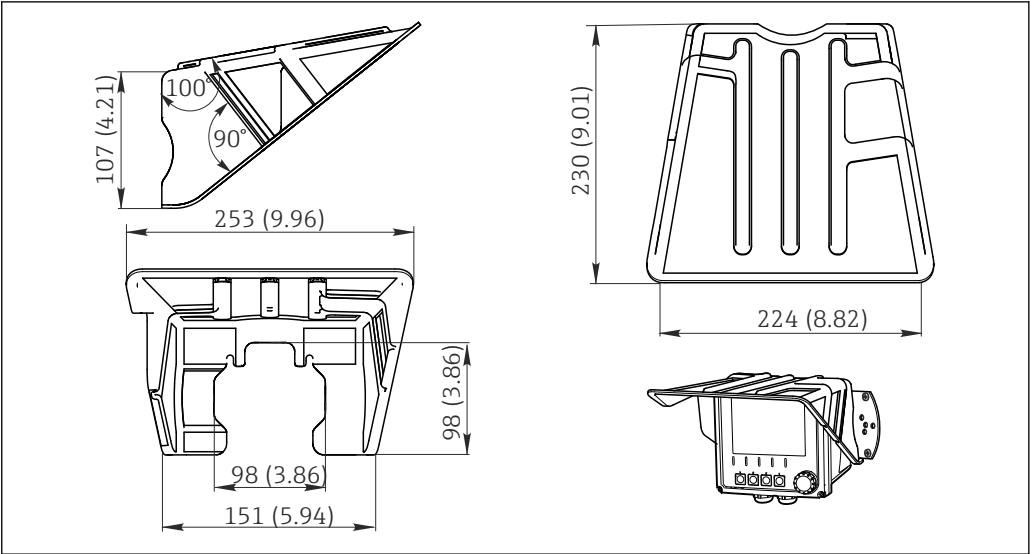
49 单位: mm (inch)
