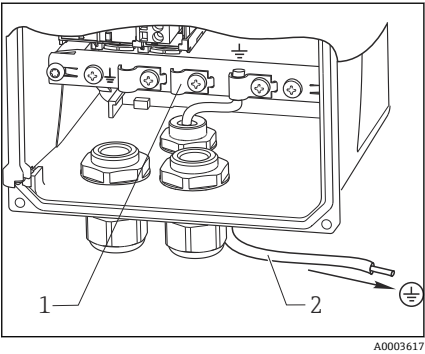
图 10 外壳接地
