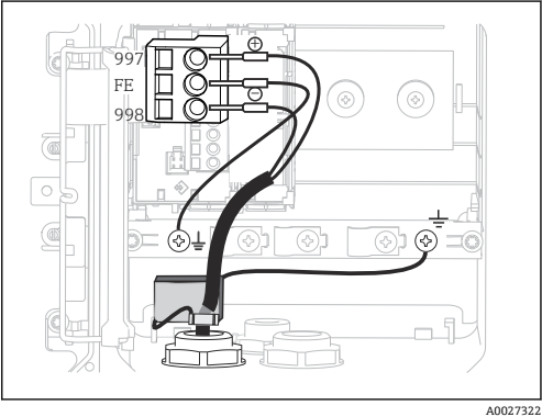
图 18 变送器的内部结构示意图 (CPU 模块)
