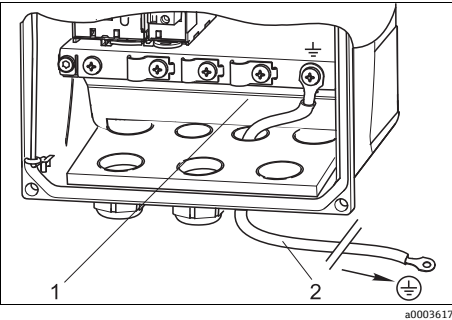
外壳接地
