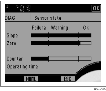
传感器监控功能的图形化显示
