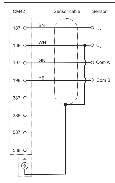
CLS50D 和 CLS54D 电气连接示意图
