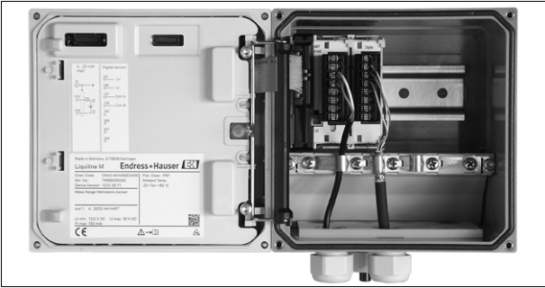
Liquiline 变送器的内部结构示意图 ( 安装有传感器模块, 未接线 )
