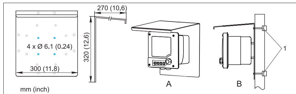
防护罩 CYY101 示意图
