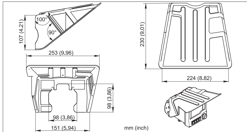
防护罩示意图
