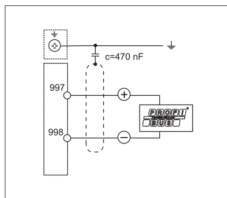
电气连接示意图
