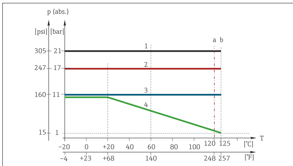
12 温压曲线
