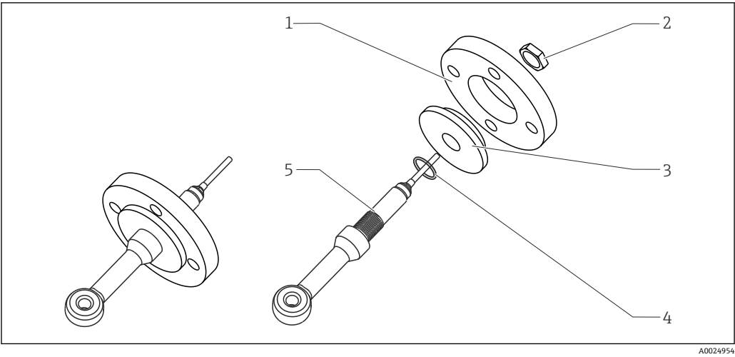
图 9 不接液松套法兰的安装示意图(订购选项“过程连接”，选型代号 A、B、C)
