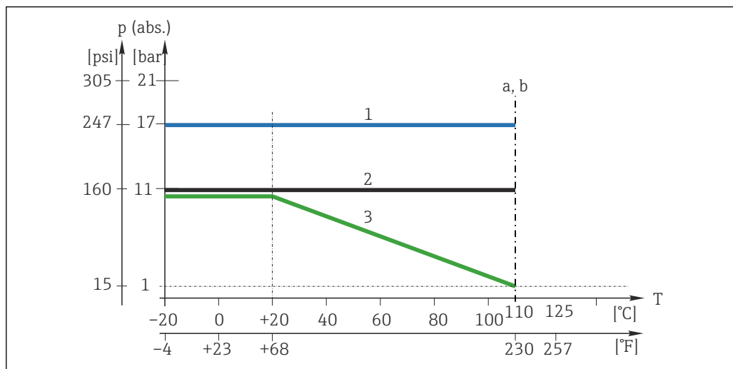
13 温压曲线
