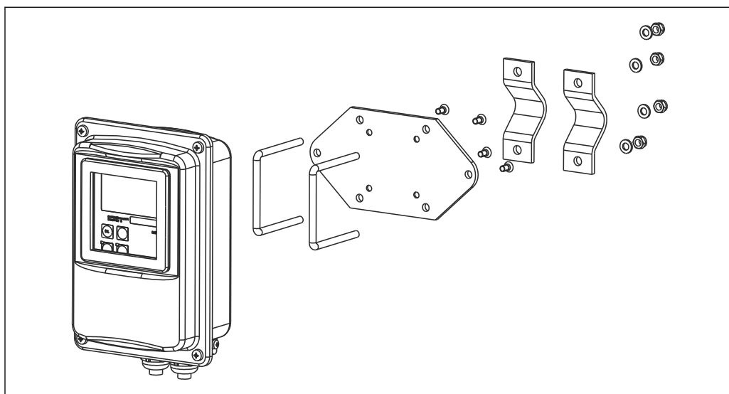
图 14 CLD134 分体式安装的柱式安装套件
