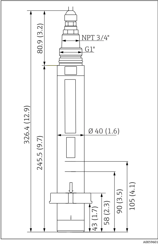
图 3 传感器（带卡环）的外形尺寸；单位：mm (in)
