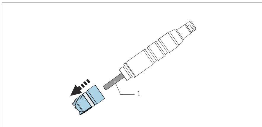
15 小心拆除覆膜帽。
