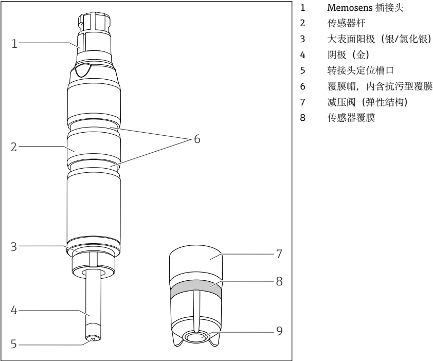
1 传感器结构
