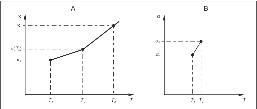
24 温度系数的定义曲线
