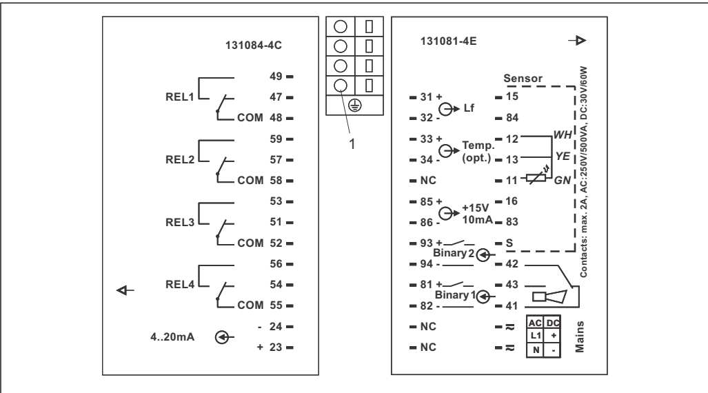
11 盘装型变送器的接线粘贴标签示意图 1 接地端
