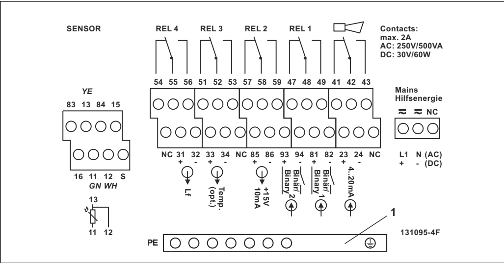
10 现场型变送器接线腔内的粘贴标签示意图 1 CD/CS 型变送器的等电势端(PE) (连接电导式传感器)
