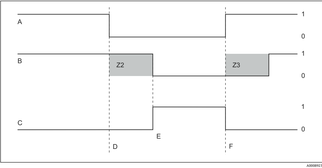
图 25 主流量报警信号的触发与试剂添加过程关闭示意图
