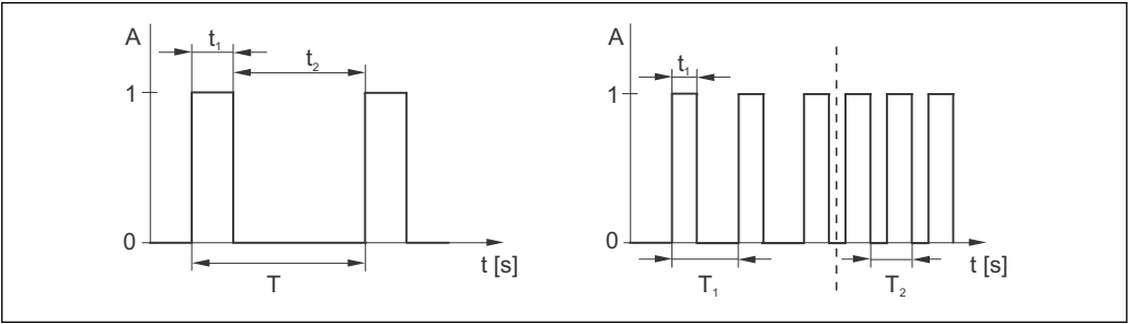
图 32 左图：脉冲宽度调制控制器触点信号；右图：脉冲频率调制控制器触信号
