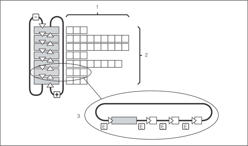
图 23 菜单结构示意图 1 功能选项(参数选择、数值输入) 2 功能组，通过 PLUS 键和 MINUS 键前后滚动选择 3 通过 ENTER 键进行功能切换
