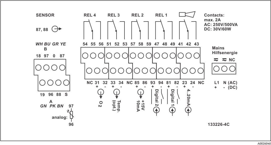
图 15 WX/WS 型 Liquisys M 现场型变送器接线腔的粘贴标签示意图
