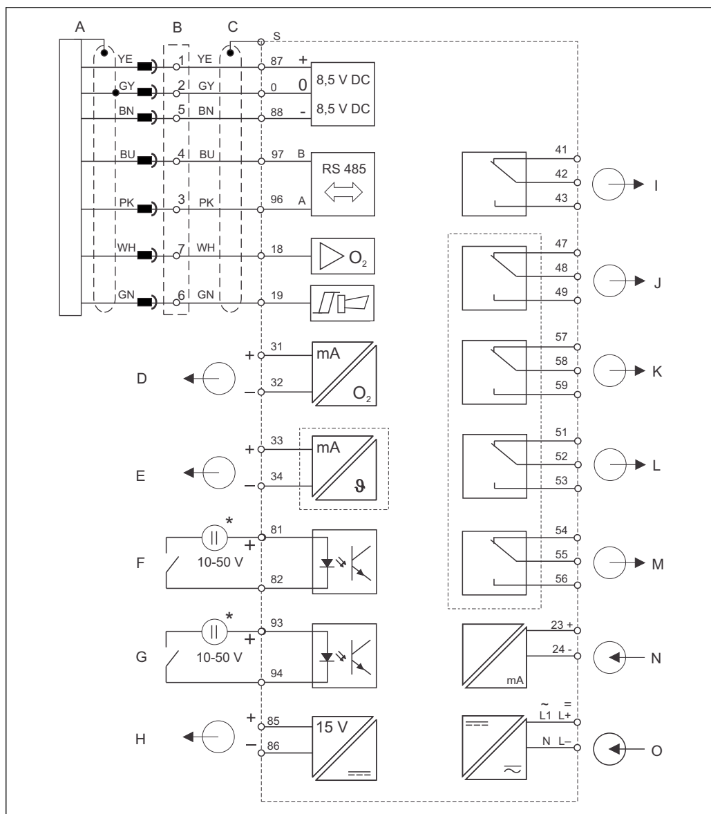
图 14 WX 或 WS 型 Liquisys M COM223/253 变送器的电气连接示意图
