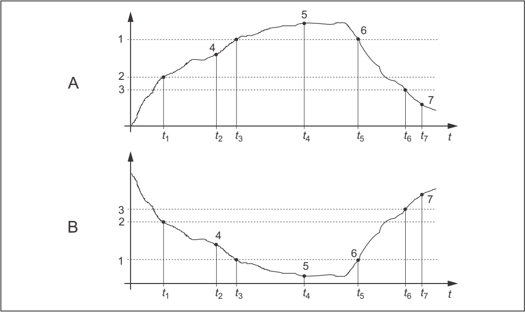
30 报警和限定值功能的图示说明
