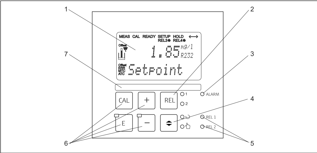
21 操作单元示意图
