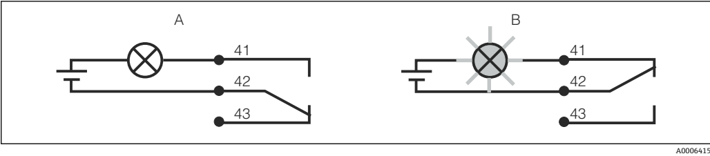
图 19 报警继电器触点的推荐故障安全切换
