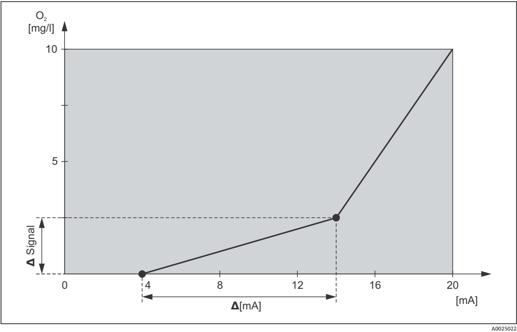
图 29 用户自定义电流输出特征参数示例
