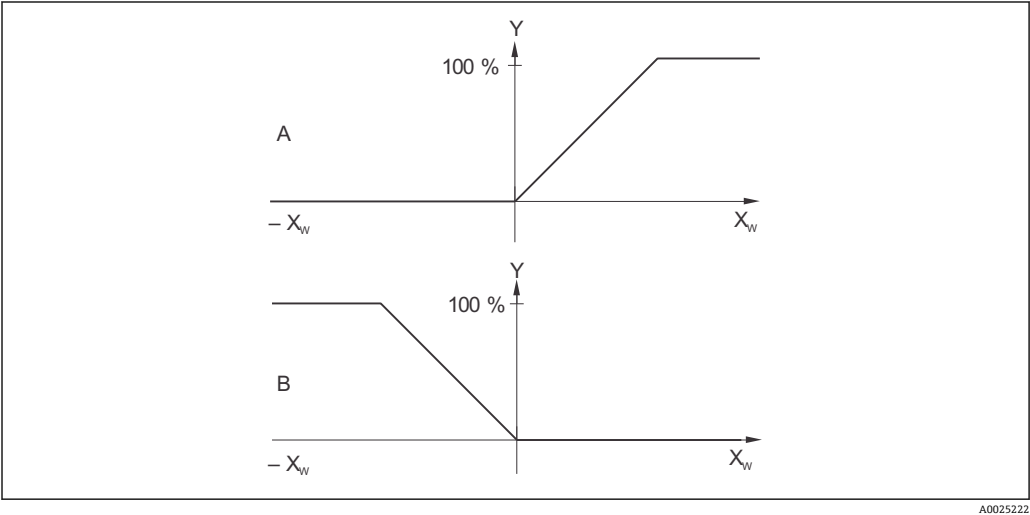
图 34 比例控制器的正向控制响应和反向控制响应的控制性能示意图
