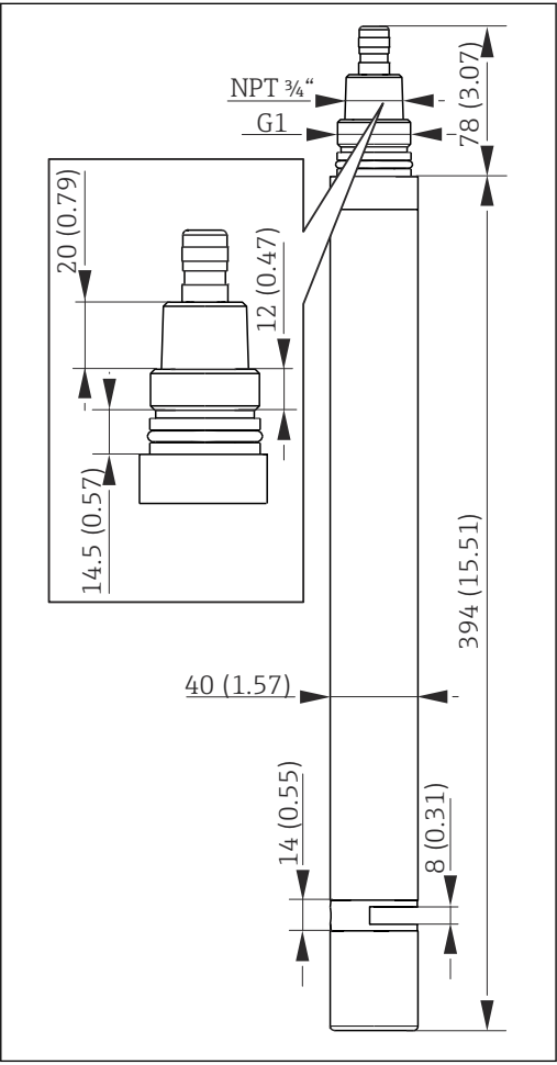
图 10 8 mm (0.31 in)光程的传感器的外形尺寸示意图; 单位: mm (in)
