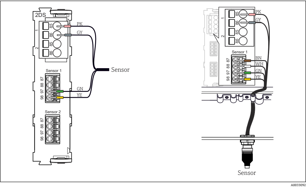
图 3 传感器直接连接输入接线端（左图），或通过 M12 插头连接（右图）
