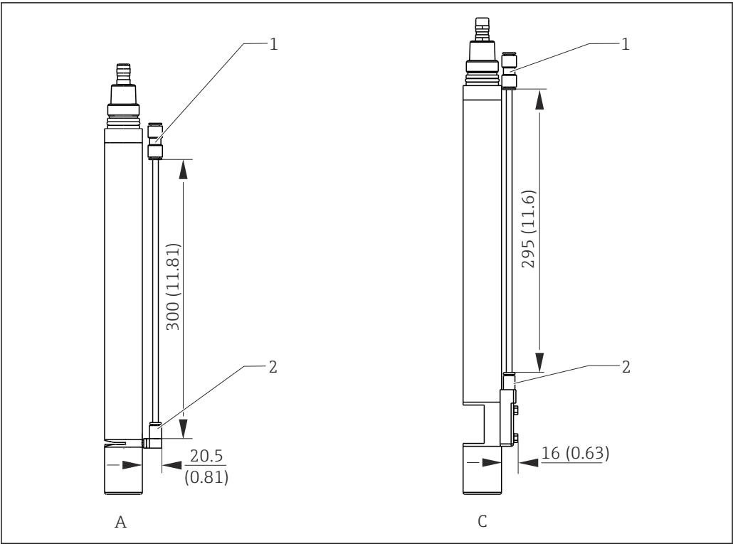
图 12 单位: mm (inch) 1 8 mm (0.31 in) 转接头, 带 300 mm (11.81 in) 软管 (仅针对 8 mm (0.31 in) 接头) 2 6 mm (0.24 in) 或 6.35 mm (0.25 in) 接头 A 传感器 (2 mm (0.08 in) 或 8 mm (0.31 in) 光程) C SAC 传感器 (40 mm (1.57 in) 光程)
