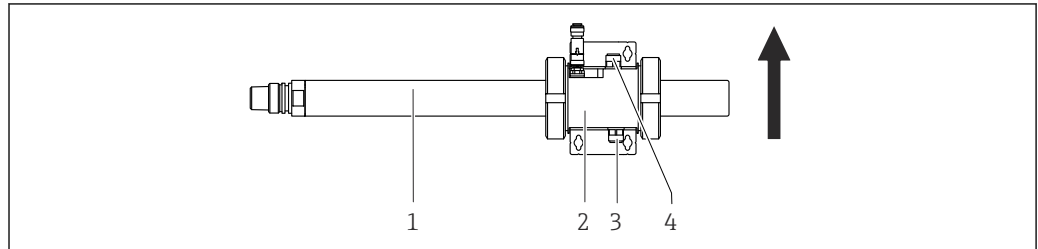
图 7 水平安装在 CAV01 流通式安装支架中，箭头指向与介质流向一致
