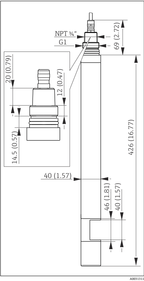
11 40 mm (1.57 in)光程的传感器的外形尺寸示意图; 单位: mm (in)
