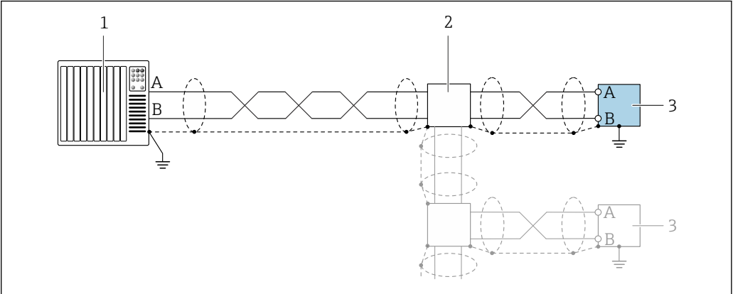
15 接线实例：Modbus RS485
