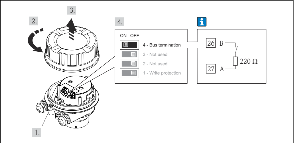
16 通过电子模块上的 DIP 开关开启终端电阻
