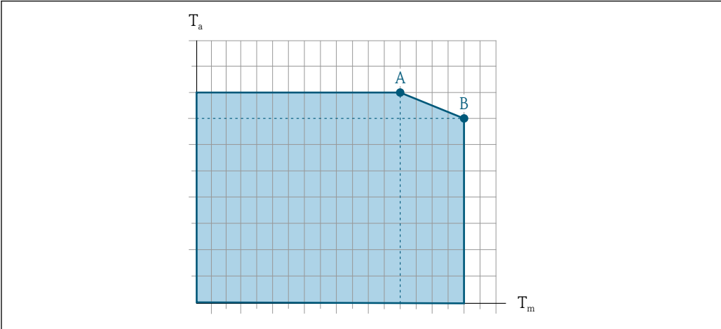
图 19 示例图，具体数值见下表。 Ta 环境温度 Tm 介质温度 A 介质温度 Tm 越高 (Ta max = 60 °C (140 °F)时)，所需的环境温度 Ta 越低 B 传感器最高允许介质温度 Tm 对应的最高允许环境温度 Ta
