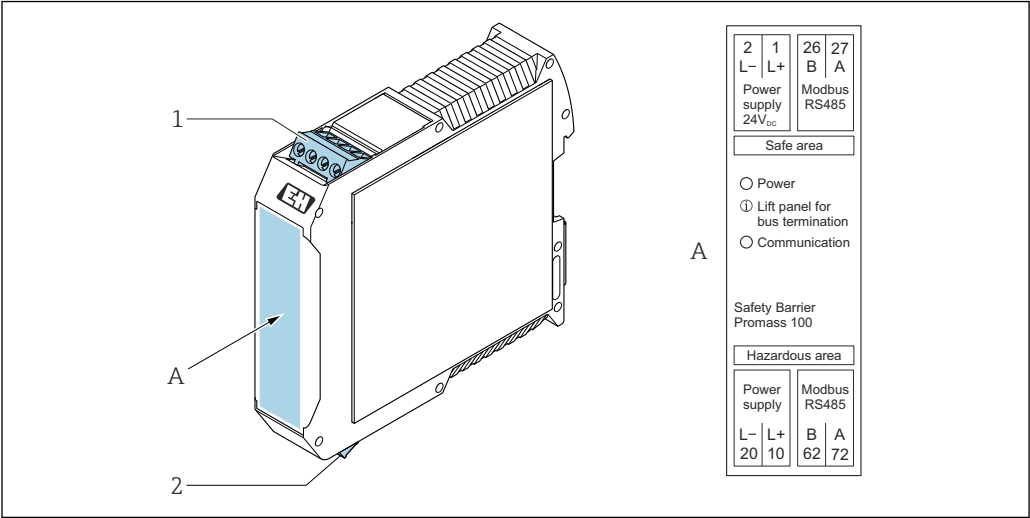
10 Promass 100 安全栅，带接线端子
