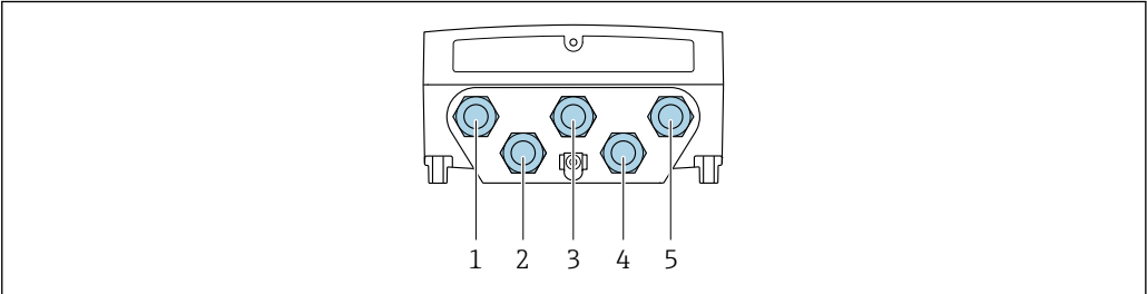
图 3 分体型仪表（墙装外壳）：连接电源和传输信号
