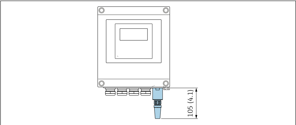
25 单位：mm (in)
