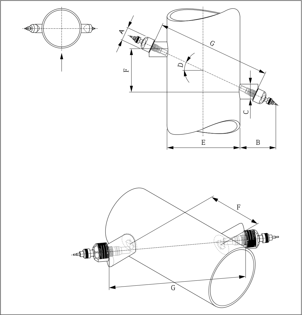
22 单路安装形式
