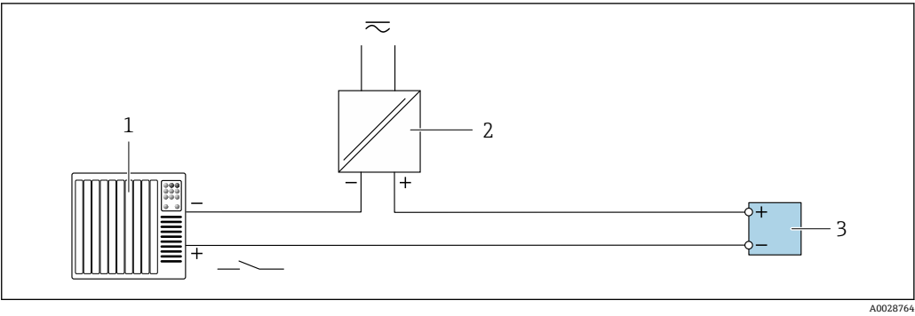
图 8 接线实例：状态输入
