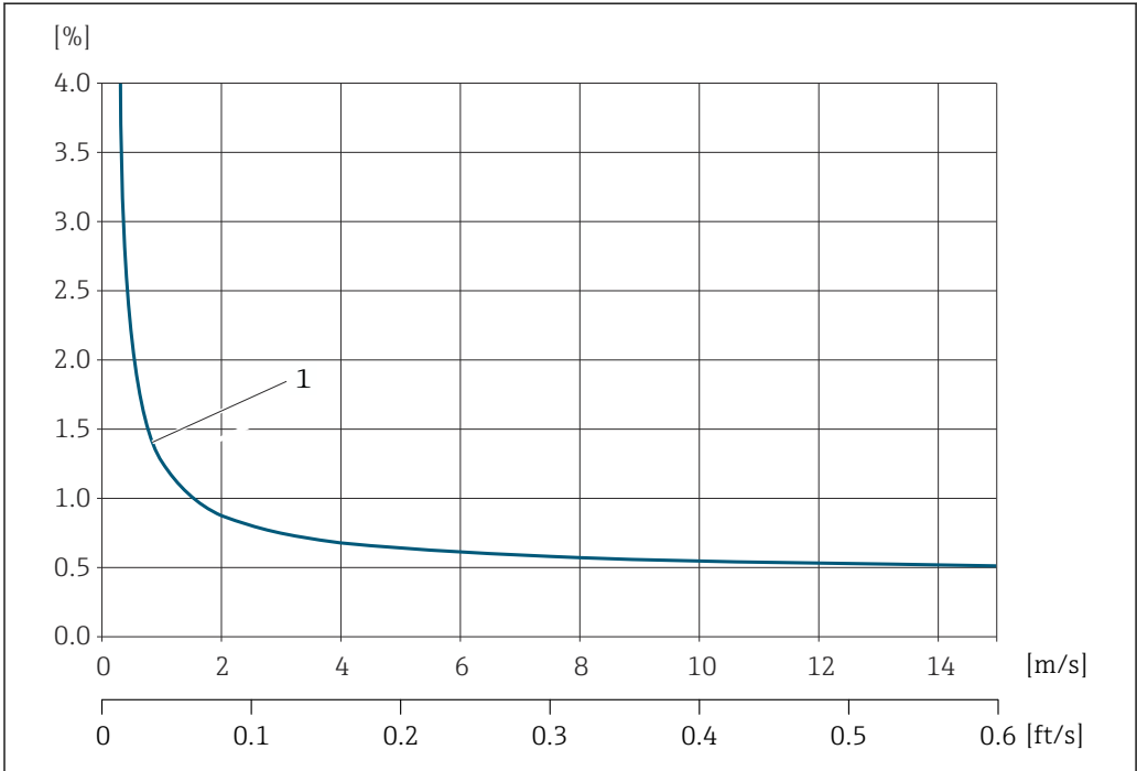
图 10 最大测量误差（体积流量）(% o.r.)的计算实例
