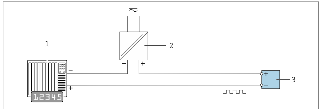
图 5 接线示例：脉冲/频率输出（无源信号）
