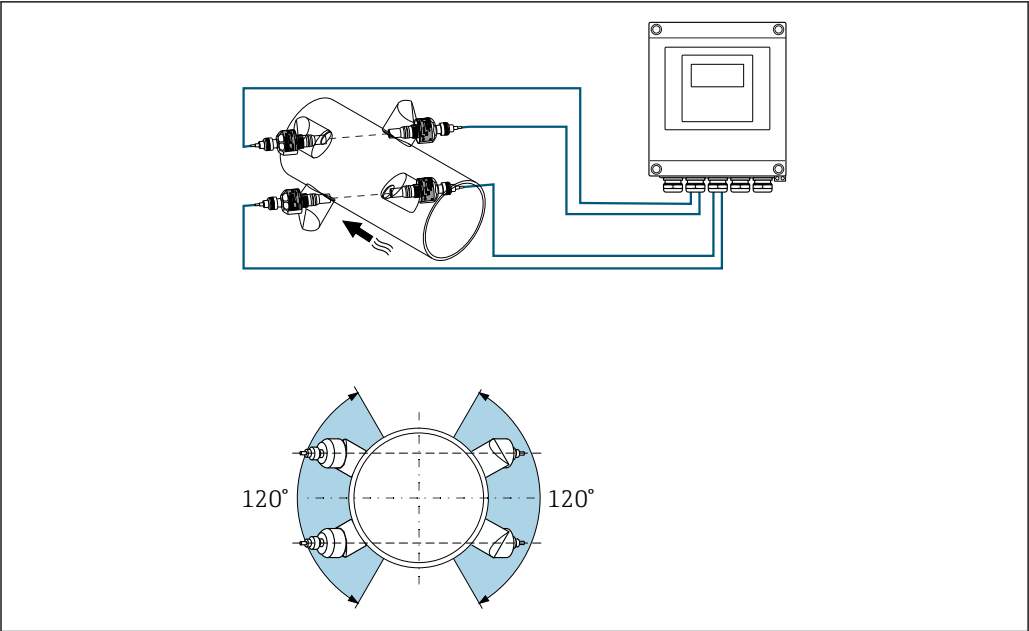
图 1 双声路测量：在测量点处水平布置传感器组的示意图
