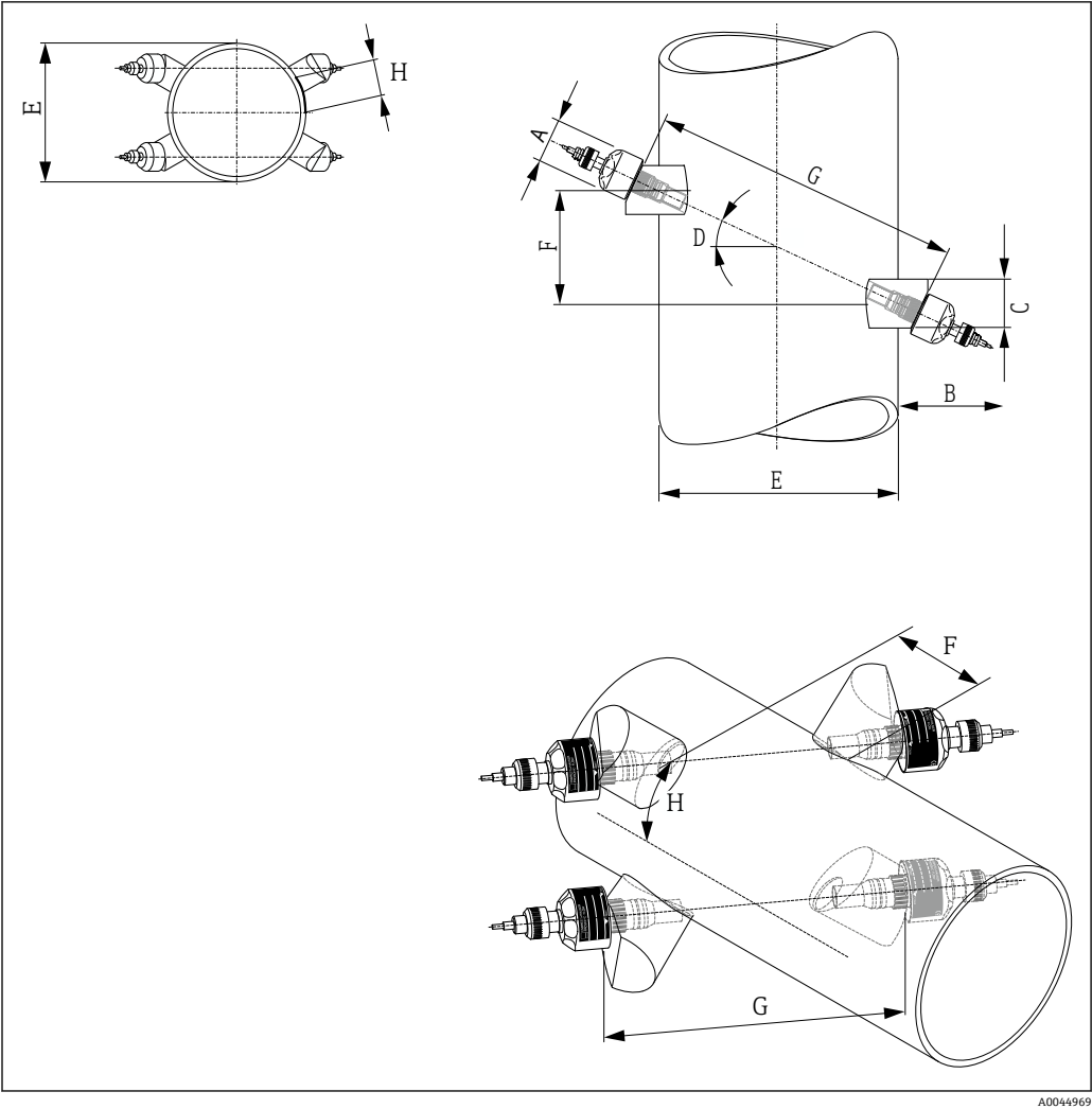
23 双路安装形式
