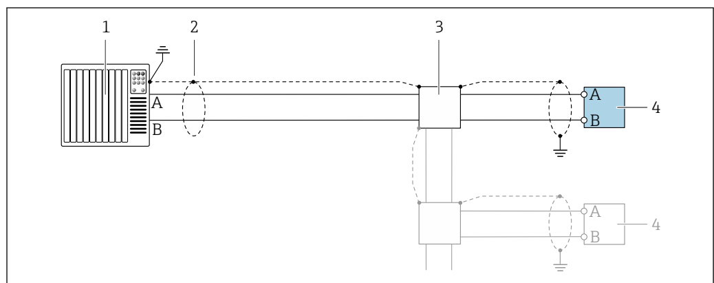
图 7 接线示例：Modbus RS485，非危险区和防爆 2 区/ Div. 2 防爆场合
