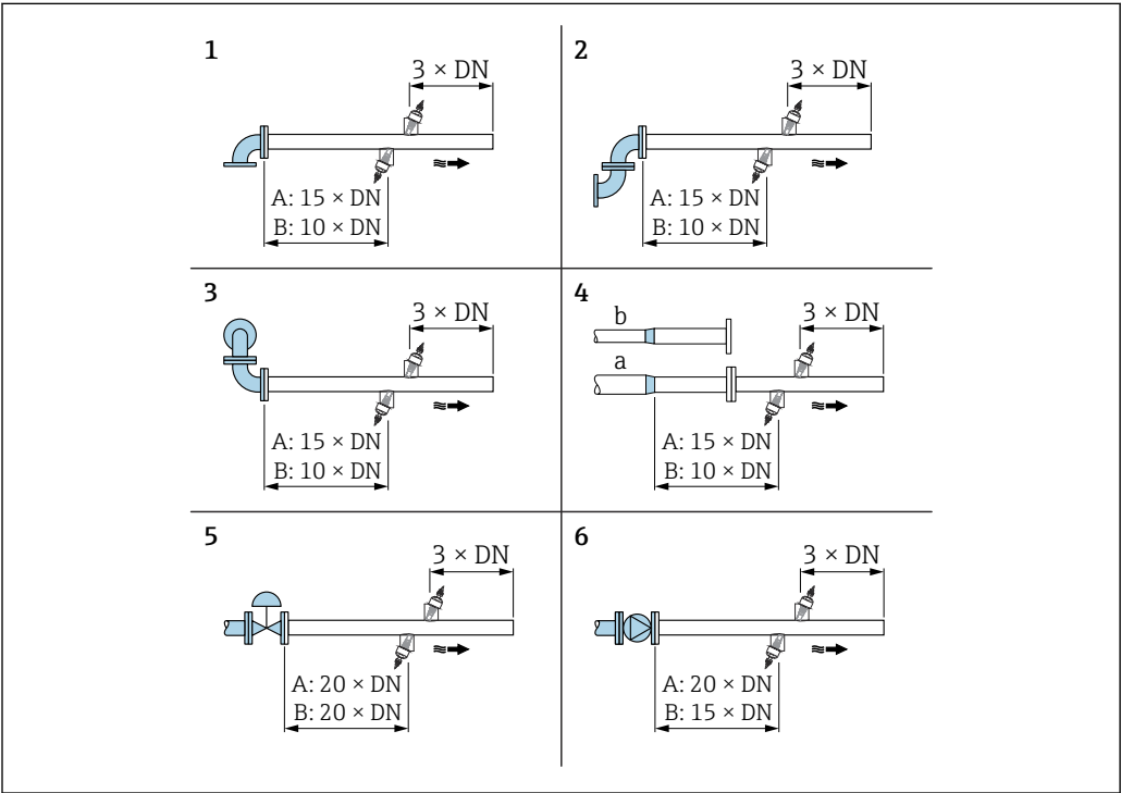
图 12 使用不同节流装置时的最小前后直管段长度 (A: 单声路测量, B: 双声路测量)
