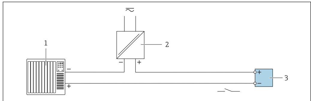
图 6 接线实例：开关量输出（无源信号）
