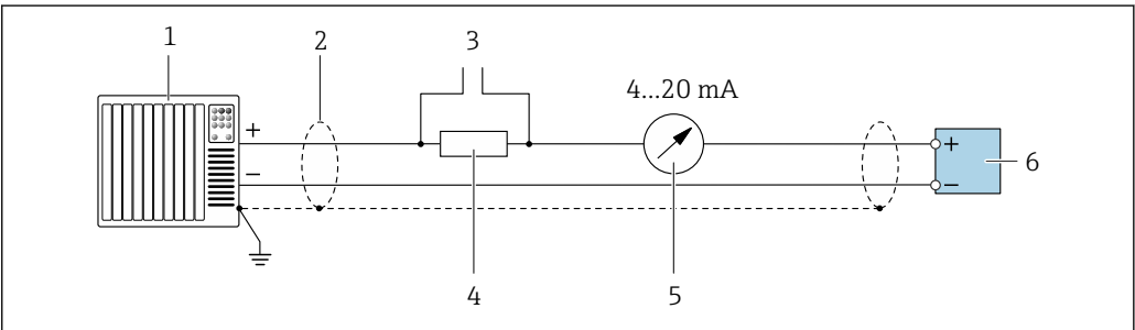
图 4 4...20 mA HART 电流输出（有源）的接线图
