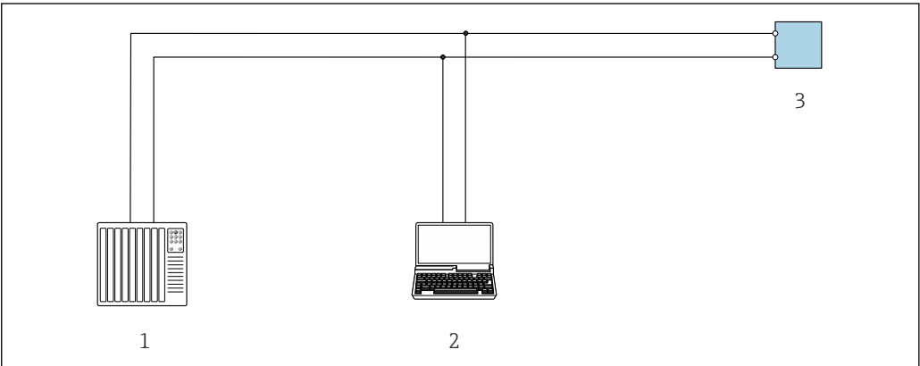
图 30 通过 Modbus RS485 通信进行远程操作（有源信号）
