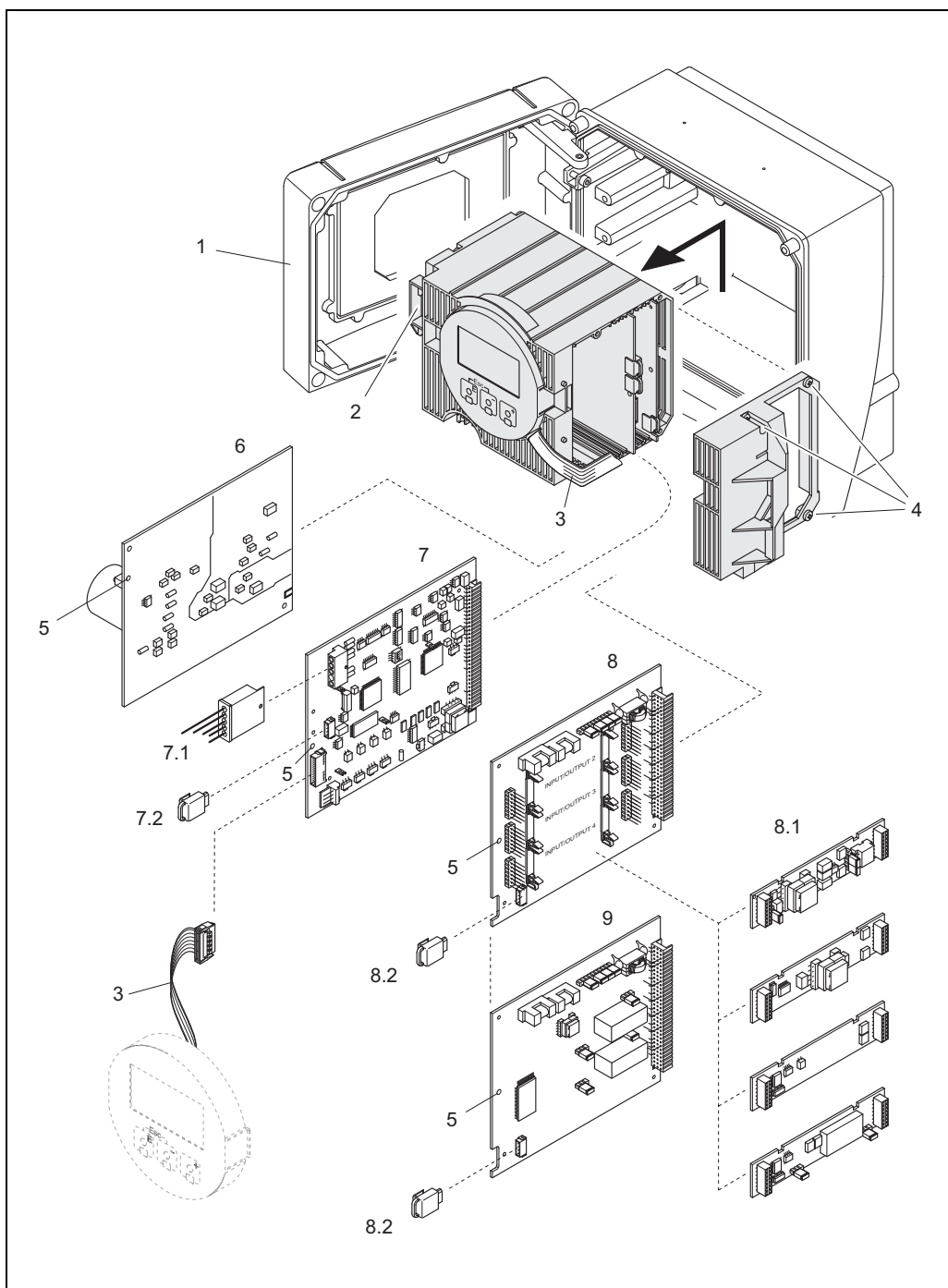
图 89: 墙装型外壳: 拆除和安装印刷电路板
