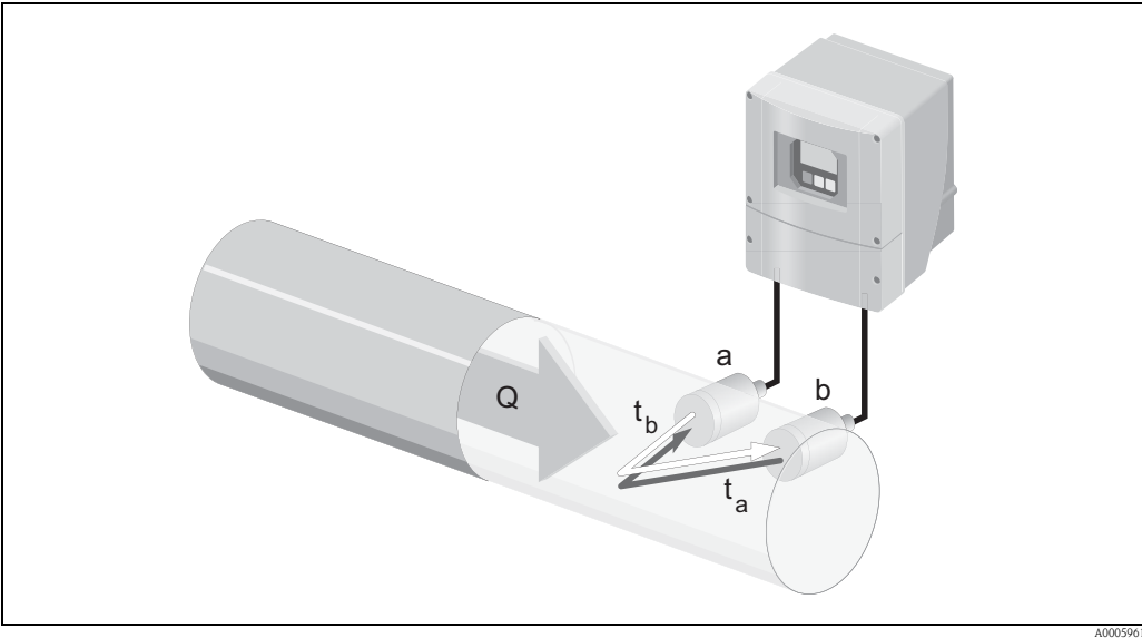
时差法测量原理示意图
