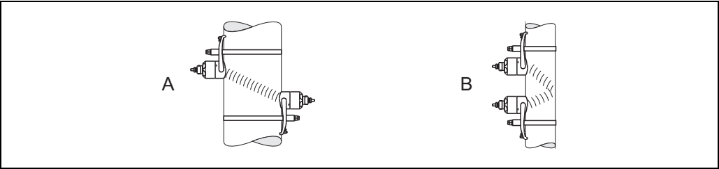
传感器的安装位置示意图
