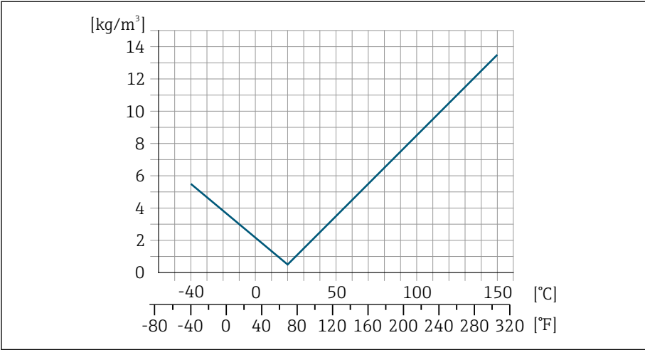
图 7 现场密度校准，例如在 +20^\circ\text{C} ( +68^\circ\text{F} ) 时
