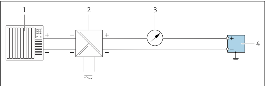
12 接线实例：4 ... 20 mA 电流输出（无源） 1 自动化系统，带电流输入（例如 PLC） 2 电源 3 可选附加显示单元：注意最大负载 4 变送器，带电流输出（无源）
