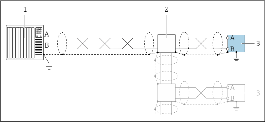
10 接线实例：Modbus RS485 1 自动化系统，带 Modbus 主站（例如 PLC） 2 可选分线盒 3 Modbus RS485 变送器
