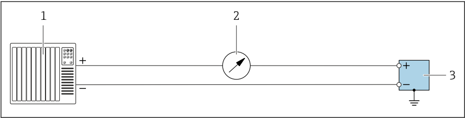
11 接线实例：4 ... 20 mA 电流输出（有源） 1 自动化系统，带电流输入（例如 PLC） 2 可选附加显示单元：注意最大负载 3 流量计，带电流输出（有源）
