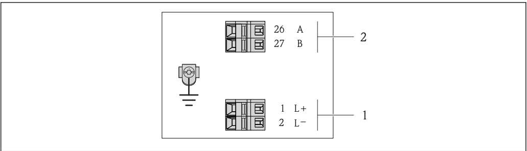
图 8 Modbus RS485 型仪表的接线端子分配示意图, 连接类型适用于在非危险区和 2 区/Div. 2 防爆场合中使用
