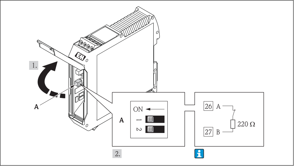
15 通过 Promass 100 安全栅上的 DIP 开关开启终端电阻
