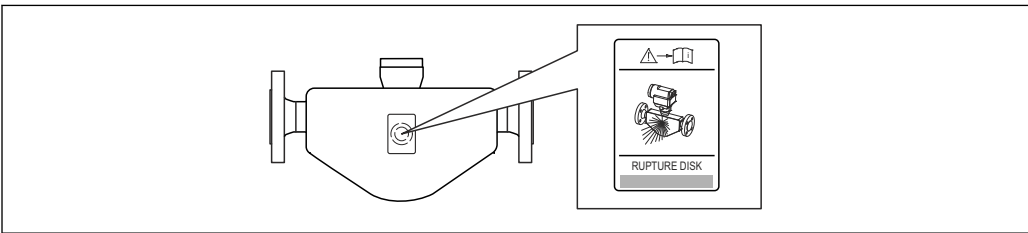
图 7 爆破片标签示意图
