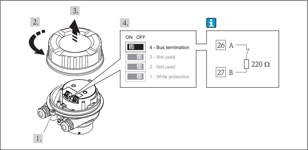
14 通过主要电子模块上的 DIP 开关开启终端电阻
