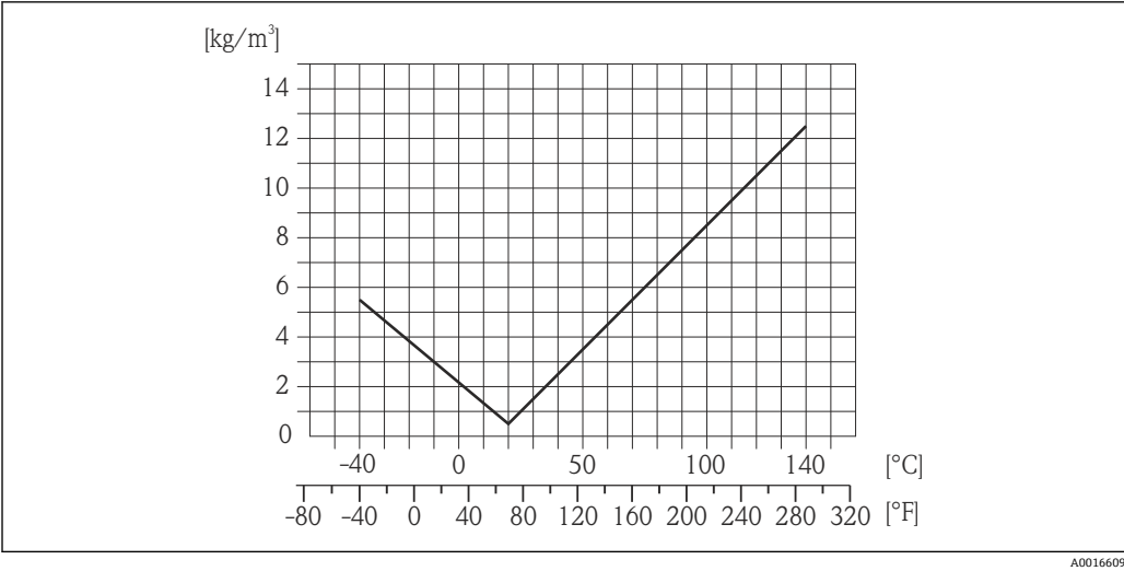
图 17 现场密度标定，例如，在+20 °C (+68 °F)时
