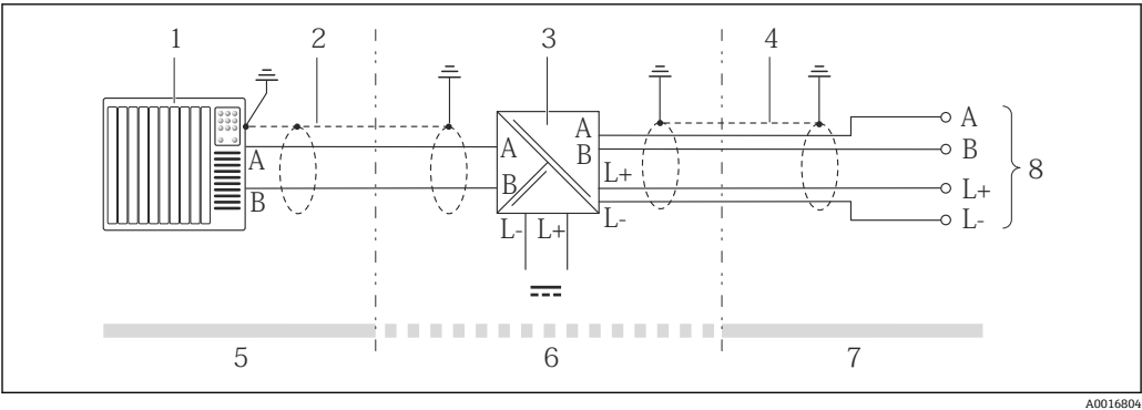
图 13 变送器和 Promass 100 安全栅间的电气连接
