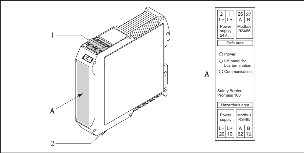
图 10 Promass 100 安全栅的接线端子示意图
