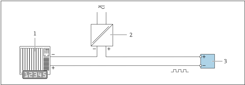
图 20 脉冲/频率输出(无源信号)的连接实例
