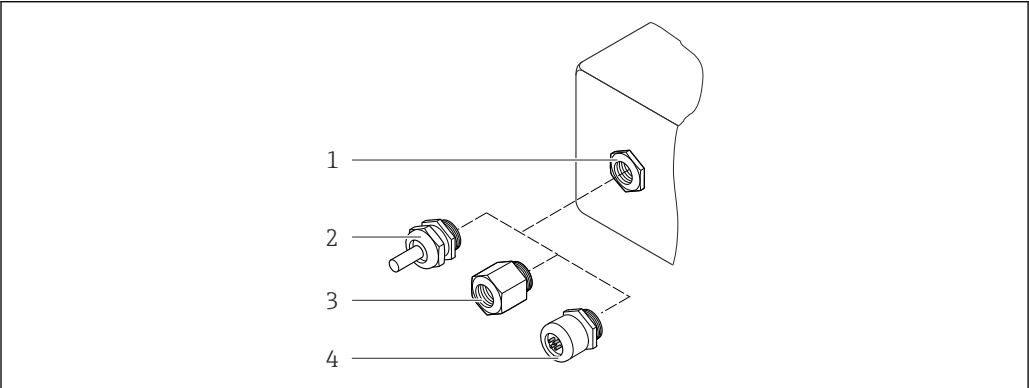
图 38 允许的电缆入口/缆塞 1 M20 × 1.5 内螺纹电缆入口 2 M20 × 1.5 缆塞 3 适配接头，适用于带 G ½"和 NPT ½"内螺纹的电缆入口 4 仪表插头
