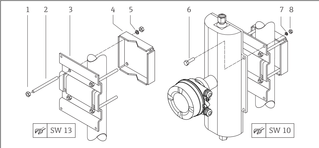
图 8 柱式安装套件
