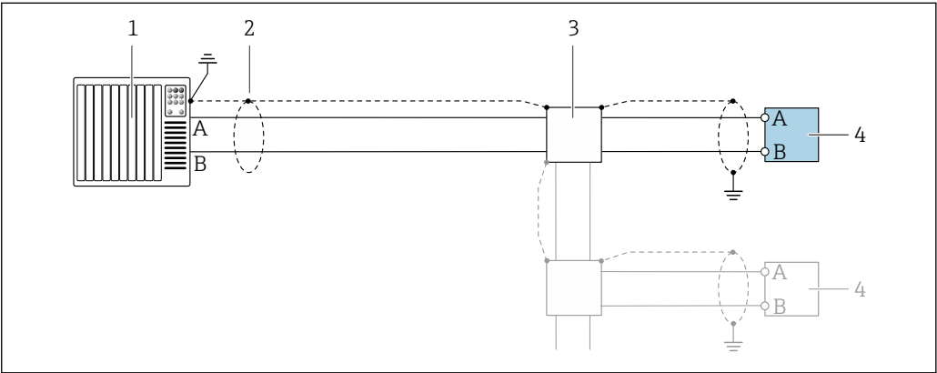
图 7 Modbus RS485 的连接实例, 在非危险区和 2 区/ Div. 2 防爆场合中
