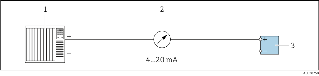
图 8 4...20 mA 有源电流输出的连接实例 1 带电流输入的自动化系统(例如: PLC) 2 模拟式显示单元: 注意最大负载 3 变送器
