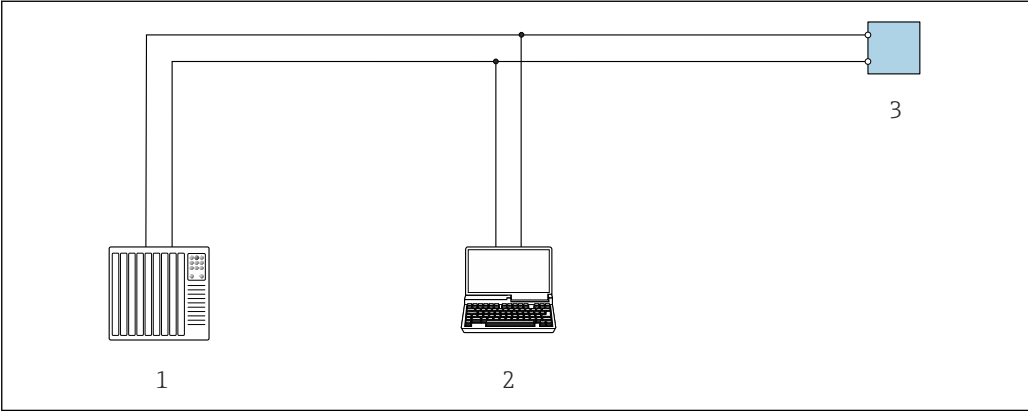
图 19 通过 Modbus-RS485 通信进行远程操作(有源信号)
