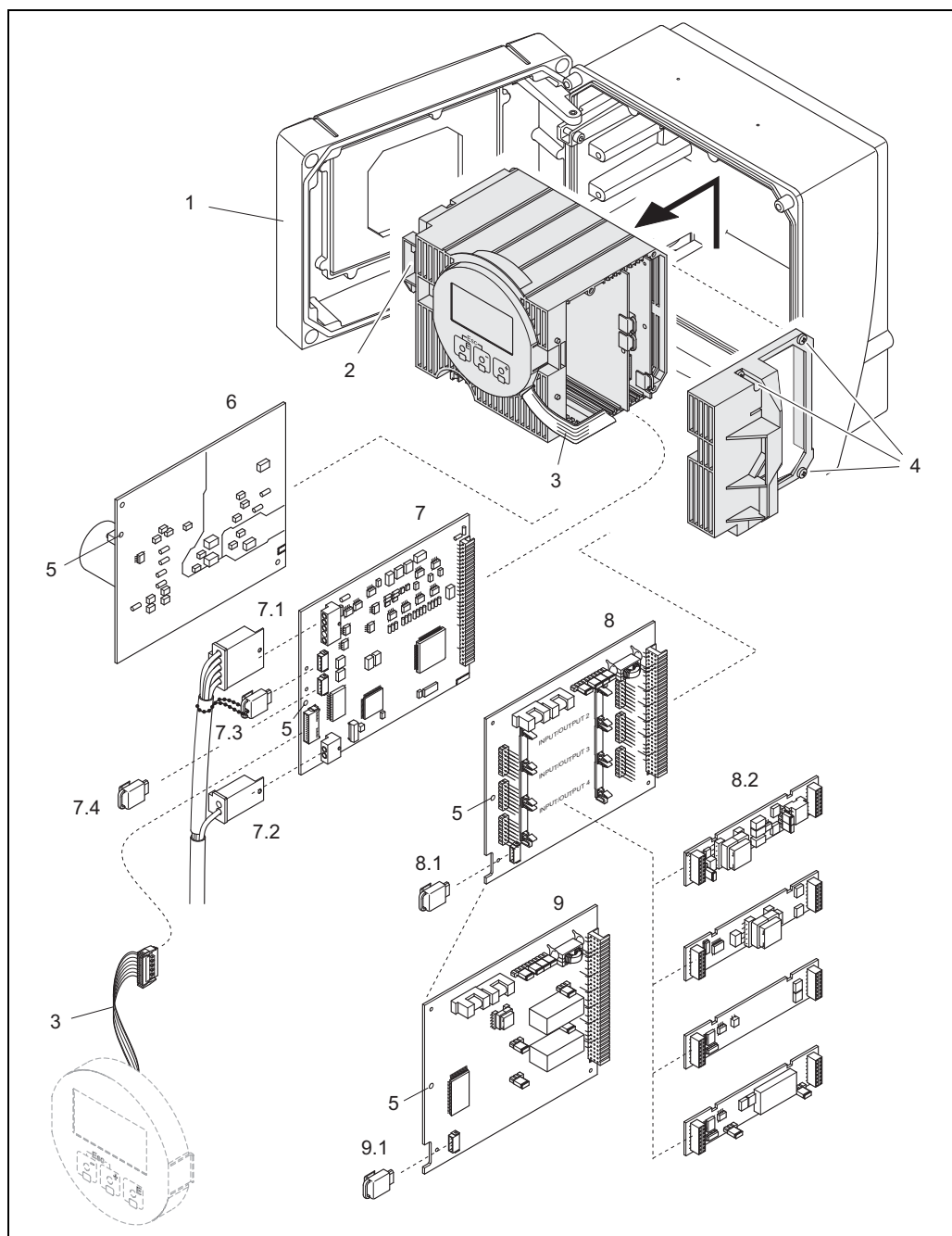
图 48: 墙装型外壳：拆除和安装印刷电路板
