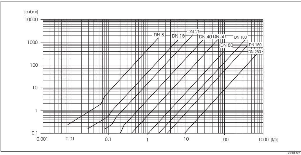
图 59: 水的压损曲线图
