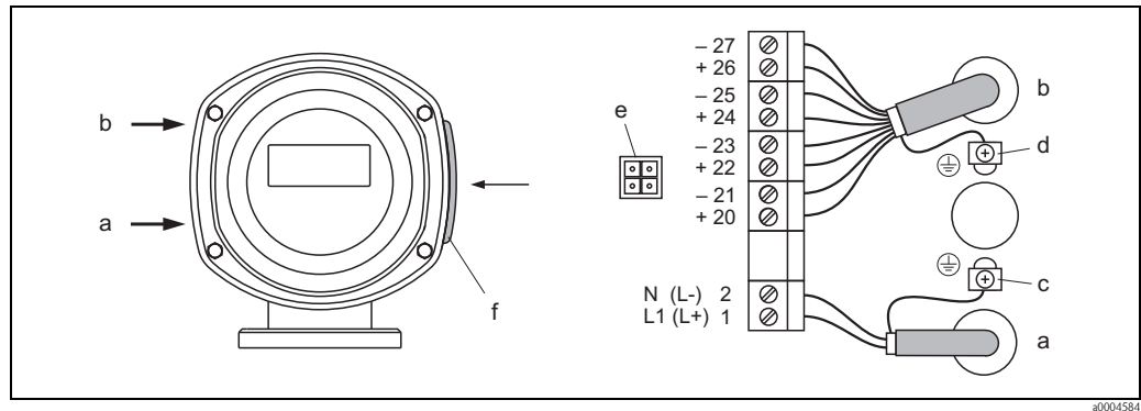
图 23: 变压器 (现场型不锈钢外壳) 的电气连接示意图, 连接电缆的横截面积: max. 2.5 mm 2
