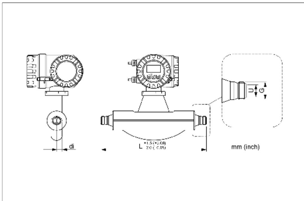
ISO 2853螺纹(卫生型): 1.4404/316L
