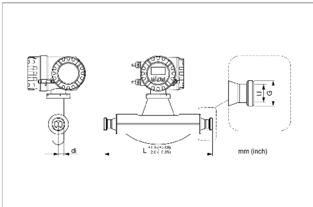
DIN 11864-1 Form A螺纹(卫生型): 1.4404/316L
