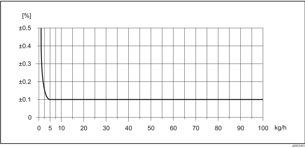
最大测量误差 (% o.r.) 的计算实例 (Promass 80A, 83A: DN 2)
