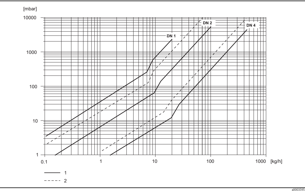
水的压损曲线图
