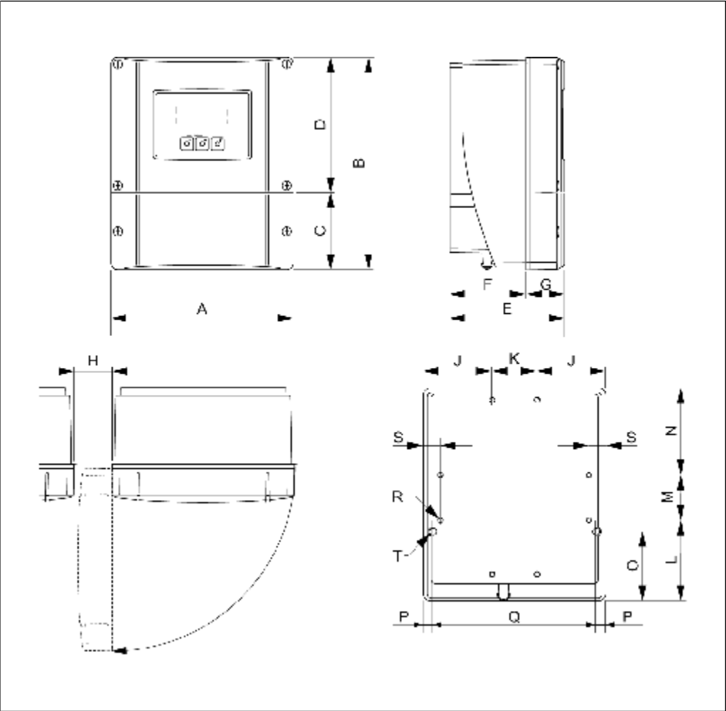
分体式墙装变送器外壳(非防爆区和II3G/2区)
