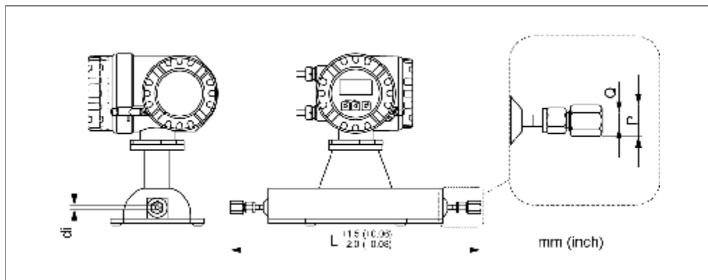
安装组件1/4" NPT-F连接: 1.4539/904L、Alloy C-22
