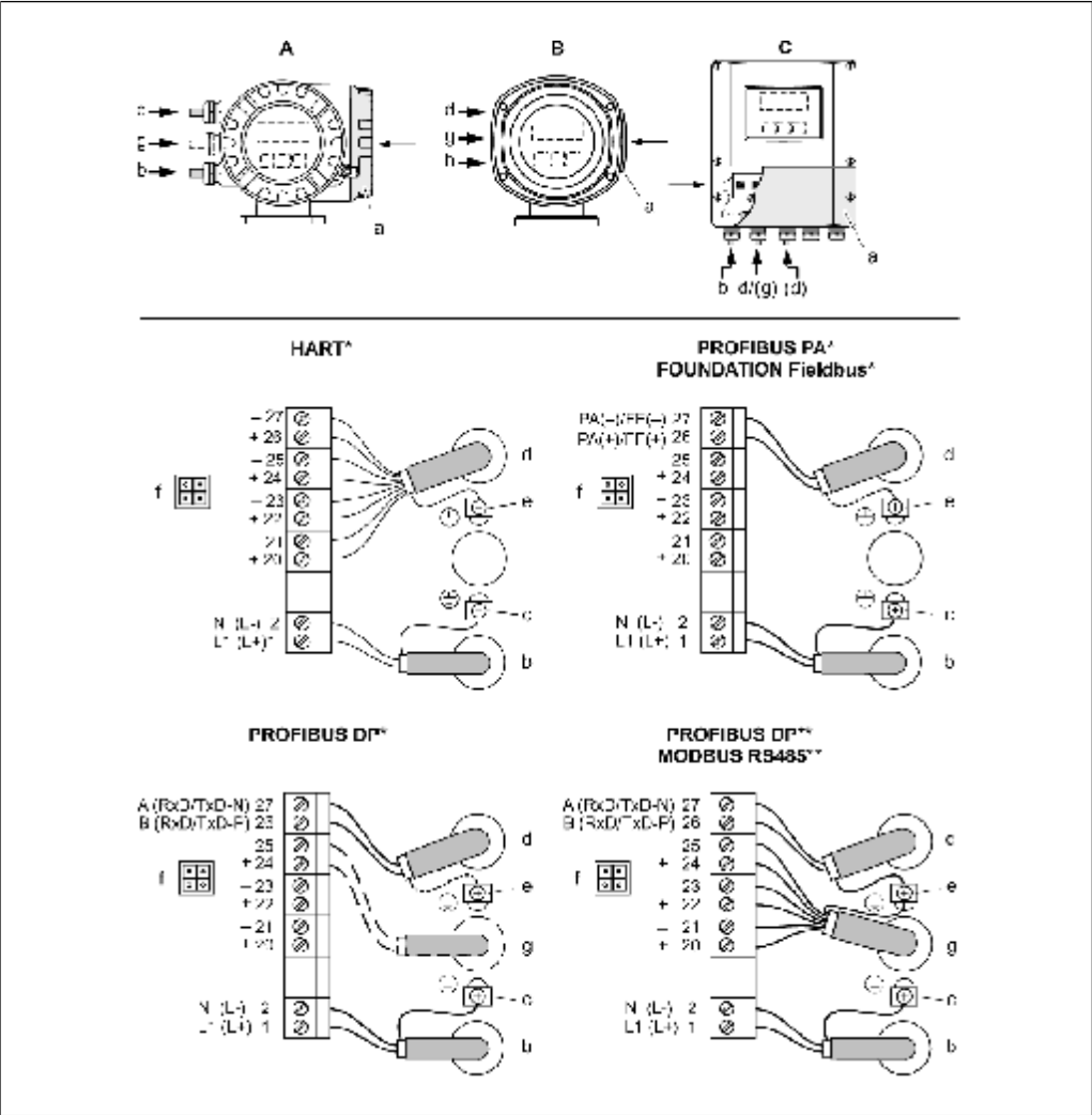
Promass变送器的电气连接示意图，连接电缆的最大横截面积为2.5 mm 2
