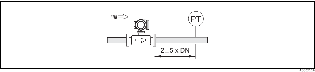
压力测量点的安装示意图 (PT = 压力变送器)
