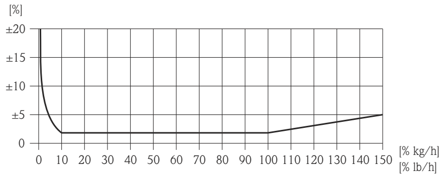
最大测量误差 (% 质量流量 (Q)) % 满量程值，参考下表
