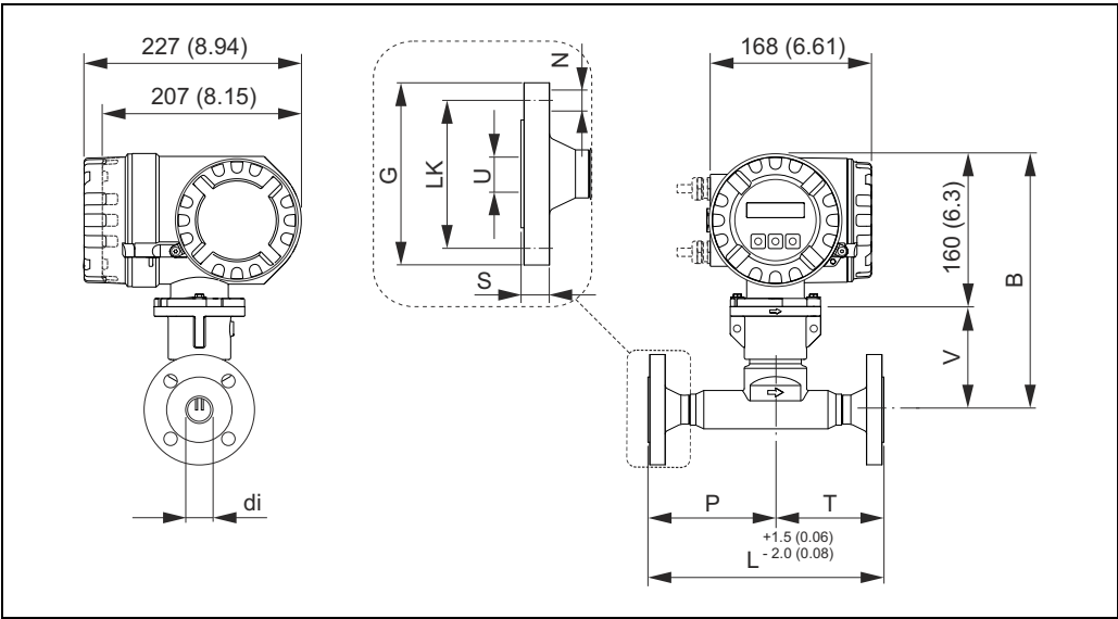
t-mass 65F : ANSI 法兰连接
