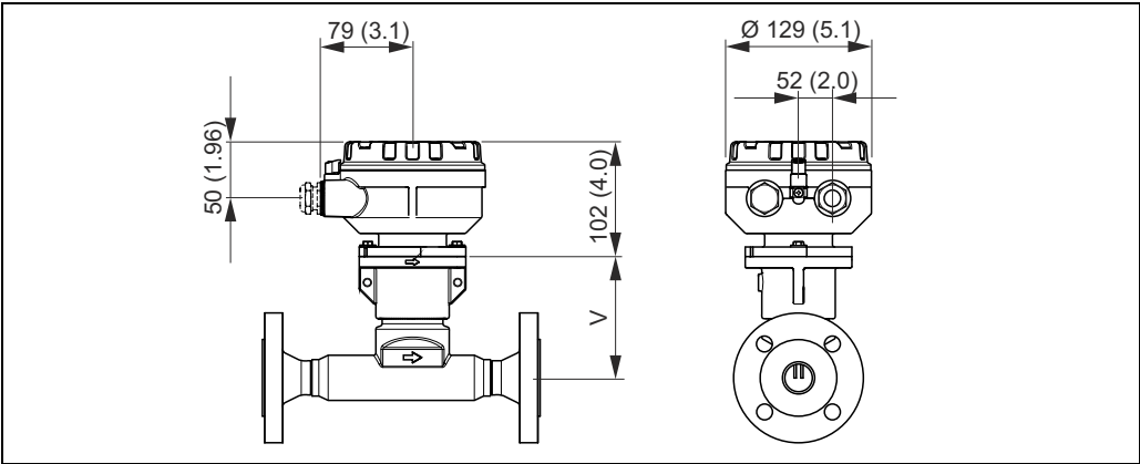
单位：mm (in)；外形尺寸“V”：→ 📄 30 和 → 📄 32
