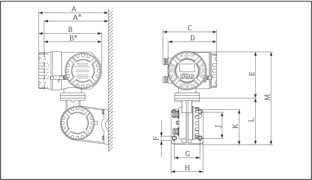
分体式变送器的接线盒 (II2G/1 区防爆场合 )
