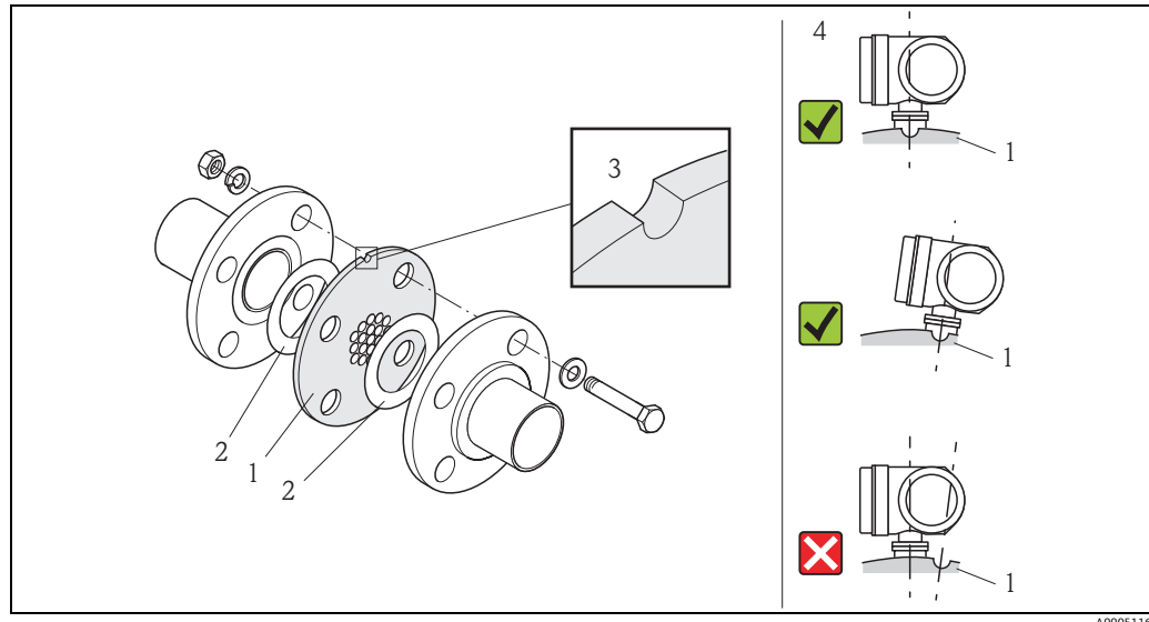
流量调节器的安装示意图 (安装实例)
