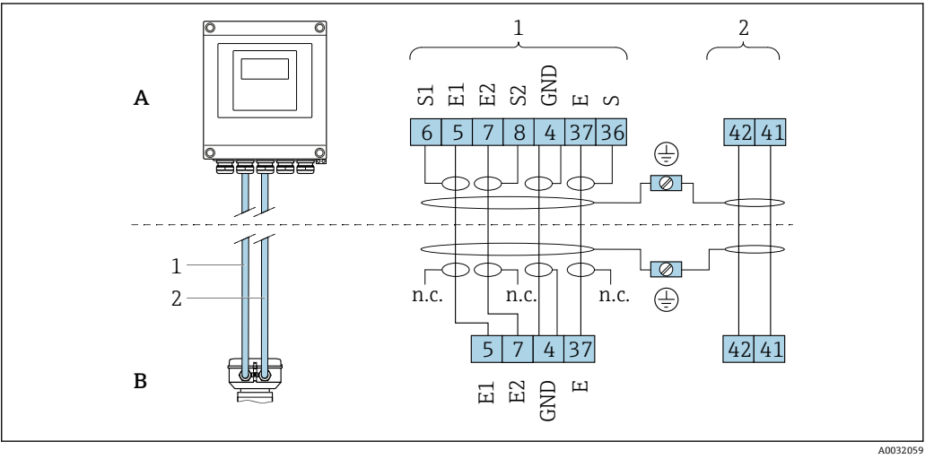
图 6 分体式仪表的接线端子分配
