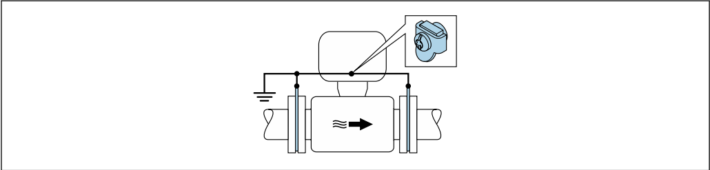
图 19 通过接地端子和接地环实现系统电势平衡
