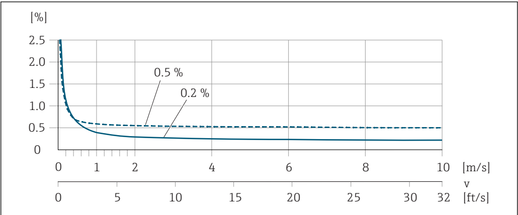
图 36 最大测量误差 (% o.r.)
