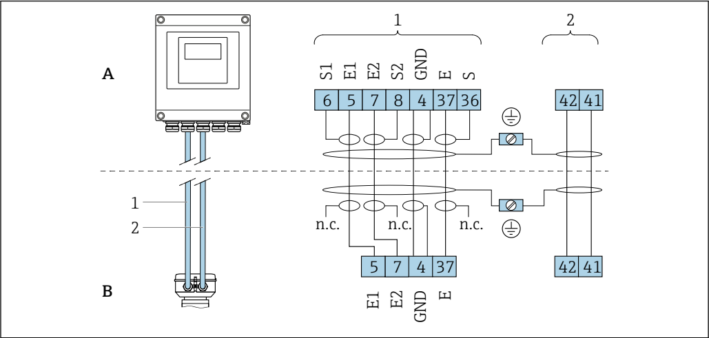
图 11 分体式仪表的接线端子分配
