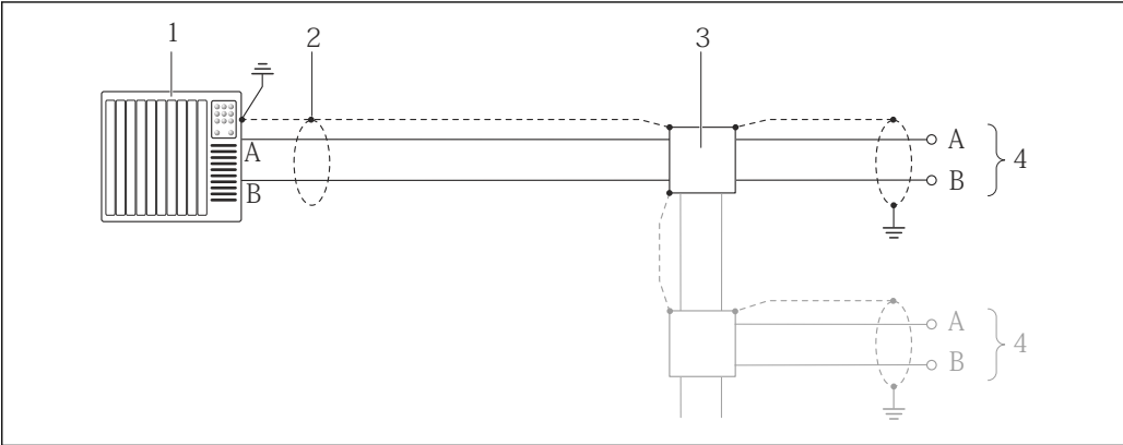
图 15 Modbus RS485 的连接示例，在非危险区和 2 区/ Div. 2 防爆场合中
