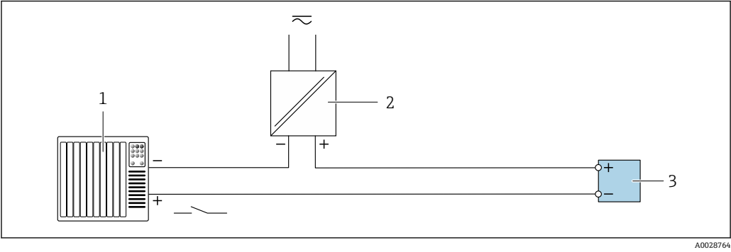
图 21 状态输入的连接实例
