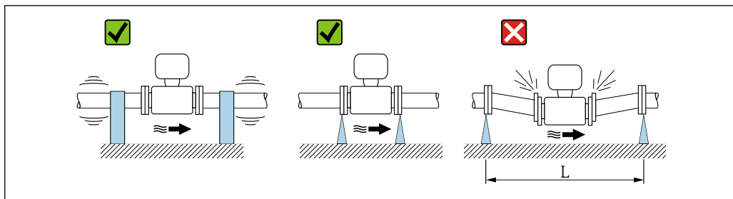
5 避免仪表振动的措施( L > 10\text{ m} (33 ft))
