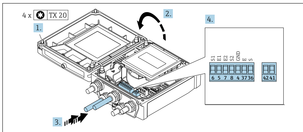
图 15 变送器：带接线端子的主要电子模块
