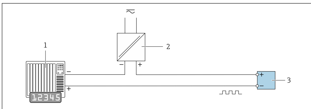
图 19 脉冲/频率输出(无源信号)的连接实例
