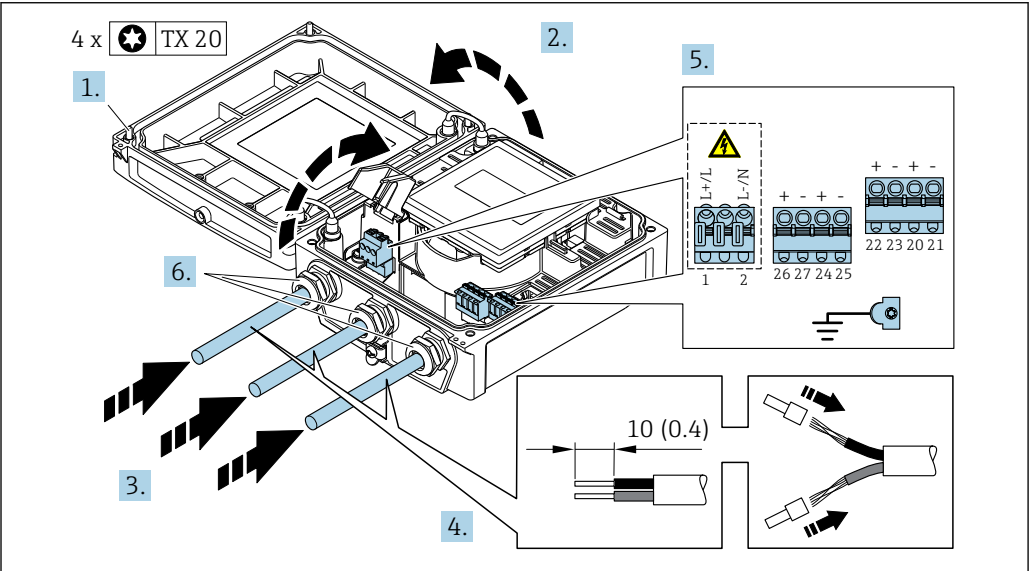
图 16 电源和 0...20 mA / 4...20 mA HART 的连接示意图，带附加输出和输入
