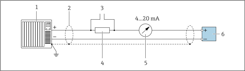
图 17 4...20 mA HART 电流输出(有源)的连接实例
