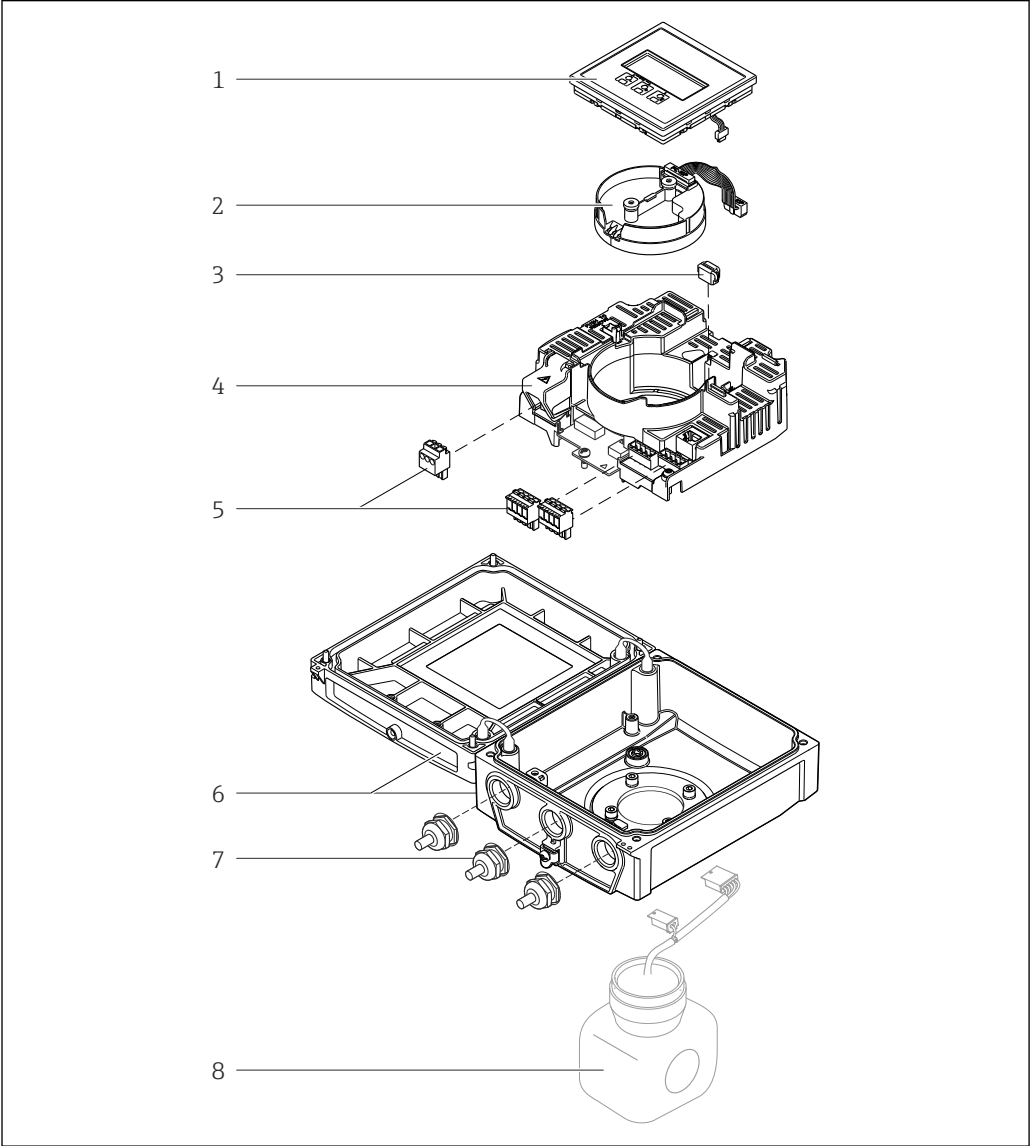
图 1 一体式仪表的重要部件
