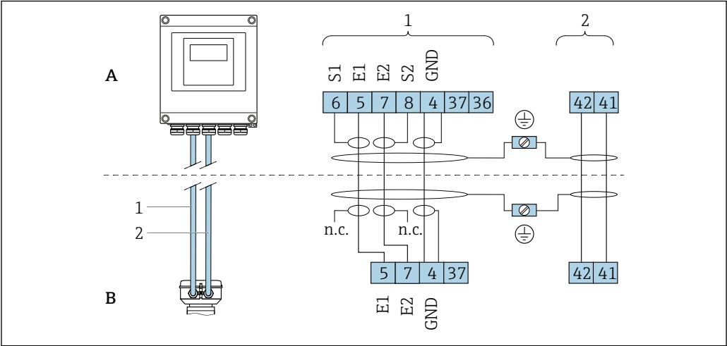
图 11 分体式仪表的接线端子分配
