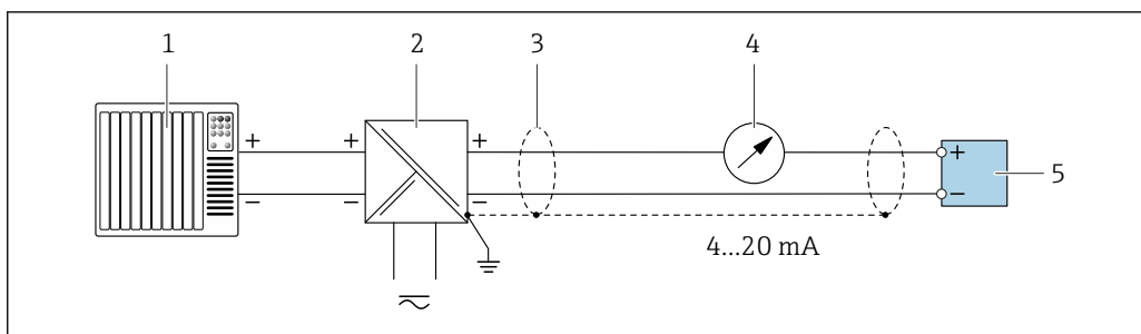
图 18 4...20 mA HART 电流输出(无源)的连接示例
