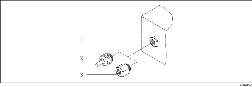
34 允许的电缆入口/缆塞 1 M20 × 1.5 内螺纹电缆入口 2 M20 × 1.5 缆塞 3 适配接头，适用于带 G ½"和 NPT ½"内螺纹的电缆入口
