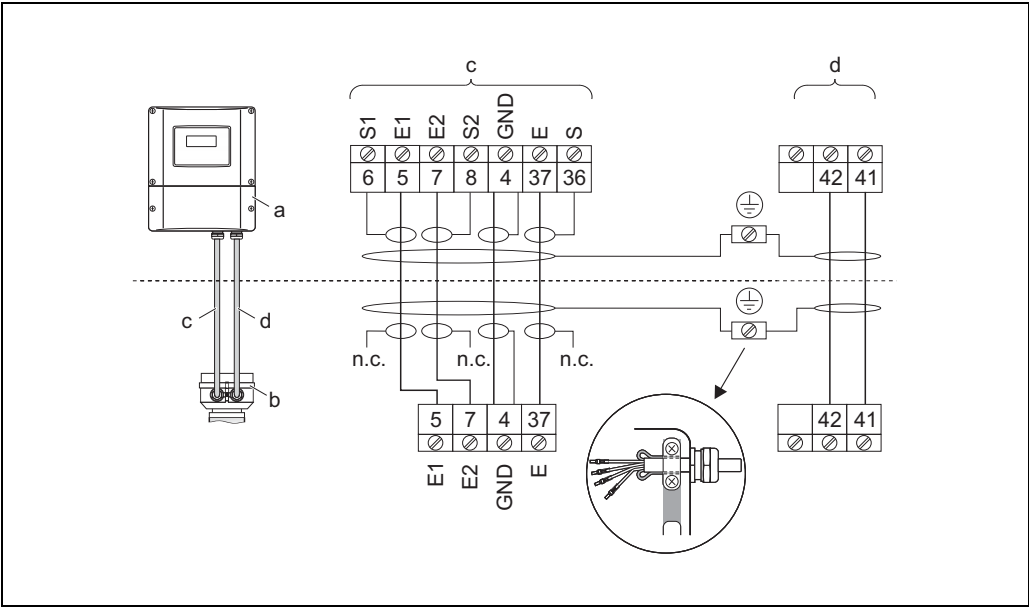
图 29: 分体式 Promag H 的电气连接示意图
