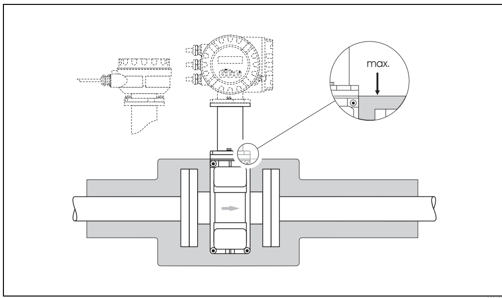
图 19: Promag P 传感器 (高温型) 的安装示意图: 管道隔热
