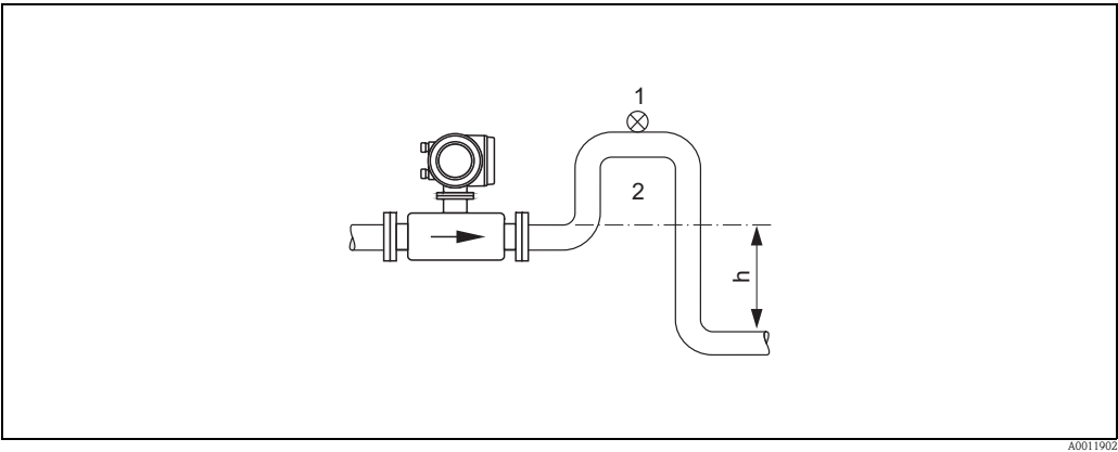
图 9: 在竖直向下管道中安装
