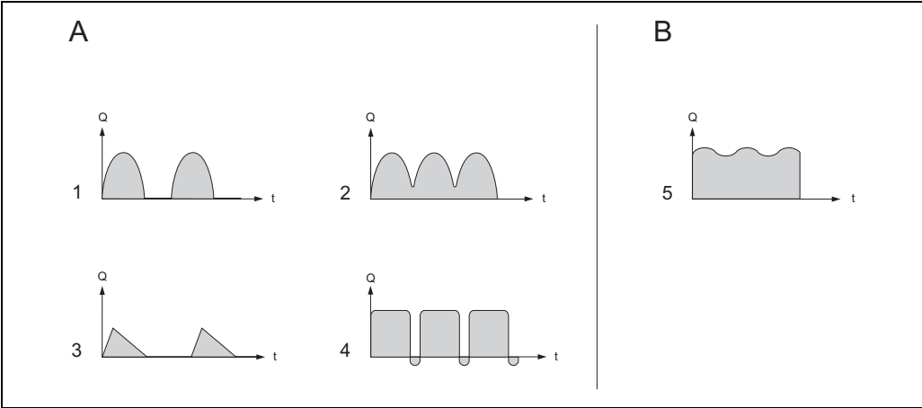
图 48: 各类泵的流量特征曲线图
