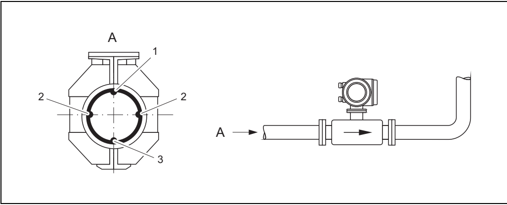
图 11: 水平管道安装示意图
