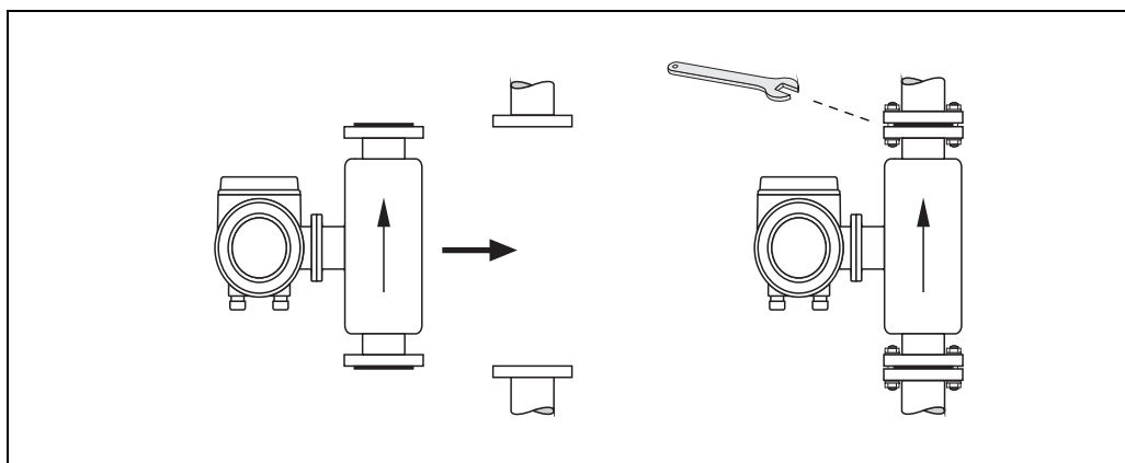
图 18: Promag P 传感器的安装示意图
