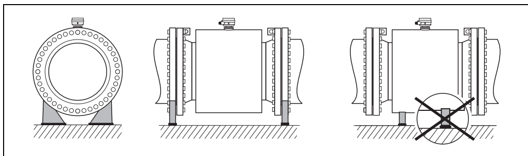
图 14: 正确安装大标称口径的传感器 ( DN \geq 350 (14"))
