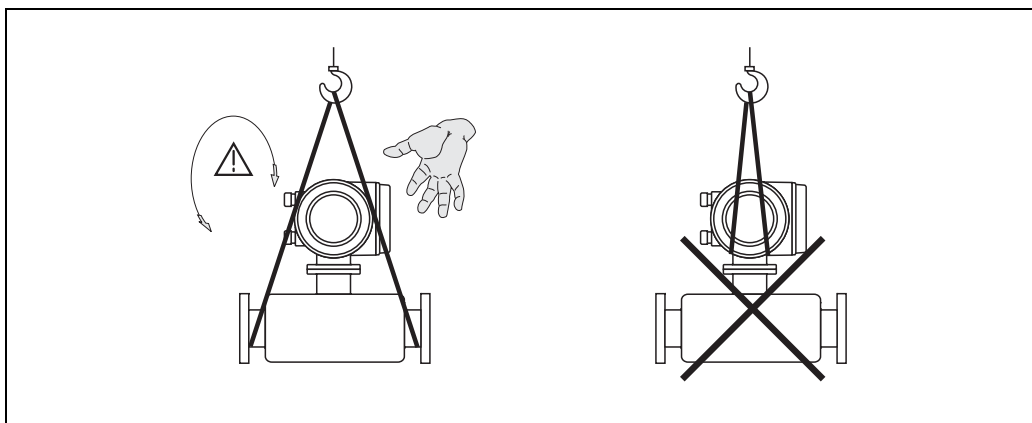
图 4: 传感器 ( \leq DN 300 (12")) 的运输指南示意图
