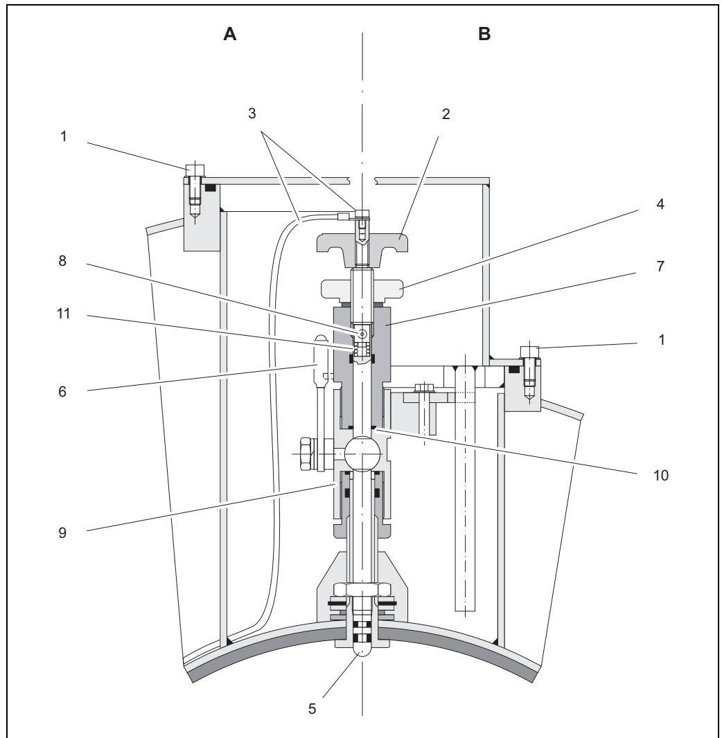
图 61: 更换设备的可更换电极
