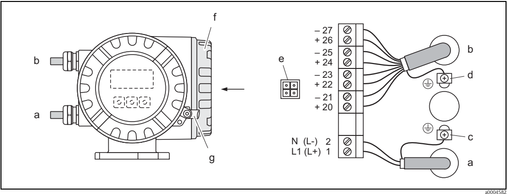
图 31: 变送器 (现场型铝外壳) 的电气连接示意图，连接电缆的横截面积：max. 2.5 mm 2
