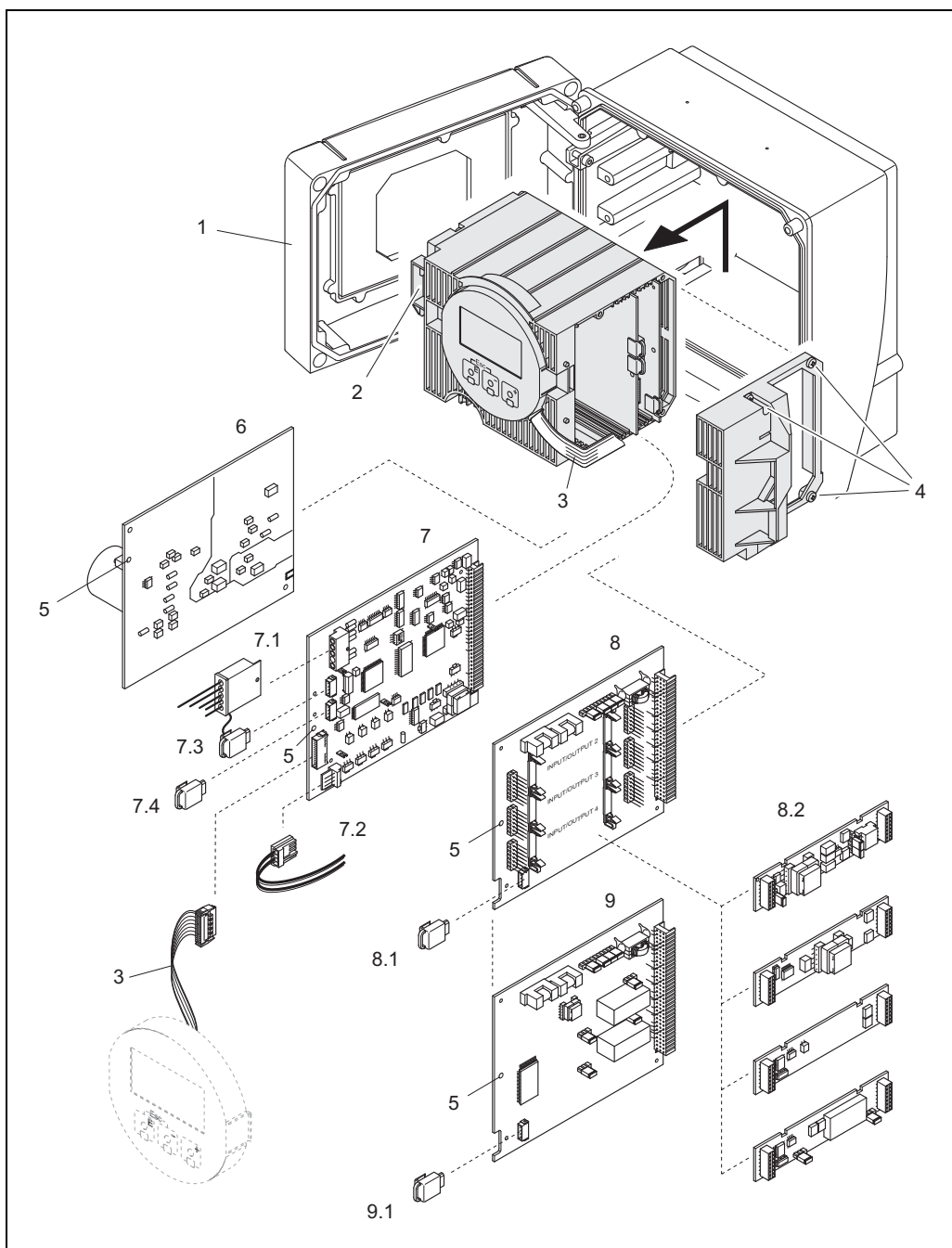
图 59: 墙装型外壳: 拆除和安装印刷电路板
