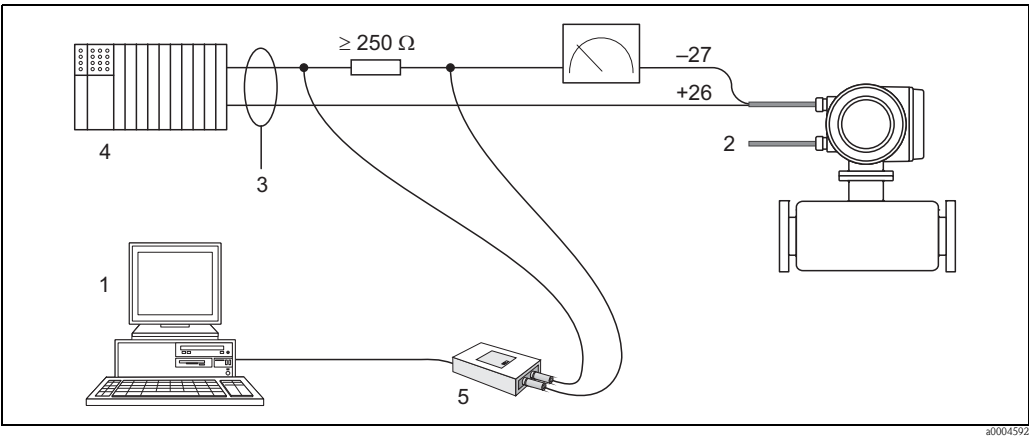
图 35: 安装有调试工具的 PC 机的电气连接示意图
