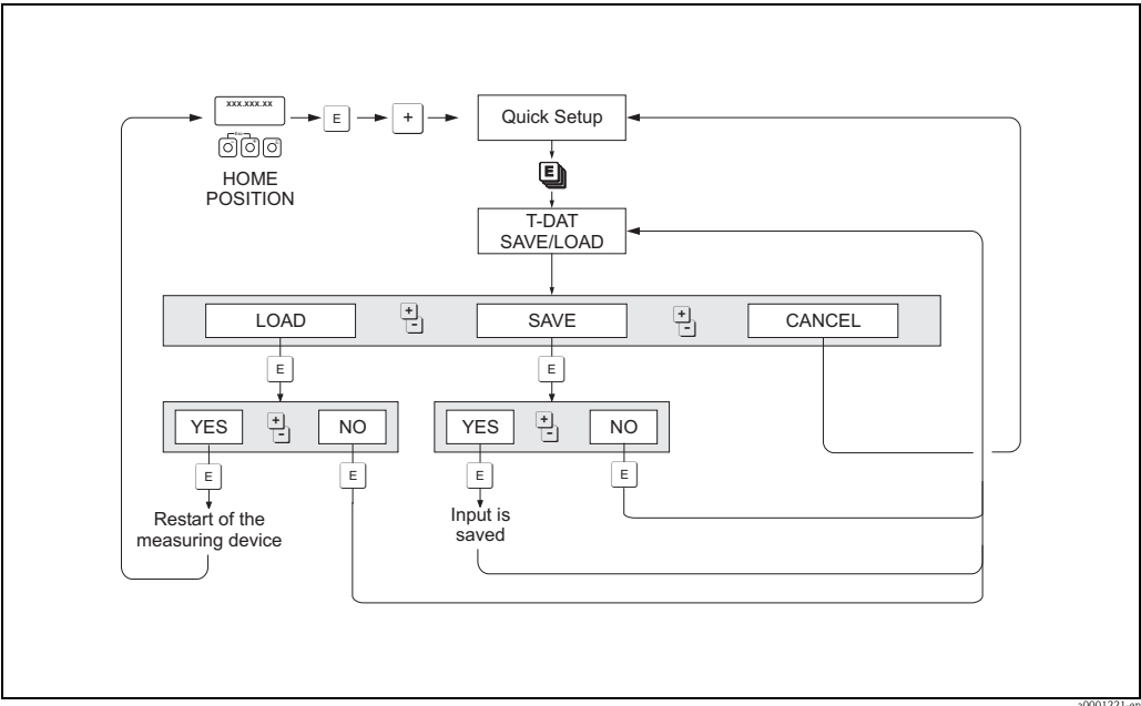
图 51: 使用 T-DAT 保存 / 上传功能进行数据备份 / 传输
