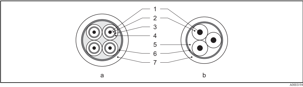
图 30: 电缆横截面示意图
