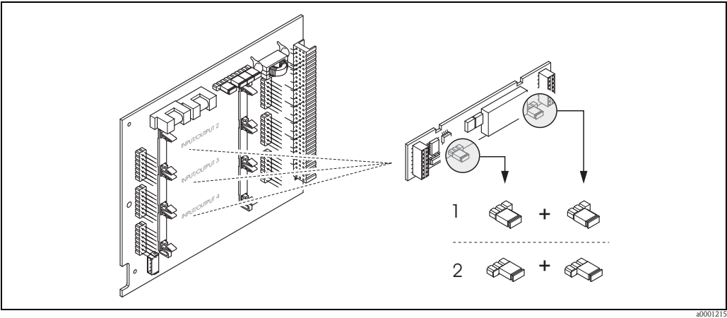
图 55: 可灵活设置 I/O 板 (子模块) 上的继电器触点 (NC / NO) 设置 )
