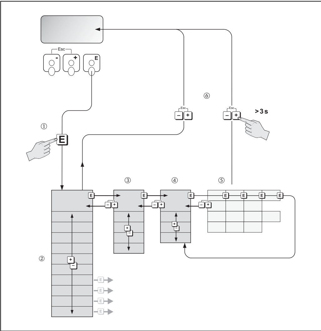
图 44: 选择功能参数和设置参数 (功能菜单)
