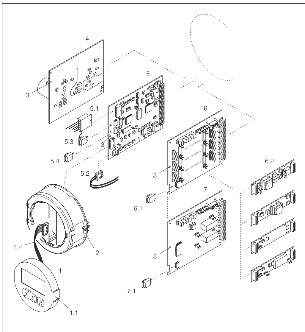
图 58: 现场型外壳: 拆除和安装印刷电路板
