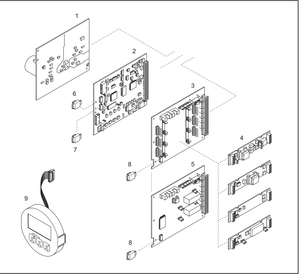
图 57: Promag 变送器的备件 ( 现场型外壳和墙装型外壳 )
