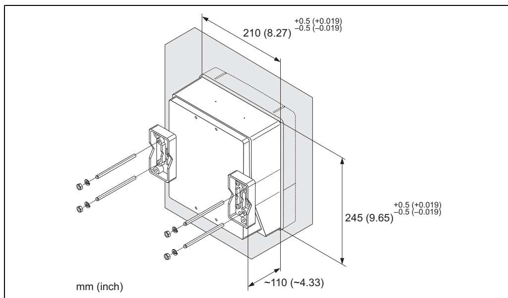
图 26: 盘式安装 ( 墙装型外壳 )
