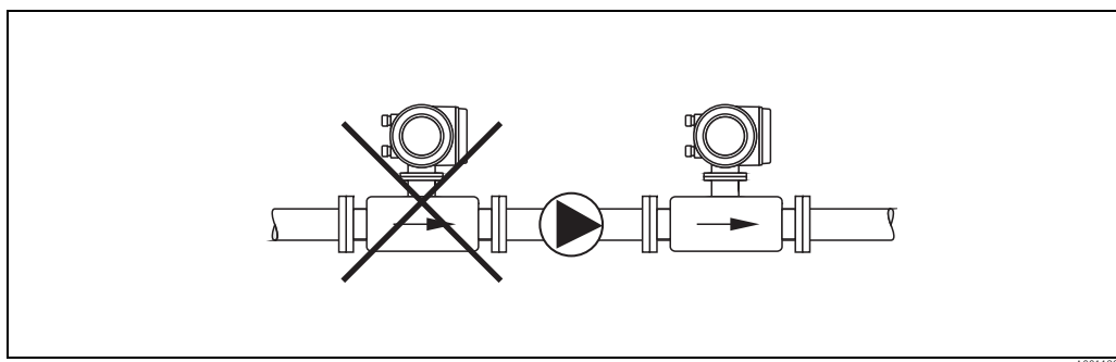
图 7: 使用泵时的安装位置示意图
