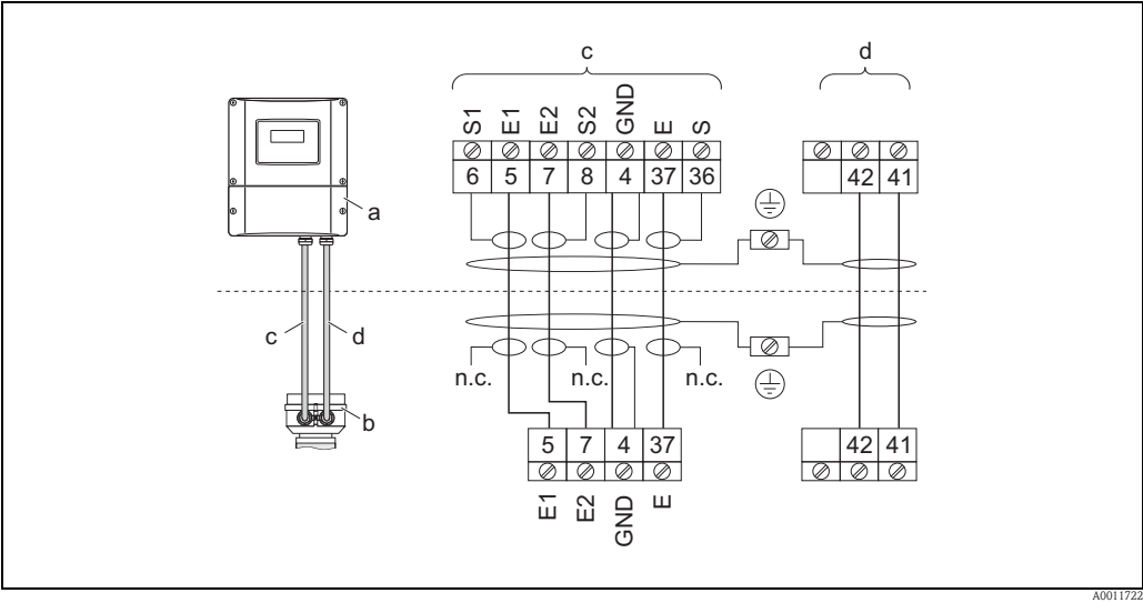
图 28: 分体式 Promag W、P 的电气连接示意图
