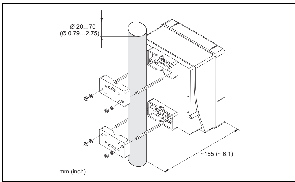
图 27: 柱式安装 ( 墙装型外壳 )
