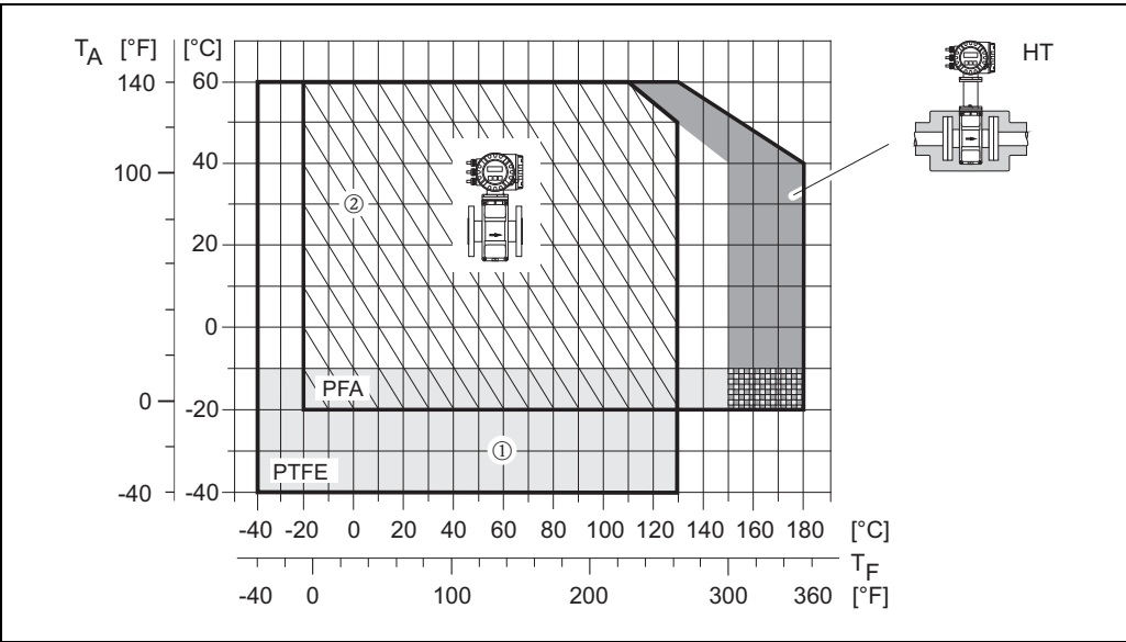
图 63：一体式 Promag P 传感器 (带 PFA 或 PTFE 内衬)
