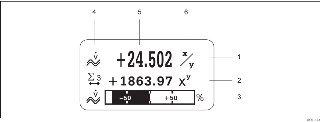
图 42: 正常操作模式下的典型显示界面 ( 主显示界面 )
