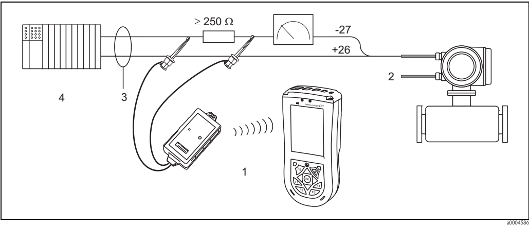
图 34: HART 手操器 Field Xpert SFX100 的电气连接示意图
