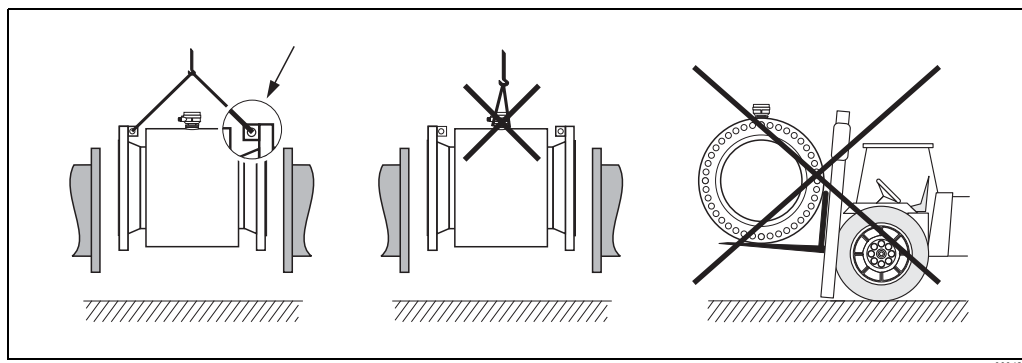
图 5: 传感器 (> DN 300 (12")) 的运输指南示意图
