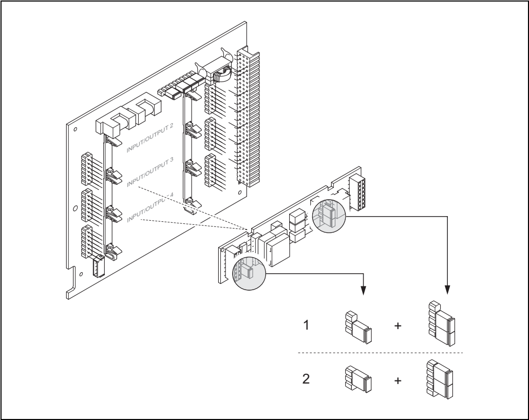
图 54: 通过跳线针 (I/O 板 ) 设置电流输入
