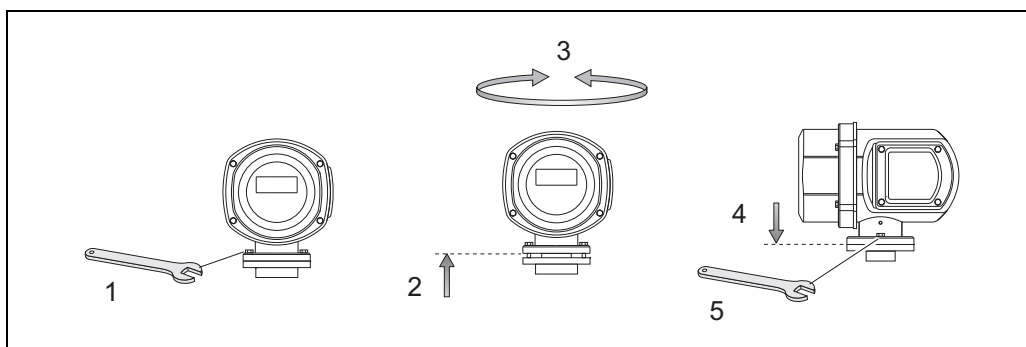
图 23: 旋转变送器外壳 (现场型不锈钢外壳)
