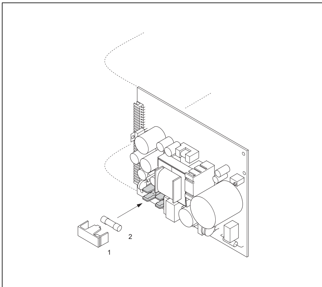
图 60: 更换电源板上的设备保险丝
