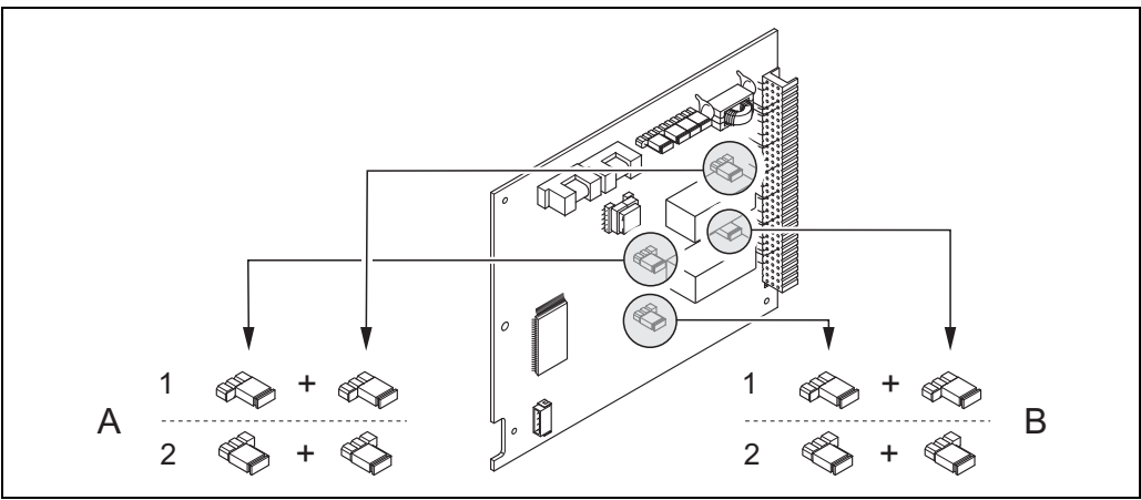
图 56: 固定 I/O 板上的继电器触点 (NC / NO) 设置
