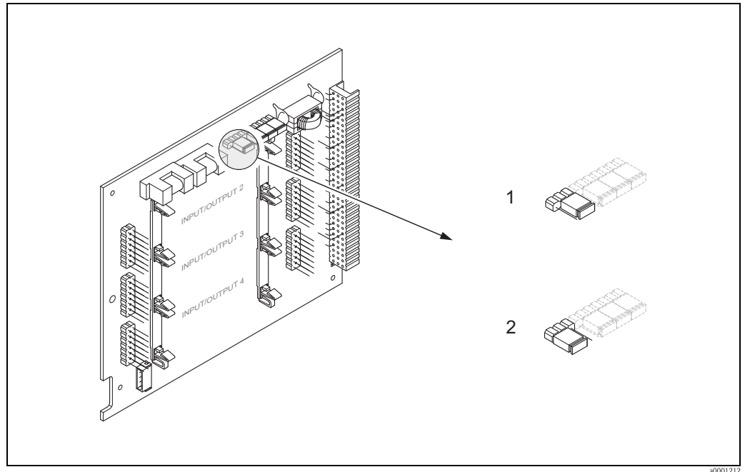
图 46: 切换 HART 写保护开 / 关
