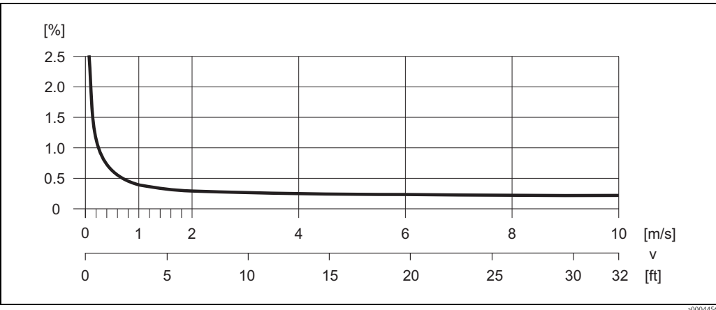
图 62: 最大测量误差 ( 读数值的 %) 示意图
