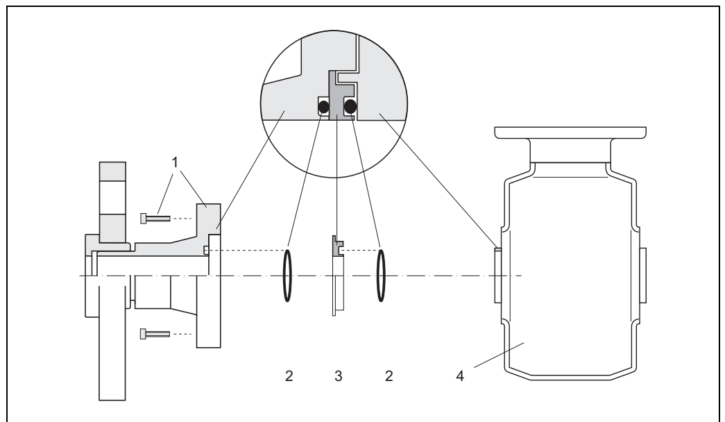
图 21: 在 Promag H 传感器内安装接地环 (DN 2...25 (1/12"...1"))
