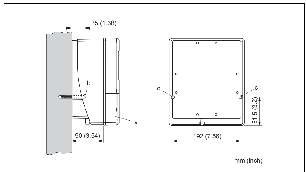
图 25: 直接安装在墙壁上
