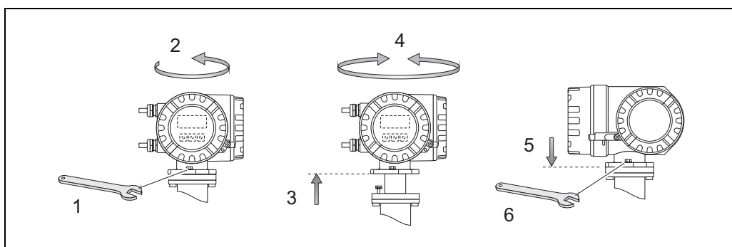
图 22: 旋转变送器外壳 (现场型铝外壳)
