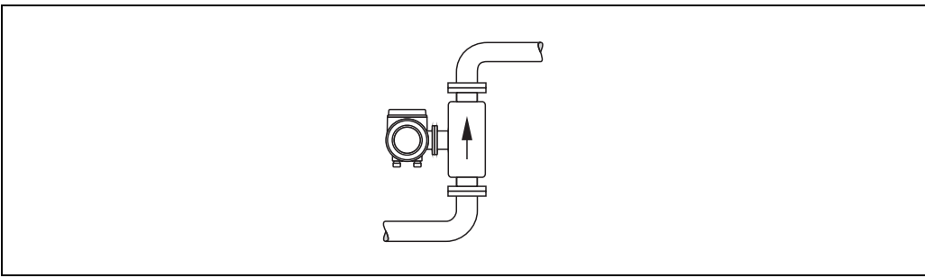
图 10: 竖直管道安装示意图
