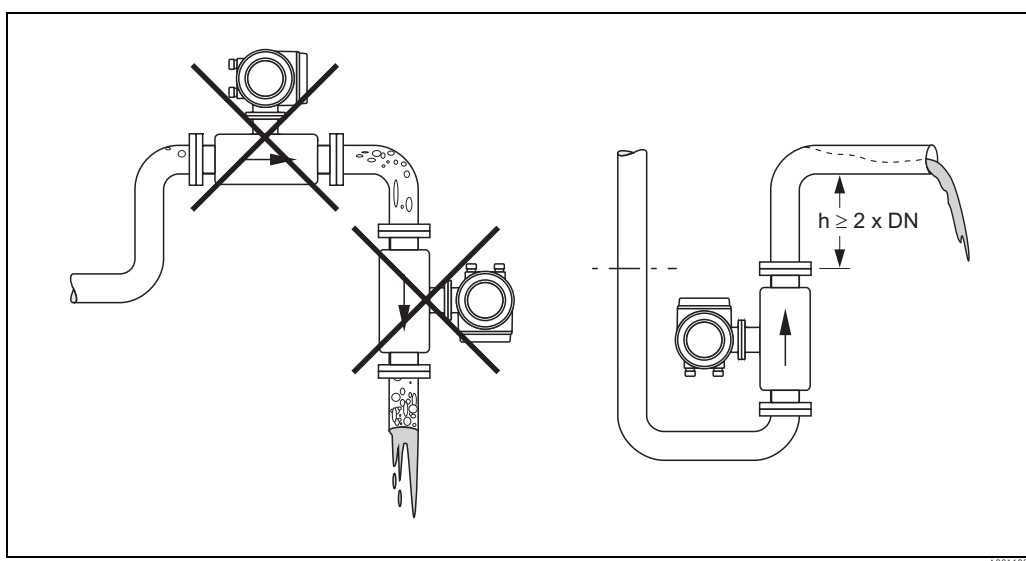
图 6: 安装位置示意图
