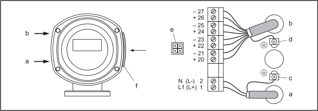
图 32: 变压器 ( 现场型不锈钢外壳 ) 的电气连接示意图，连接电缆的横截面积：max. 2.5 mm 2
