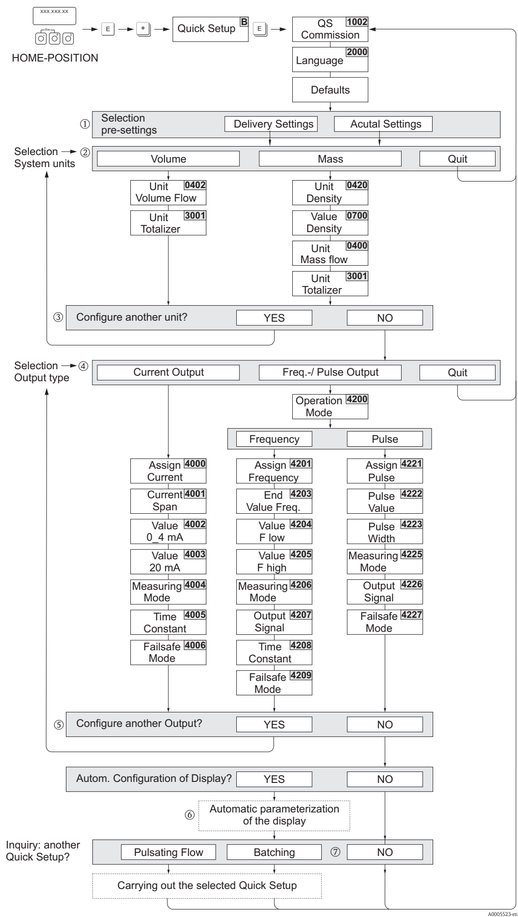
图 47: 快速设置直接进行仪表调试
