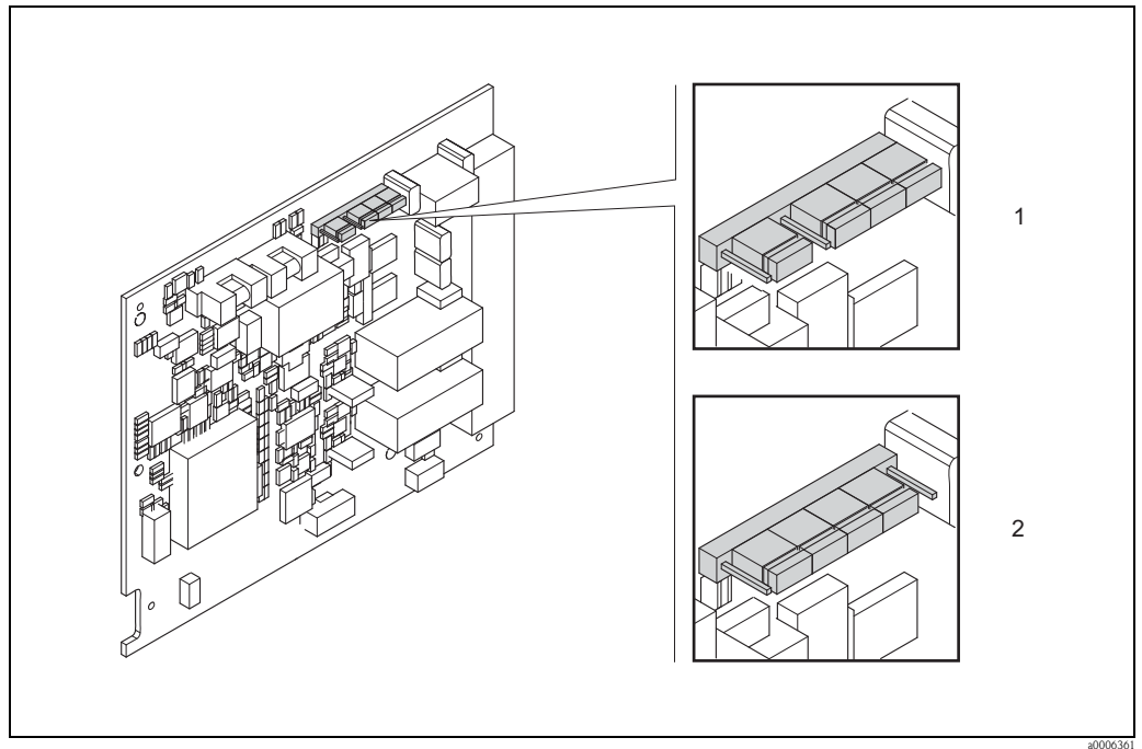
图 53: 通过跳线针 (固定 I/O 板) 设置电流输出
