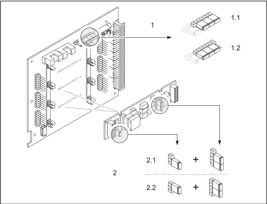
图 52: 通过跳线针 (可灵活设置 I/O 板) 设置电流输出
