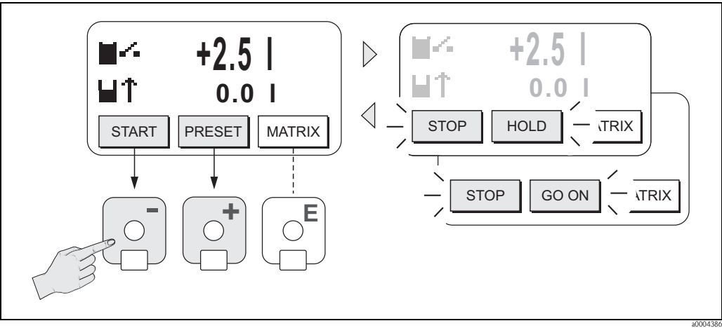
图 43: 通过现场显示 ( 功能按键 ) 控制批处理过程
