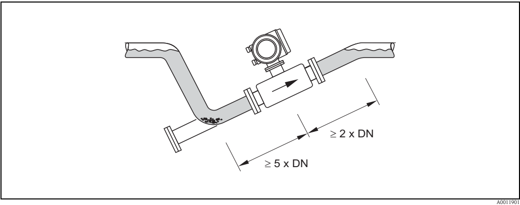
图 8: 在非满管管道中安装
