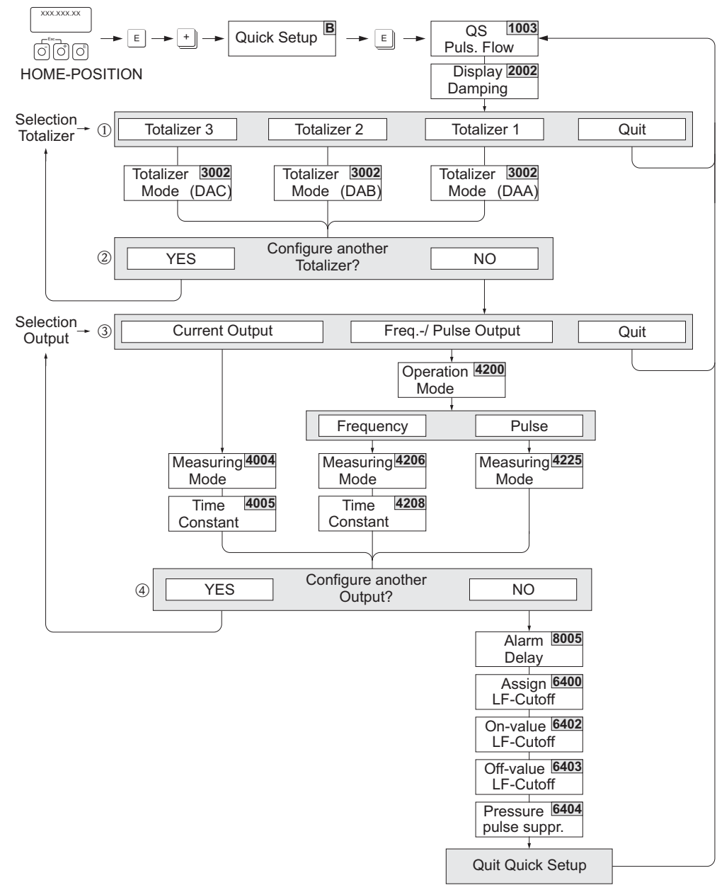
图 49: 剧烈脉动流的快速设置菜单。推荐设置如下。
