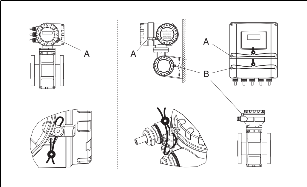
Promag 51 测量系统的标准权威机构铅封示意图
