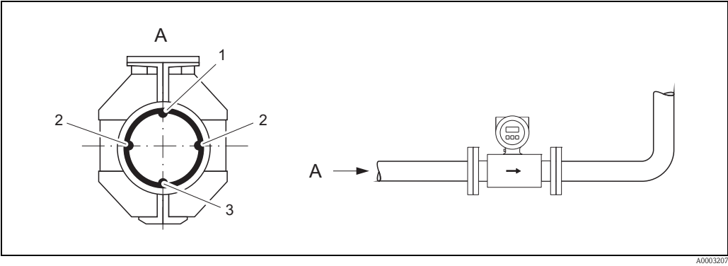
水平安装示意图
