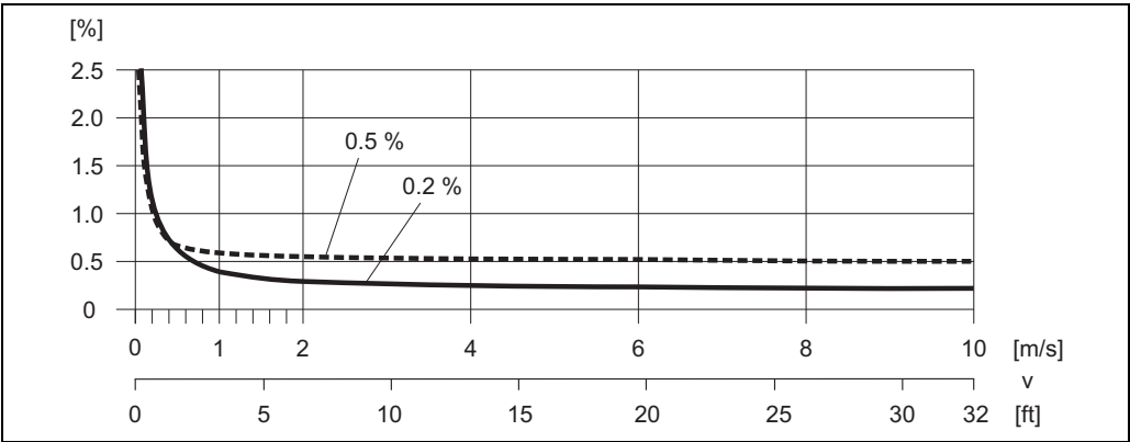
最大测量误差 ( 读数值的 %) 示意图
