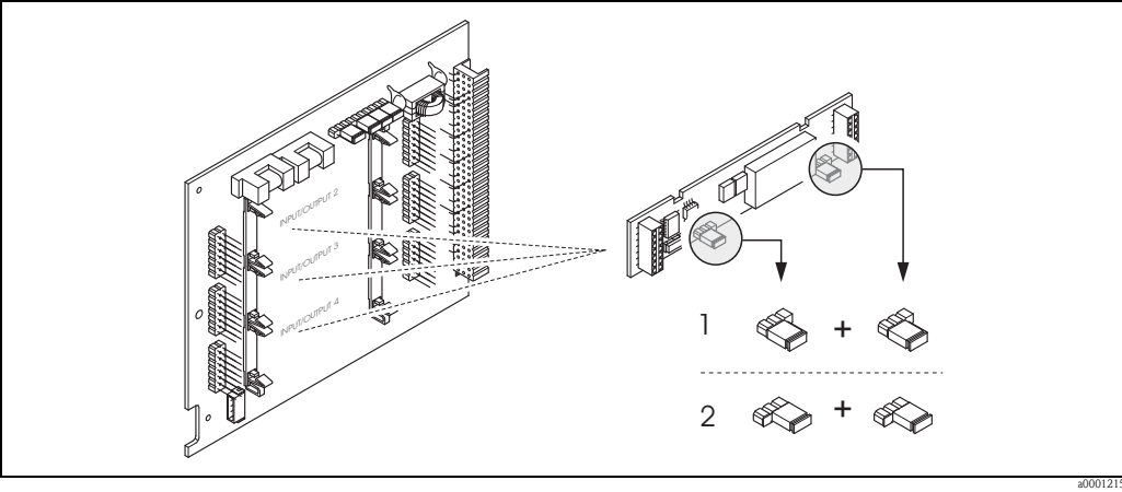
图 55: 可灵活设置 I/O 板 (子模块) 上的继电器触点 (NC / NO) 设置 )
