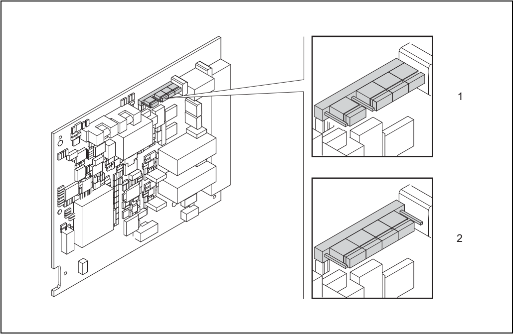
图 53: 通过跳线针 ( 固定 I/O 板 ) 设置电流输出
