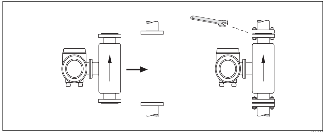
图 17: Promag W 传感器的安装示意图
