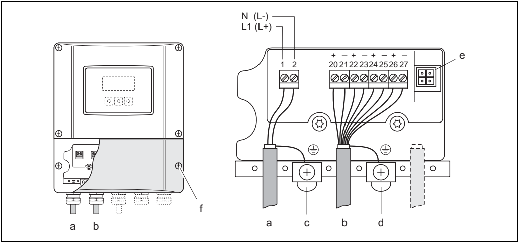
图 33: 变送器 ( 墙装型外壳 ) 的电气连接示意图, 连接电缆的横截面积: max. 2.5 mm 2
