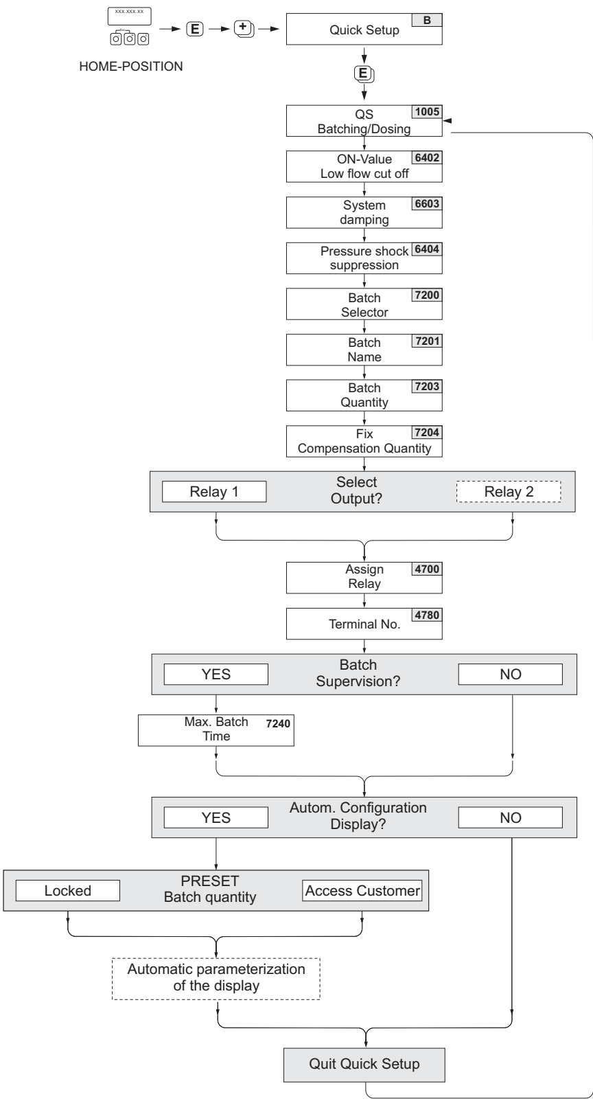
图 50: “Batching / 批处理”快速设置菜单。推荐设置请参考下表。
