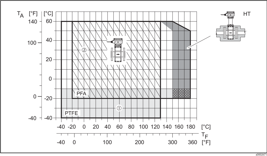
图 64: 分体式 Promag P 传感器 (带 PFA 或 PTFE 内衬) T_A = 环境温度; T_F = 流体温度; HT = 高温型仪表, 带保温层 ① = 灰色区域 → 温度范围: -10 \dots -40^\circ\text{C} ( -14 \dots -40^\circ\text{F} ), 适用于不锈钢法兰 ② = 斜线区域 → 泡沫内衬 (HE) + IP68 防护等级 = 流体温度: max. 130^\circ\text{C} ( 266^\circ\text{F} )
