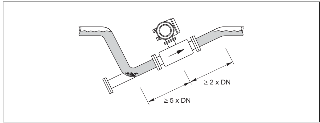
图 8: 在非满管管道中安装
