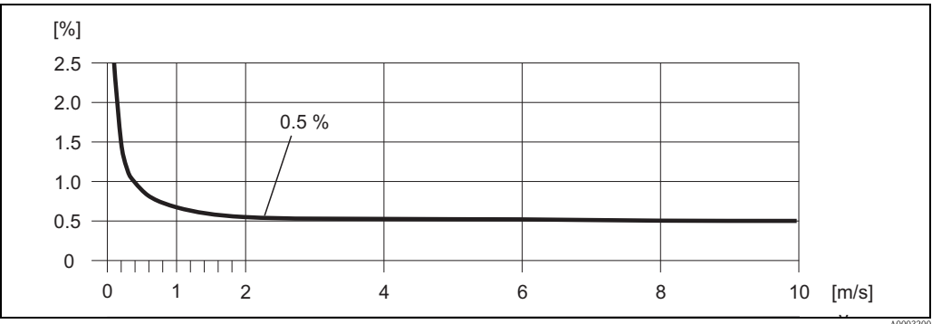
最大测量误差 ( 读数值的 %) 示意图
