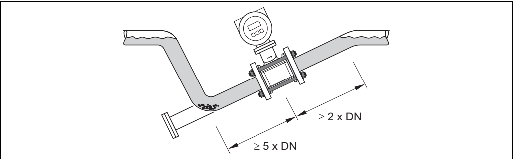
非满管道的安装示意图
