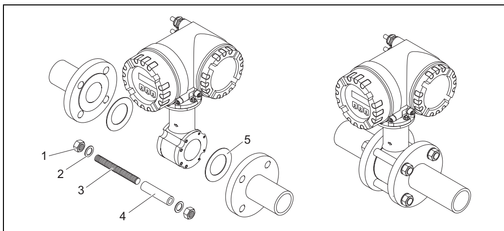
传感器的安装示意图
