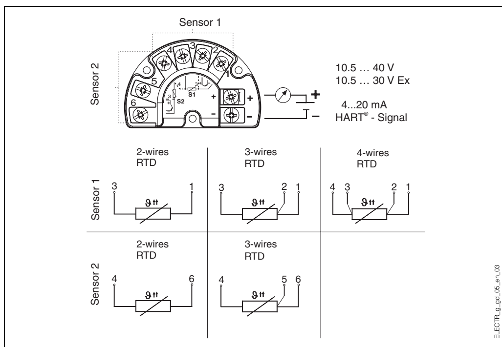
Fig. 2: Wiring diagram
