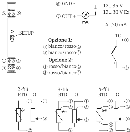
3: Disposizione dei morsetti
