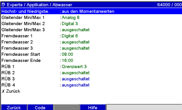
Abb. 3: Setup - Applikation - Abwasser
