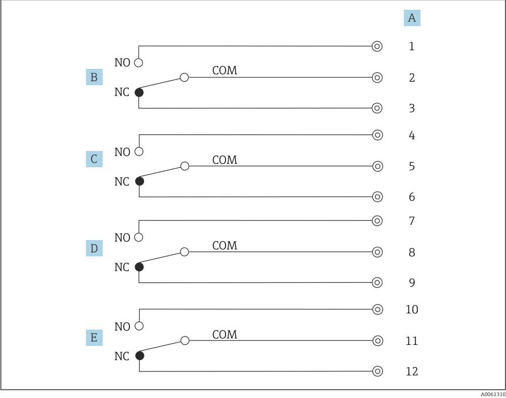
15 Wiring diagram
