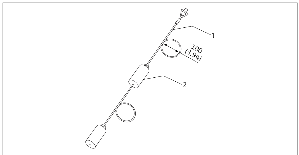
5 Displacer unit
