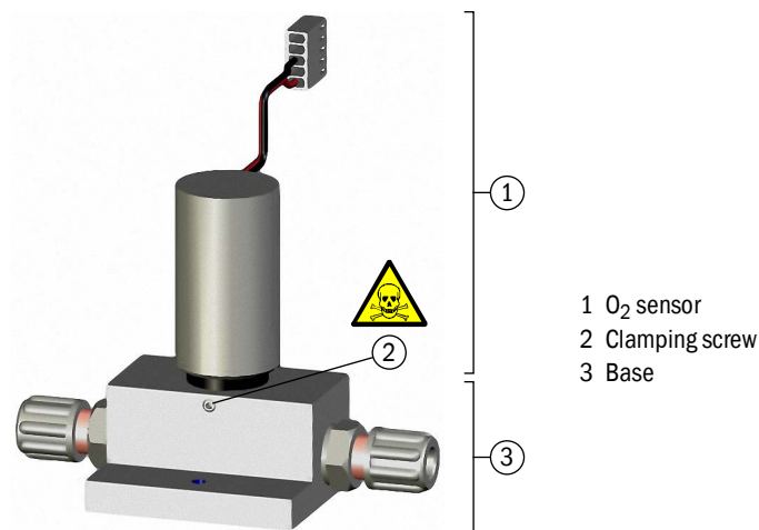
Fig. 32: Analyzer module OXOR-E
