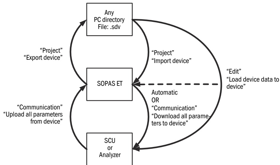
Fig. 12 Loading parameters
