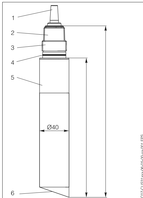
Fig. 3: CUS 31 dimensions
