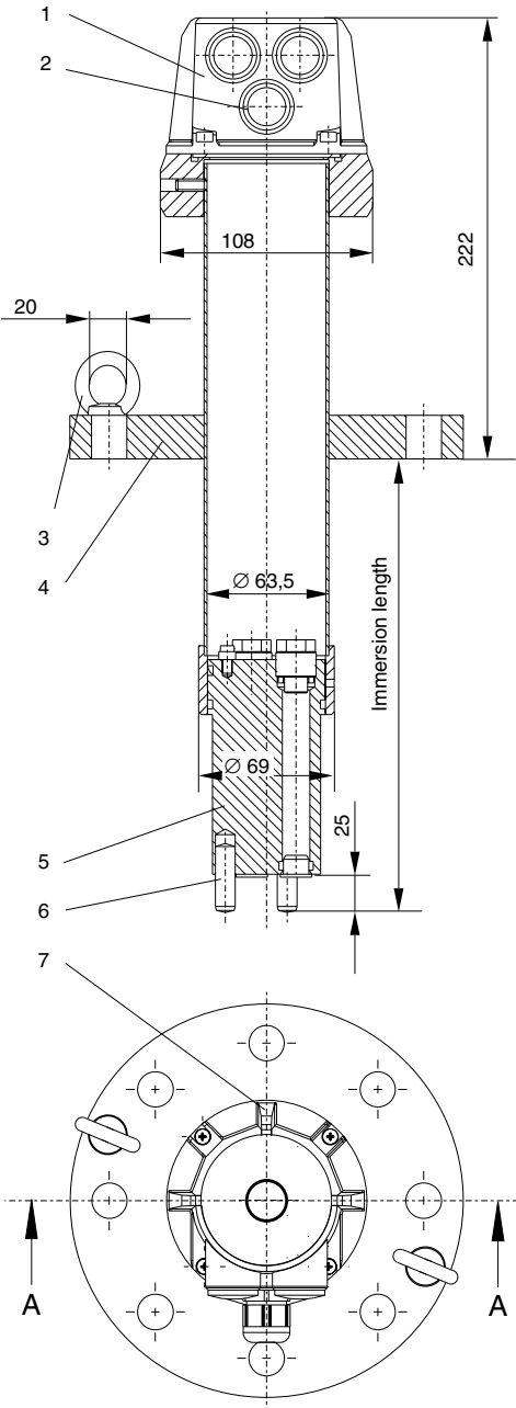
Section A-A
