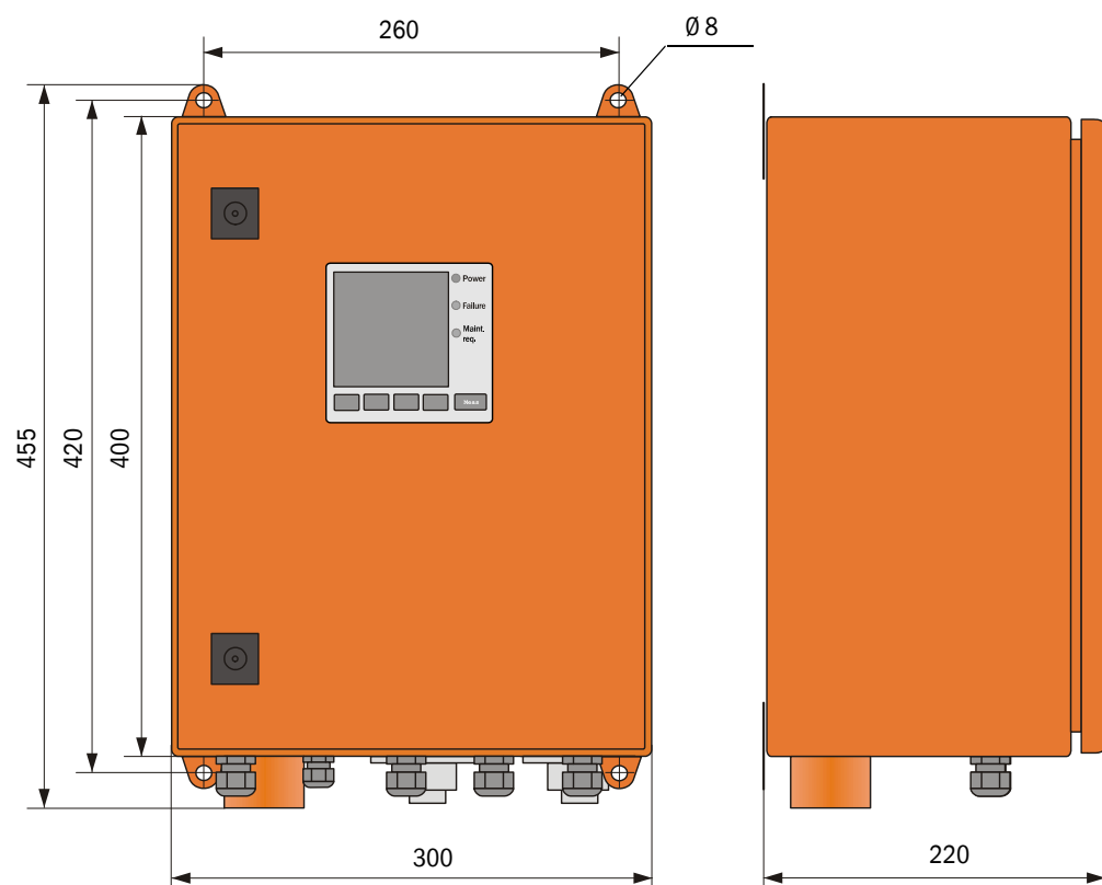
Bild 31 Steuereinheit MCU-P
