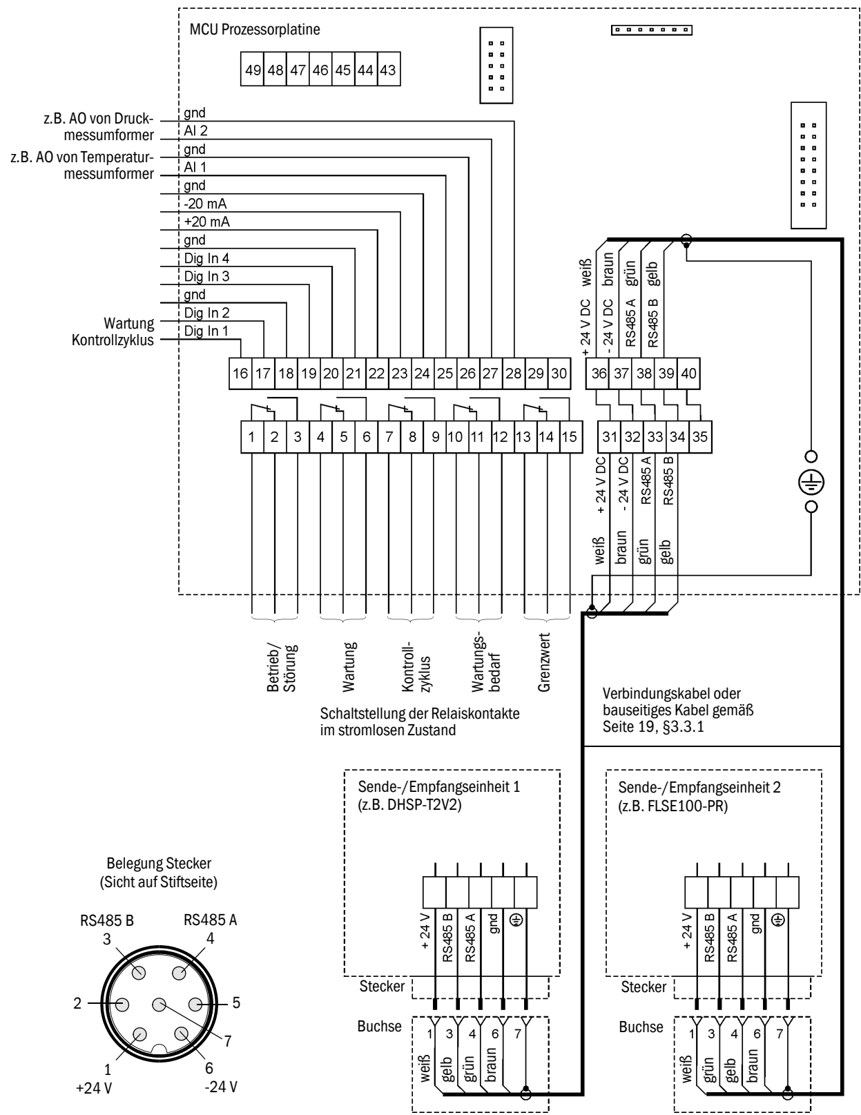
Bild 8 Anschluss der Sende-/Empfangseinheiten
