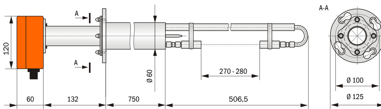
Bild 26 Sende-/Empfangseinheit FLSE100-PR
