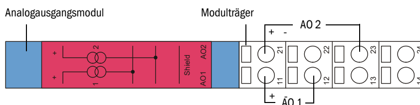
Anschlussbelegung Analogausgangsmodul
