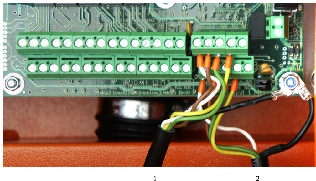
Anschluss der Sende-/Empfangseinheiten
