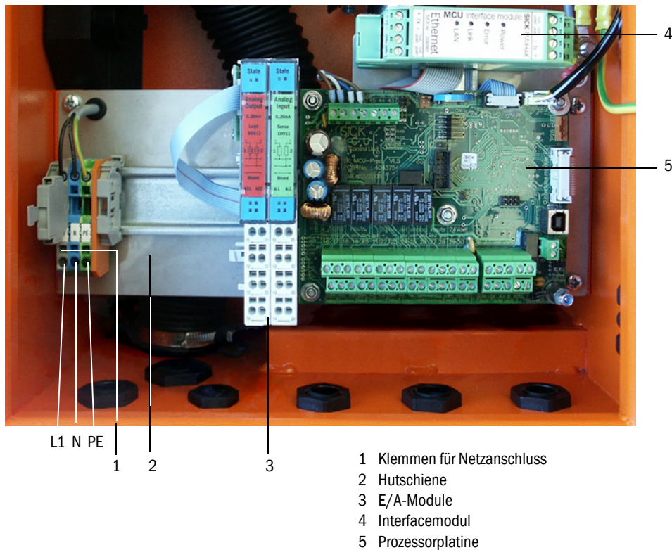
Bild 5 Innenansicht MCU
