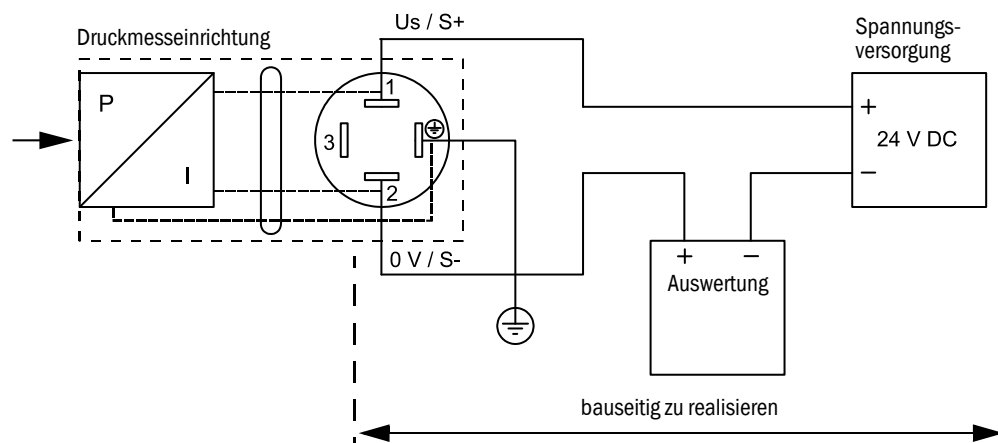
Anschluss Druckmessumformer
