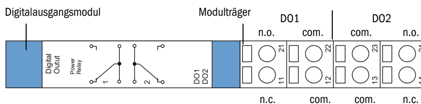
Anschlussbelegung Digitalausgangsmodul Power Relay
