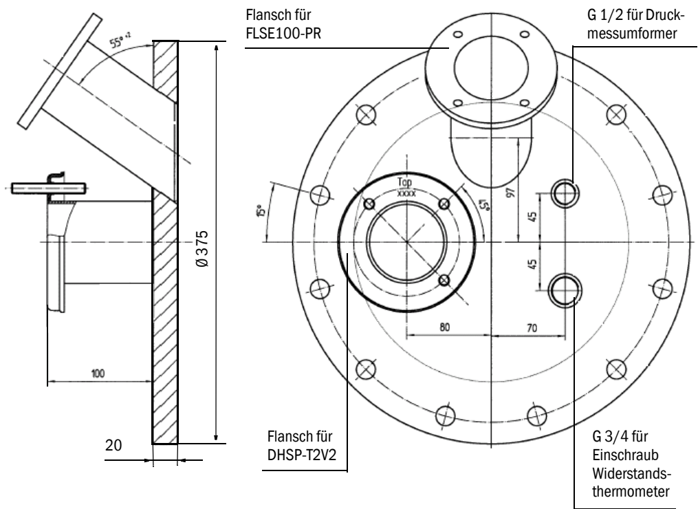
Bild 29 Kombiflansch k335 DN250
