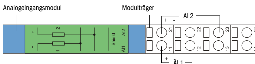
Anschlussbelegung Analogeingangsmodul
