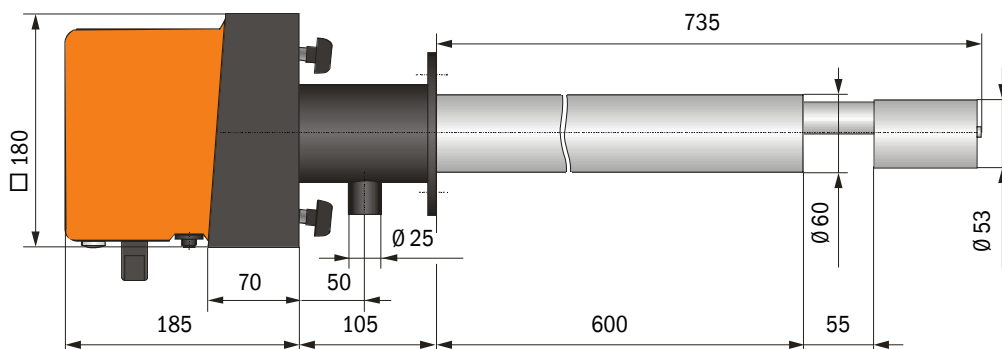
Bild 25 Sende-/Empfangseinheit DHSP-T2V2
