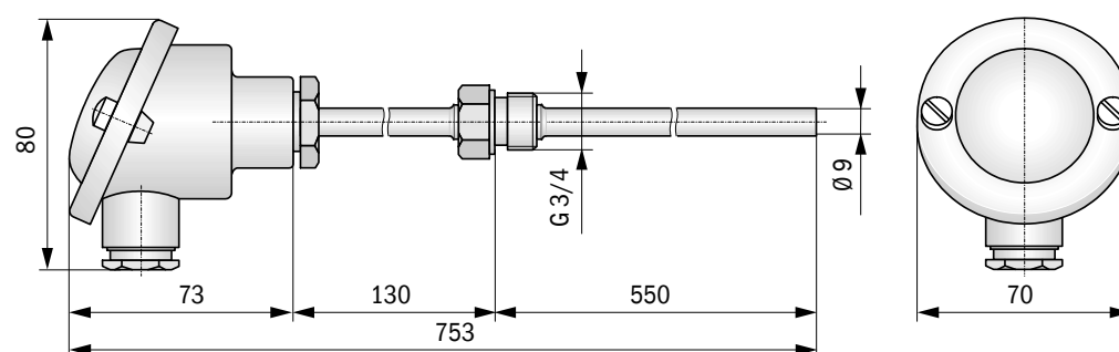
Bild 28 Einschraub-Widerstandsthermometer
