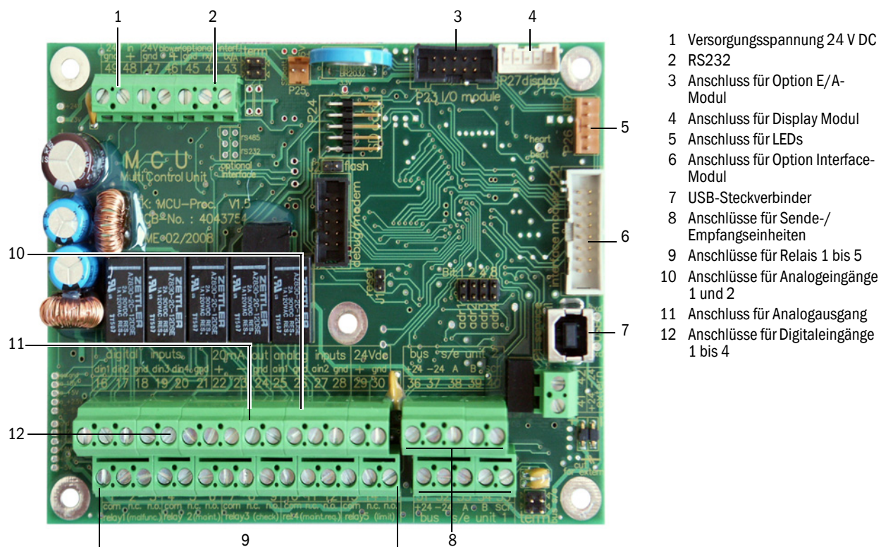
Anschlüsse der MCU-Prozessorplatine
