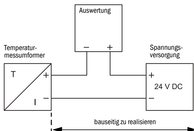
Anschluss Temperaturmessumformer
