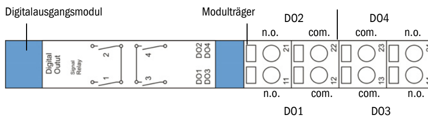
Anschlussbelegung Digitalausgangsmodul Signal Relay (4 Schließer)
