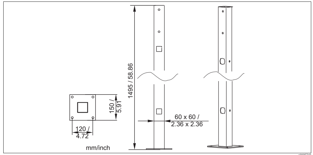
Fig. 48: Universal post
