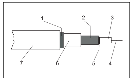
Fig. 24: CYK71 cable
